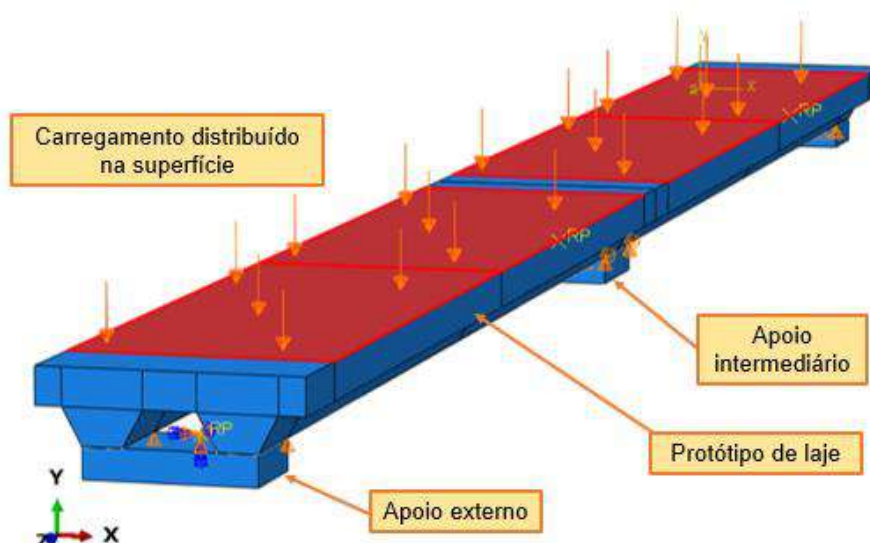
Figura 133 – Modelo de cálculo: calibração parâmetros termomecânicos (modelo 3a)
