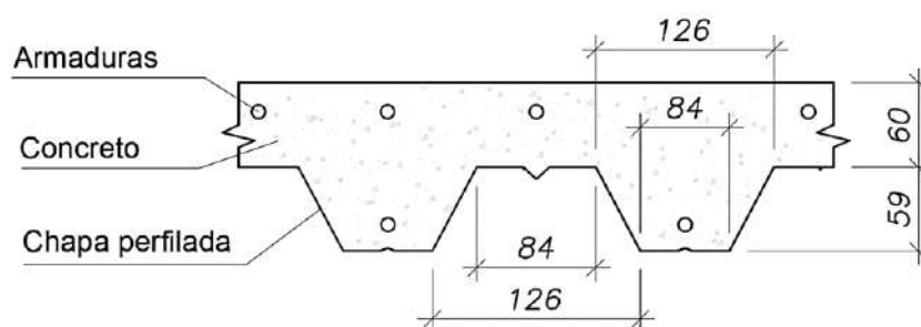
Figura 41 – Características da seção das lajes experimentais (valores em mm)
