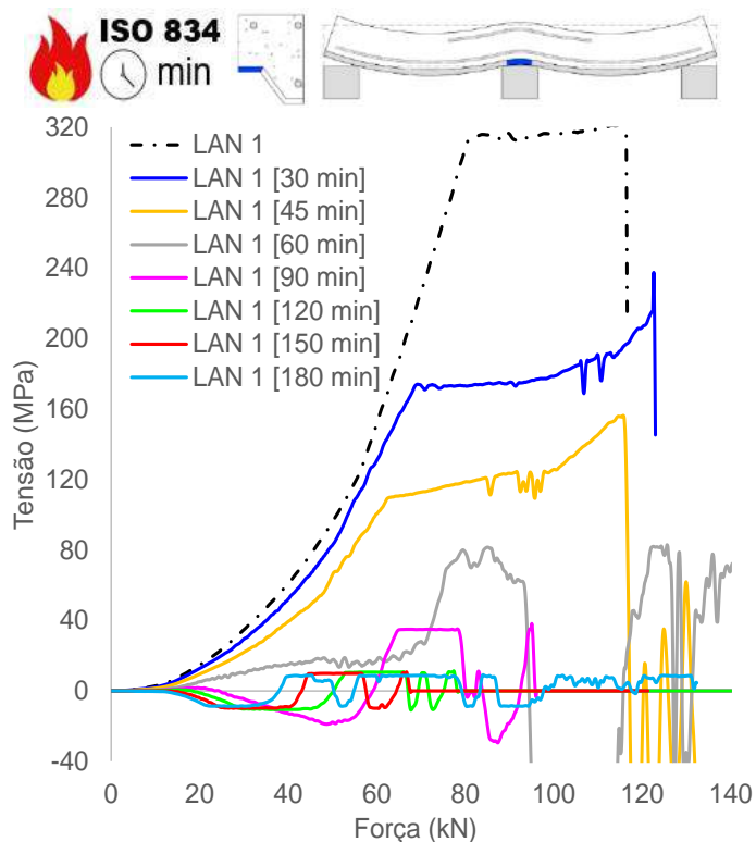
(e) Tensão chapa, mesa superior (apoio)
