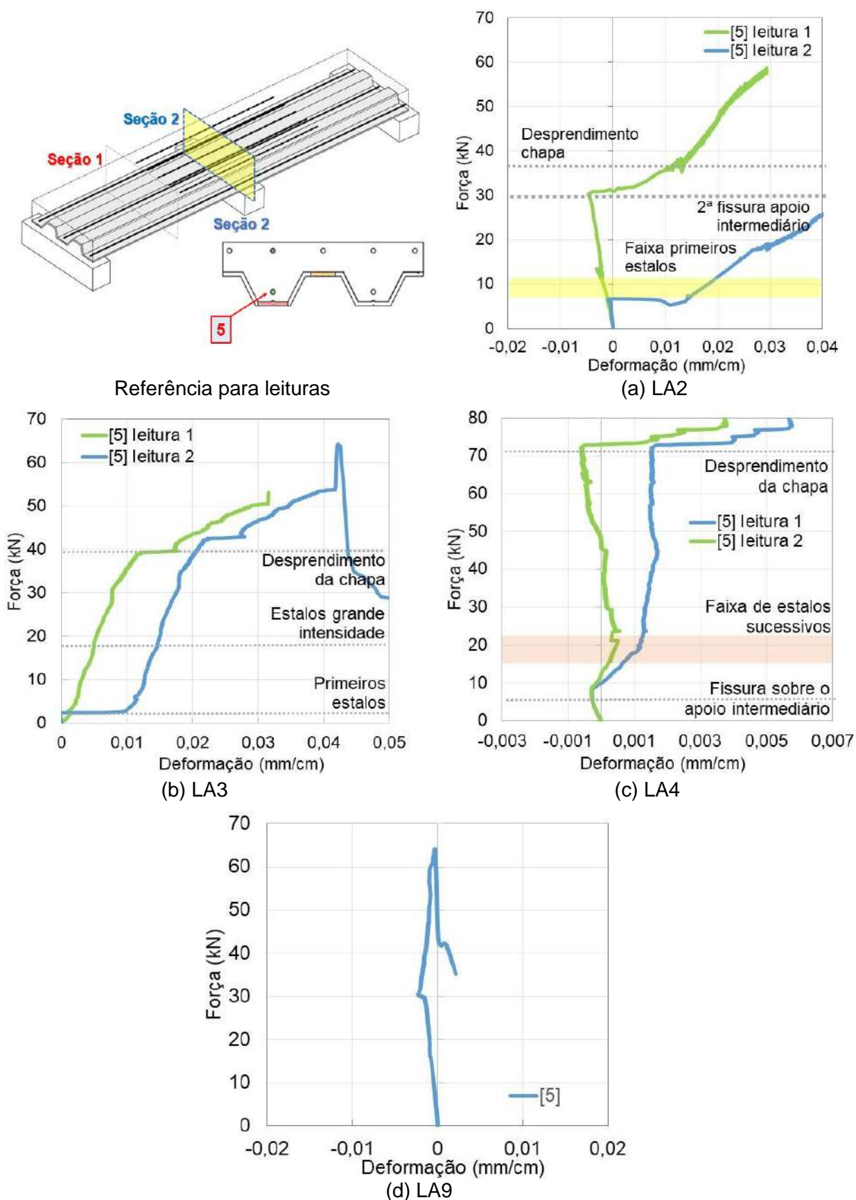
Figura 68 – Alongamento da armadura positiva junto ao apoio intermediário
