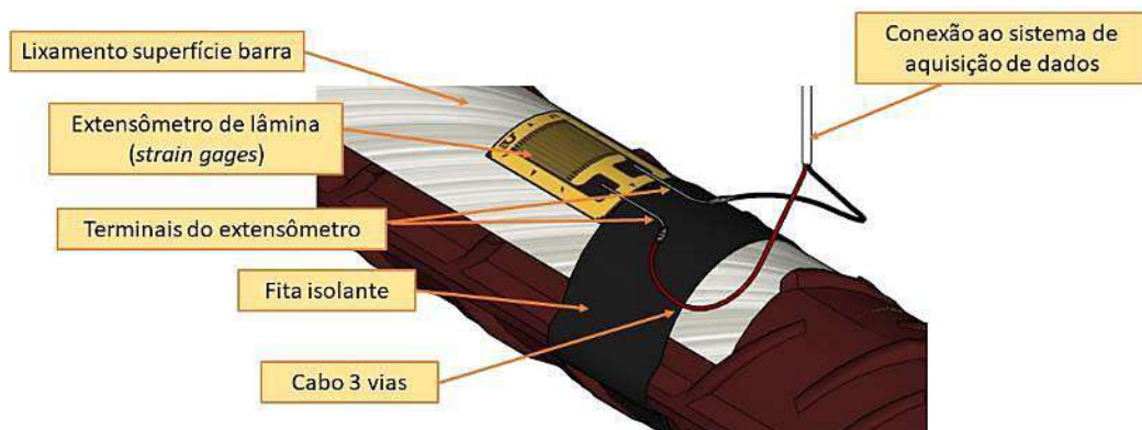
Figura 55 – Detalhe da instalação do extensômetro de lâmina
