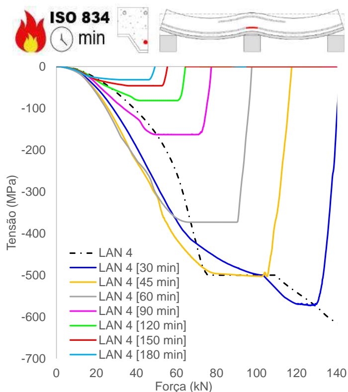
(d) Tensão armaduras positivas (apoio)
