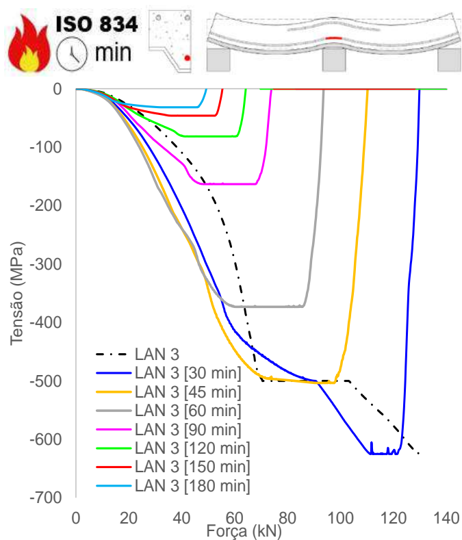
(d) Tensão armaduras positivas (apoio)
