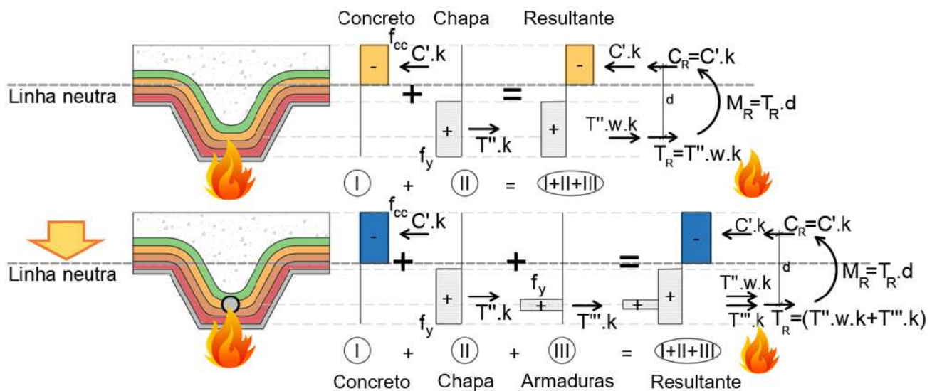
Figura 170 – Deslocamento linha neutra e armaduras positivas (meio do vão)
