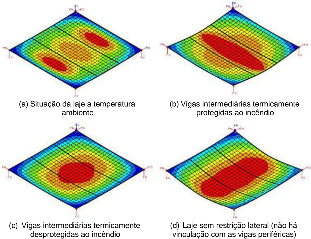
Figura 35 – Efeito da proteção térmica das vigas e vinculação das lajes Fonte: adaptado de Gernay e Khorasani (2020)
