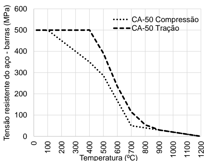
Figura 118 – Tensão resistente do aço CA-50: modelo numérico
