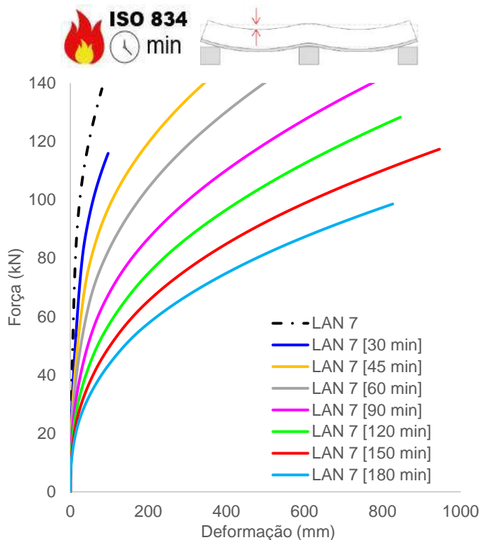
(a) Deformações verticais (flechas)
