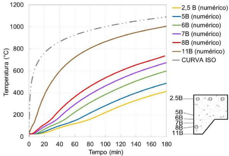
Figura 165 – Modelo numérico: temperaturas no concreto (linha B da seção)
