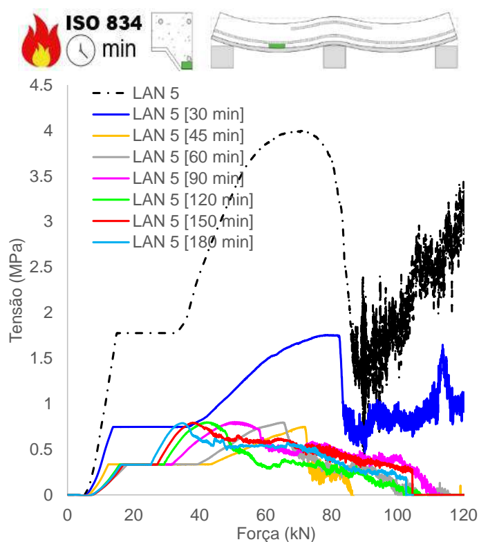
(j) Tensão concreto, adjacência mesa inferior chapa (vão)
