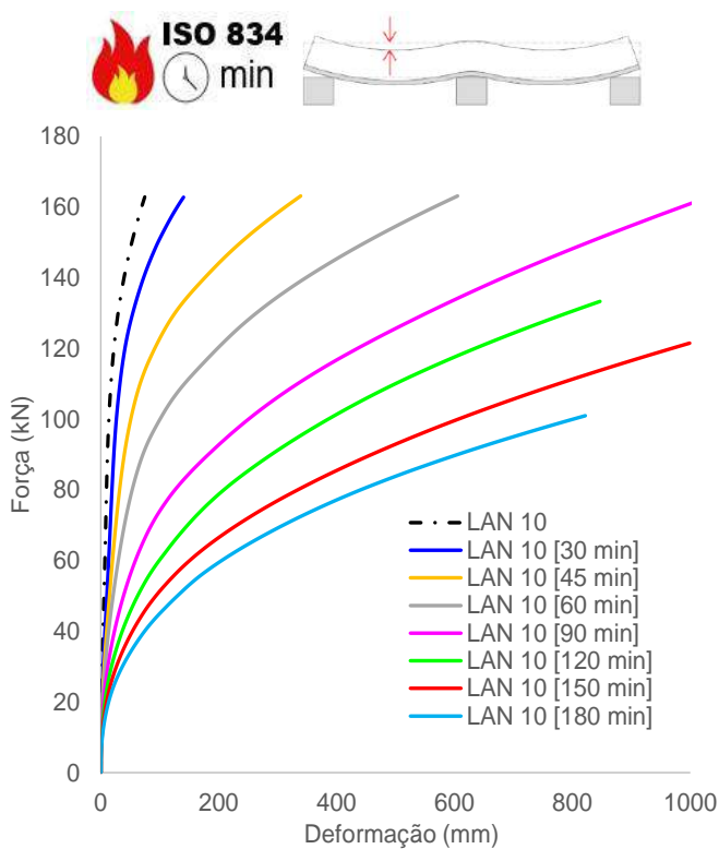
(a) Deformações verticais (flechas)
