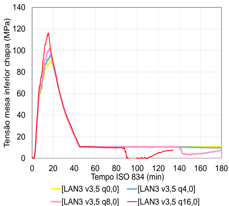
Figura 187 – Tensões produzidas na chapa perfilada (Ch.1): vão 3,5 m
