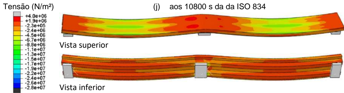
Figura 178 –Tensões na LAN3 ao longo da exposição ao incêndio padrão
