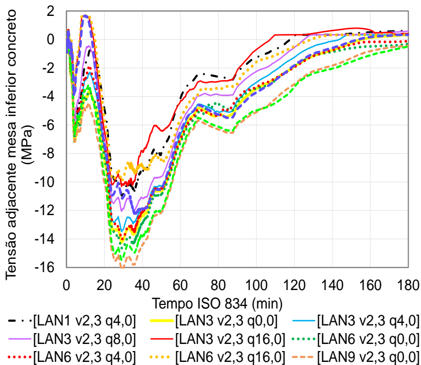
Figura 188 – Tensões produzidas no concreto, meio do vão (Co.1): vão 2,3 m
