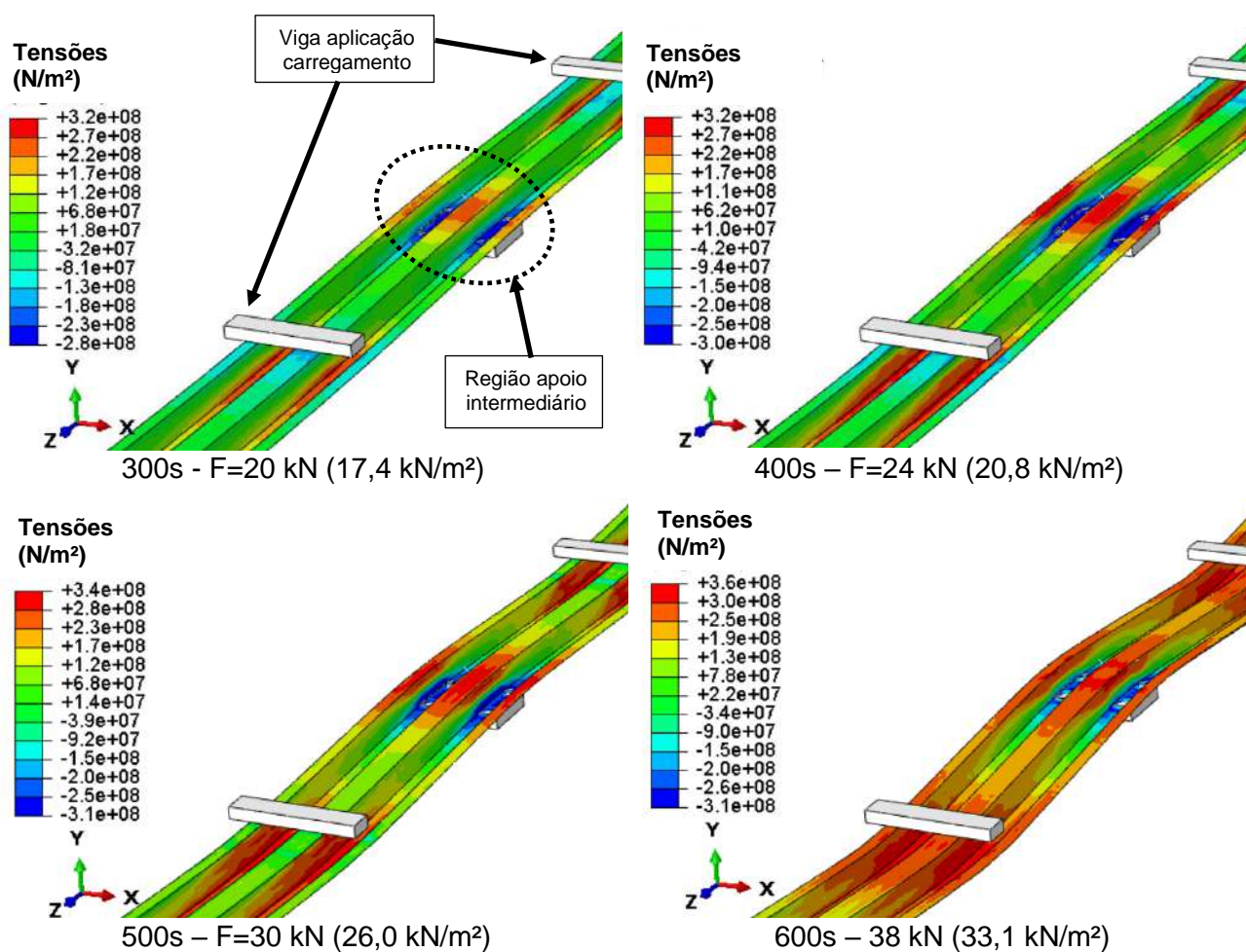
Figura 144 – Tensões na chapa na região apoio intermediário
