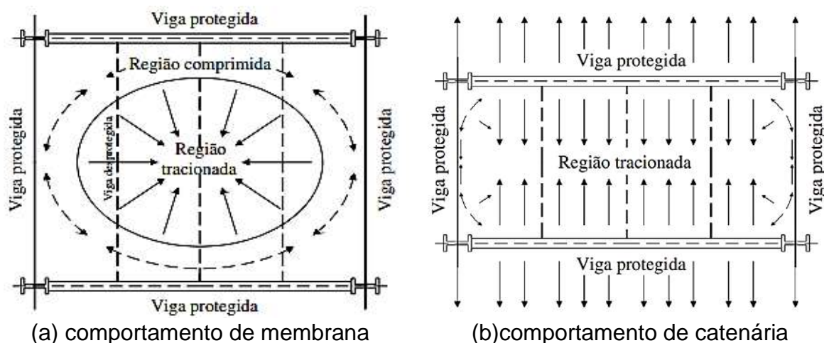
Figura 24 – Comportamento de membrana e catenária de lajes mistas
