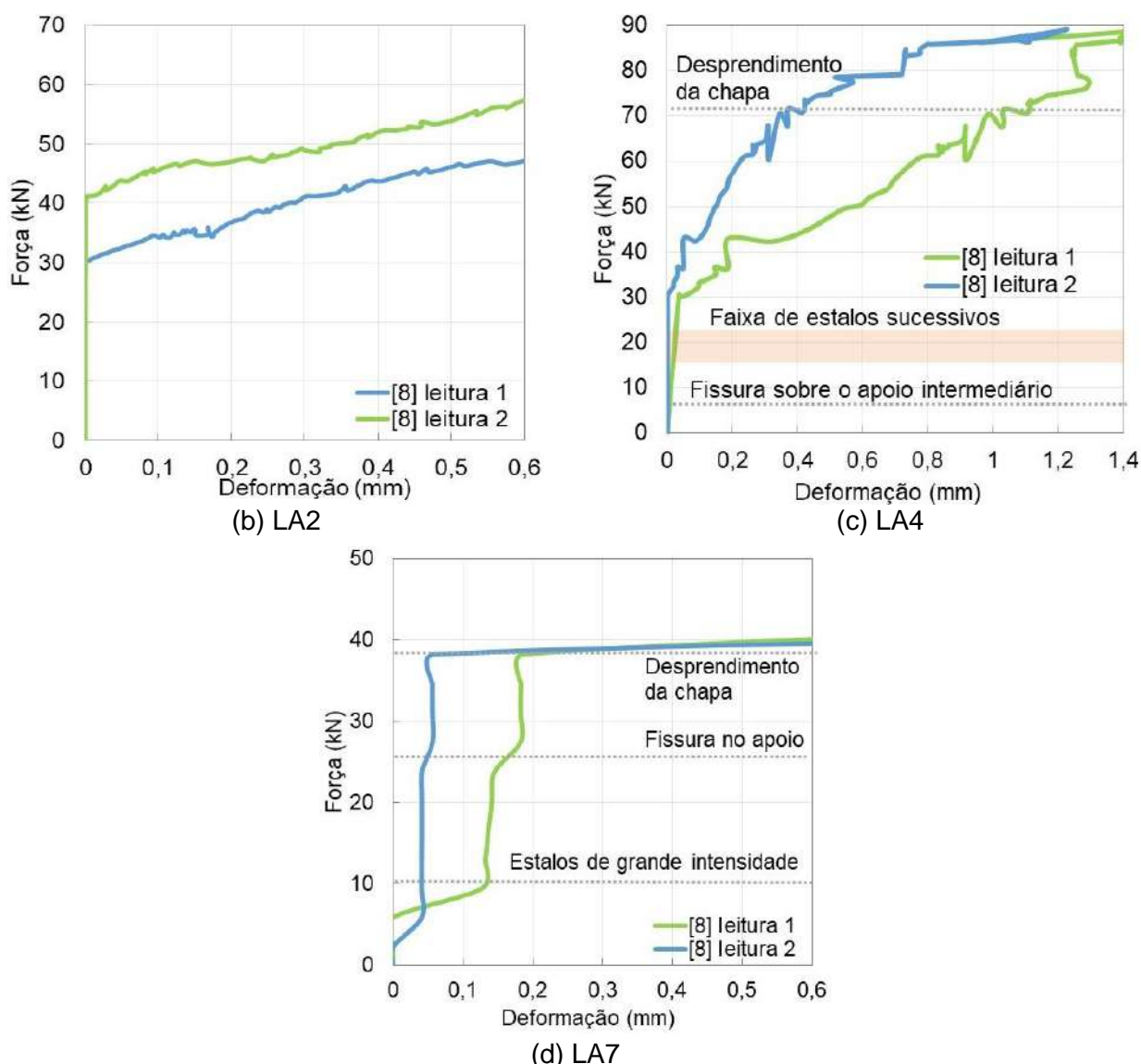
Figura 73 – Escorregamento relativo chapa-concreto
