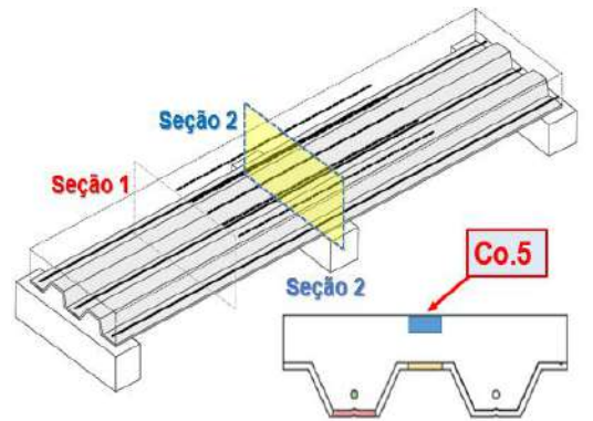
Figura 194 – Tensões no concreto, apoio intermediário (Co.5): vão 2,3 m
