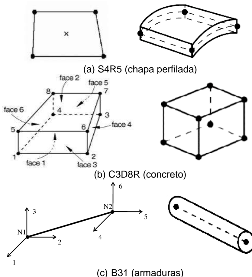
Figura 96 – Elementos finitos adotados no modelo numérico
