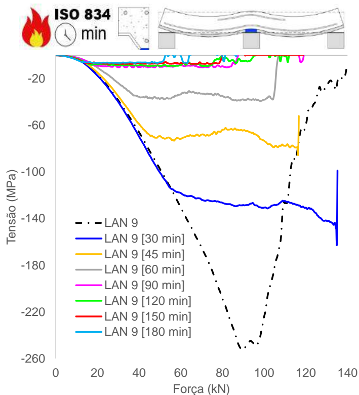
(h) Tensão chapa, mesa inferior (apoio)
