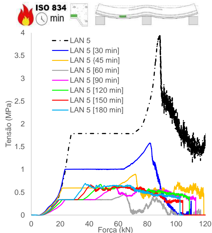
(k) Tensão concreto, adjacência mesa superior chapa (vão)
