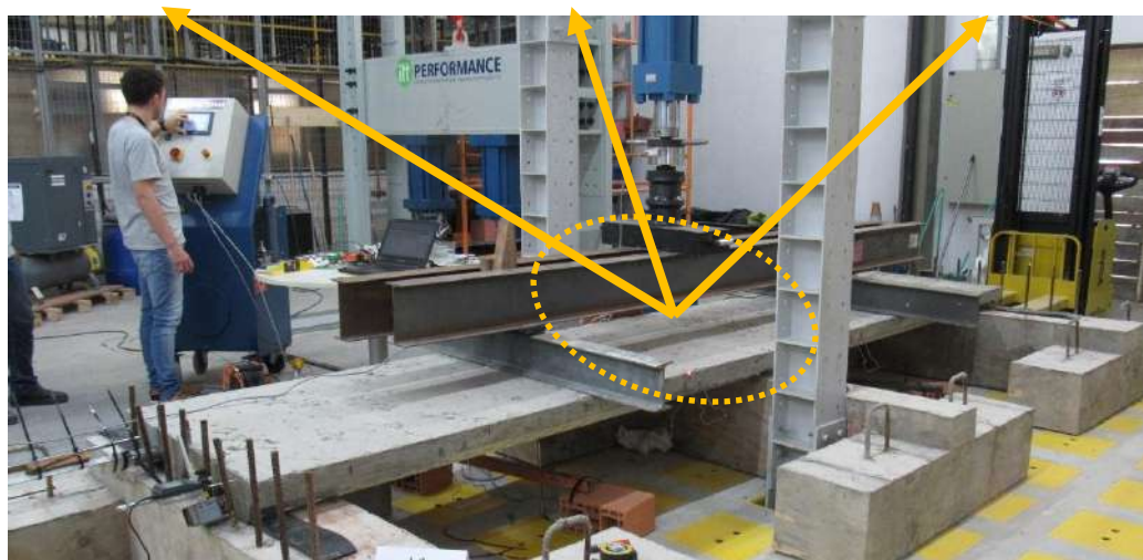
Figura 67 – Manifestações na região do apoio intermediário
