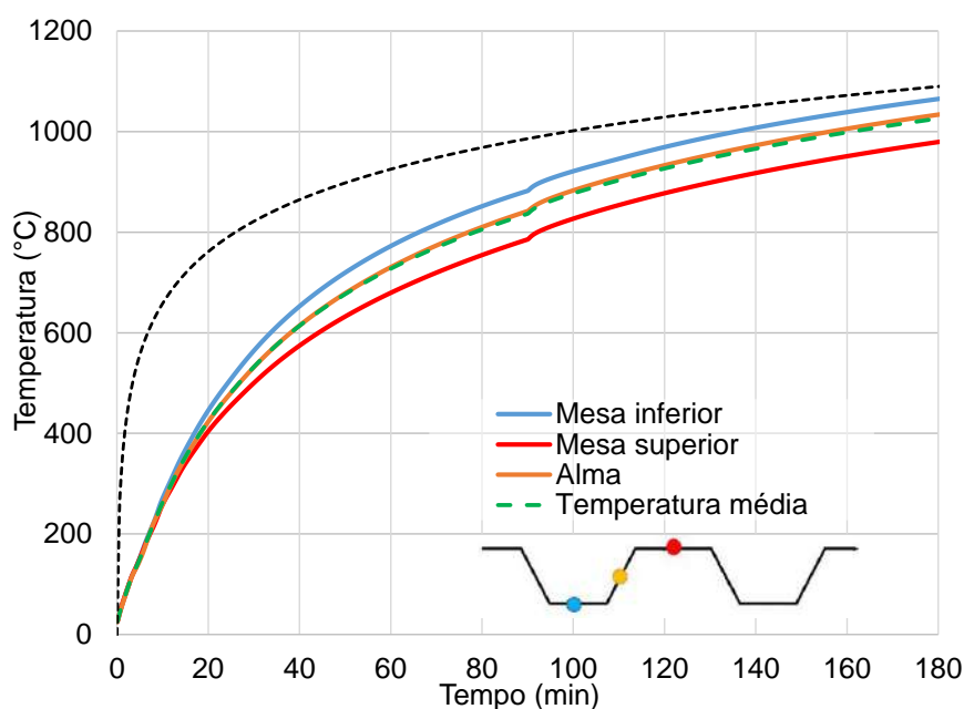
Figura 163 – Modelo numérico: curvas de temperatura na chapa
