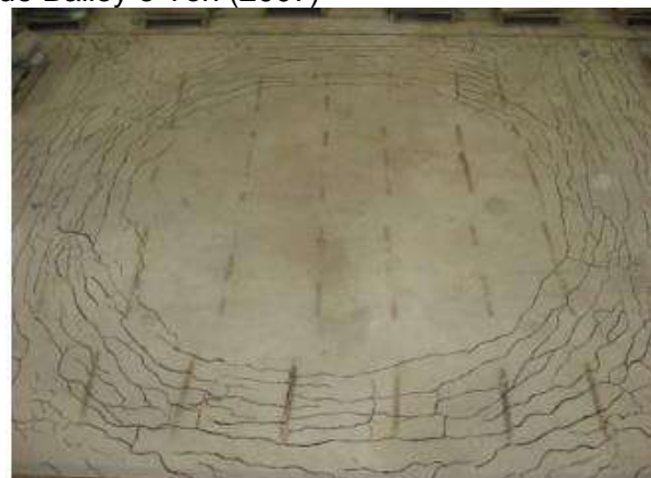
(b) Fissuras na superfície da laje
