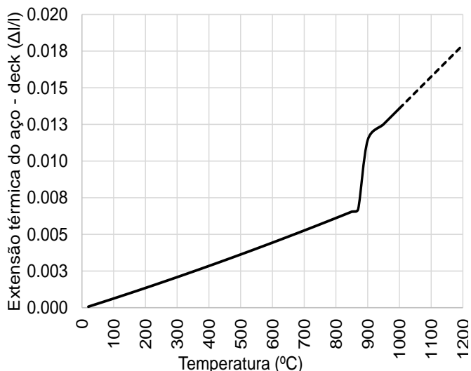
Figura 126 – Extensão térmica do aço da chapa: modelo numérico
