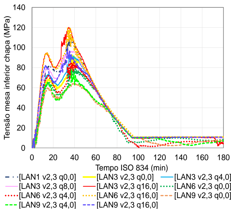
Figura 186 – Tensões produzidas na chapa perfilada (Ch.1): vão 2,3 m
