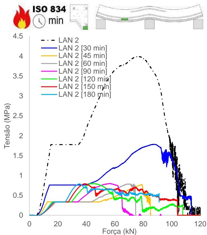
(l) Tensão concreto, adjacência mesa inferior chapa (vão)
