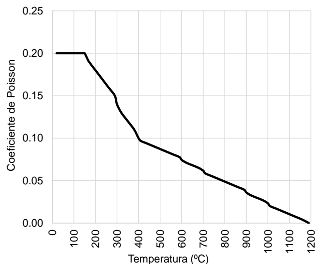
Figura 113 – Coeficiente de Poisson do concreto: modelo numérico
