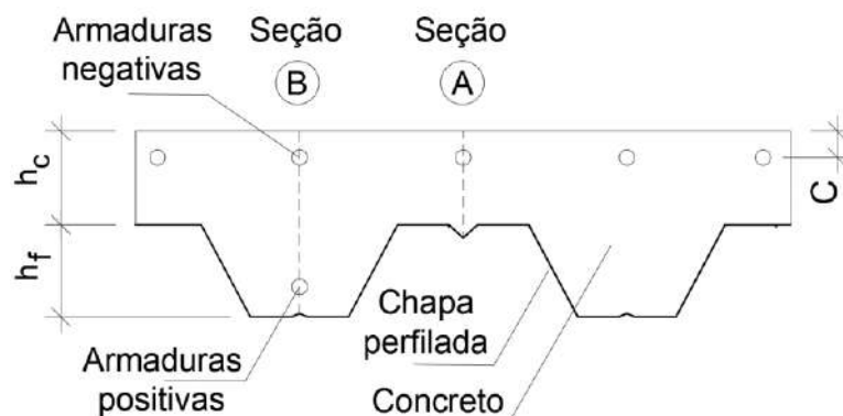
Figura 137 – Características geométricas da seção admitida no comparativo
