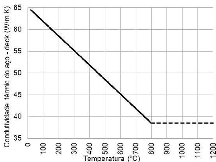
Figura 107 – Condutividade térmica do aço da chapa: modelo numérico
