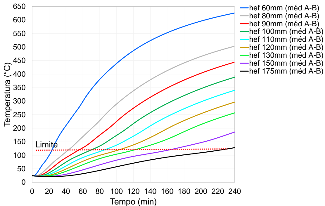
Figura 218 – Isolamento térmico: temperaturas médias (ponto A e B)
