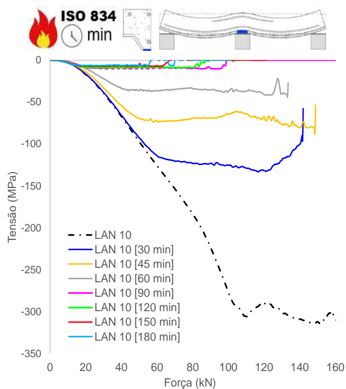
(h) Tensão chapa, mesa inferior (apoio)
