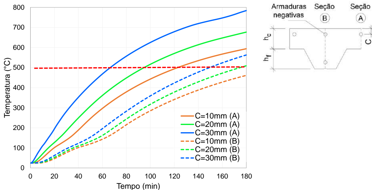
Figura 210 – Temperatura nas armaduras negativas, h_c=40\text{mm} e h_f=59\text{mm}
