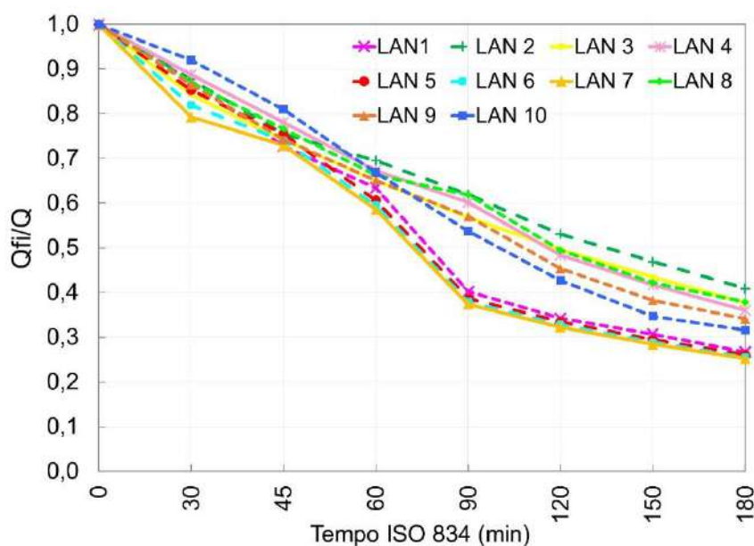
Figura 167 – Redução da resistência por laje para diferentes tempos da ISO 834
