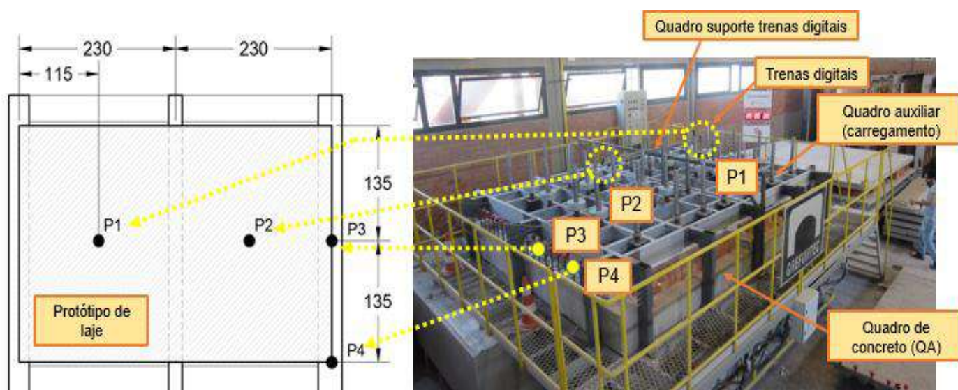
Figura 58 – Pontos de medição das deformações verticais
