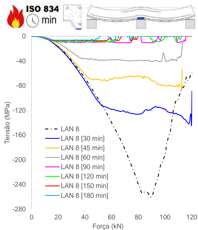
(h) Tensão chapa, mesa inferior (apoio)
