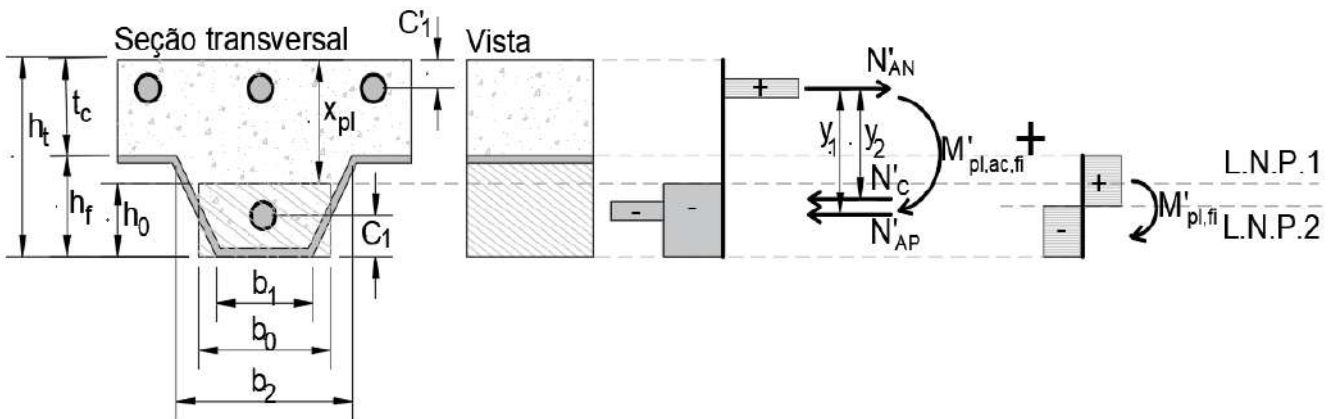
Figura 203 – Momento resistente negativo: armaduras positivas e negativas (II)
