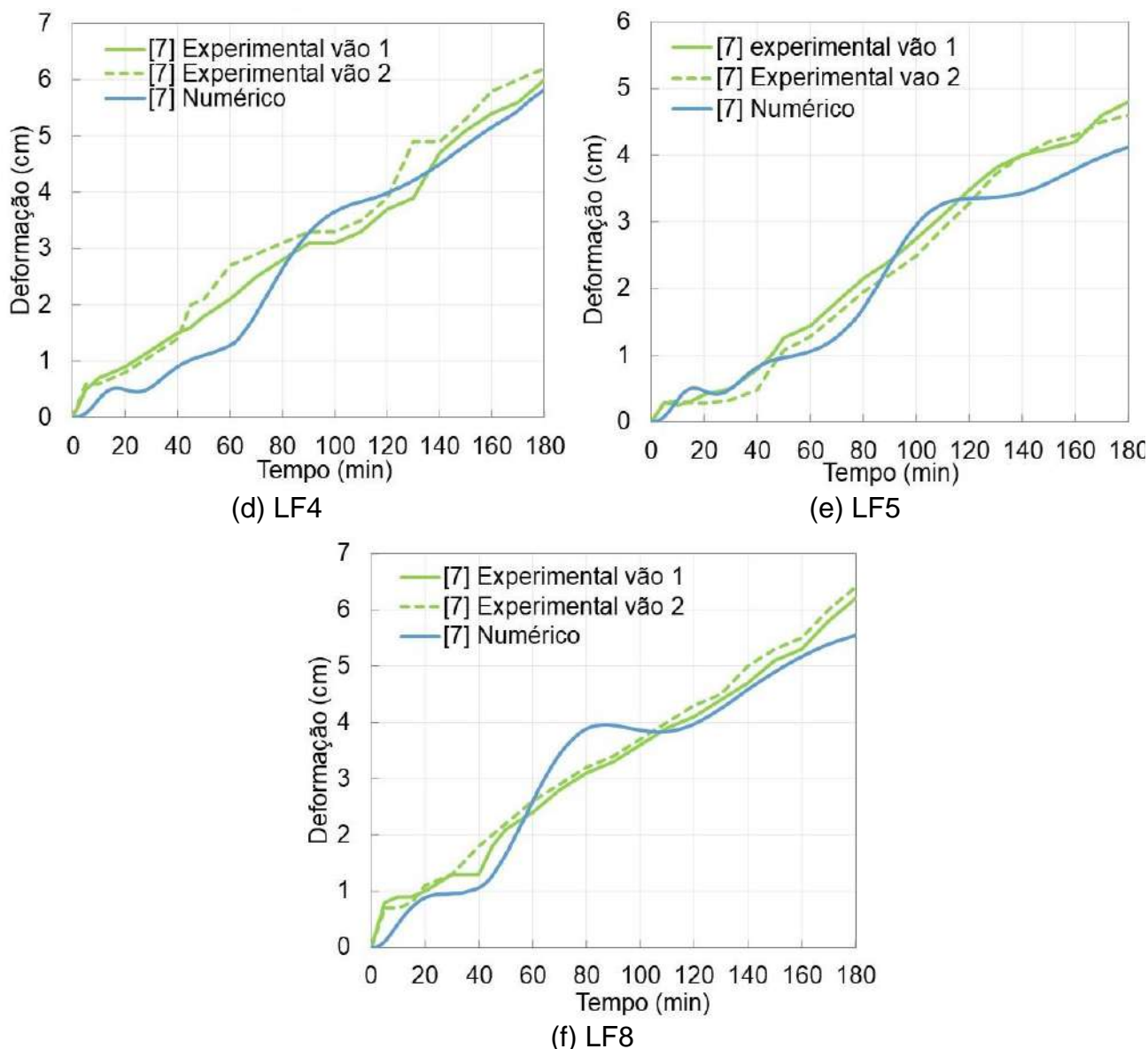
Figura 154 – Calibração da deformação vertical (flecha)
