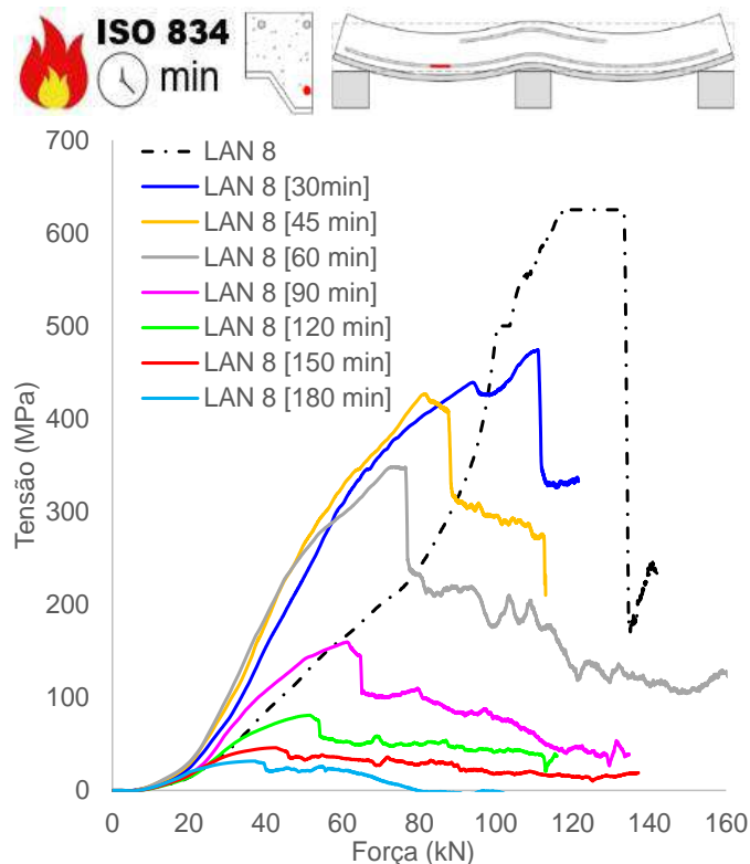
(b) Tensão armaduras positivas (vão)
