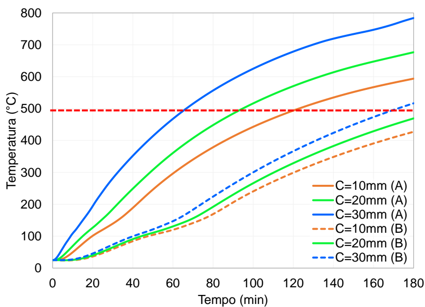
Figura 214 – Temperatura nas armaduras negativas, h_c=40\text{mm} e h_f=75\text{mm}
