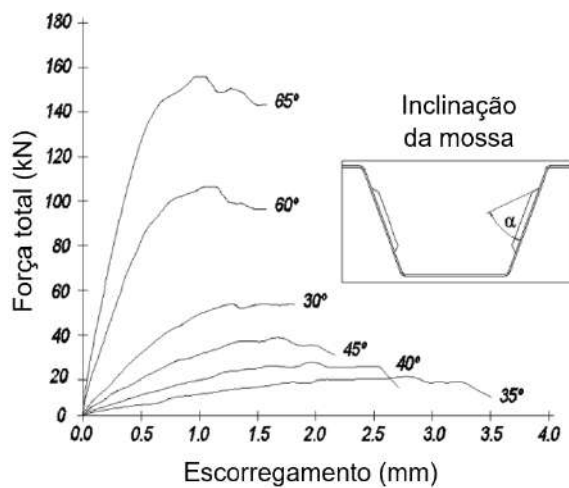
(a) inclinação da mocha
