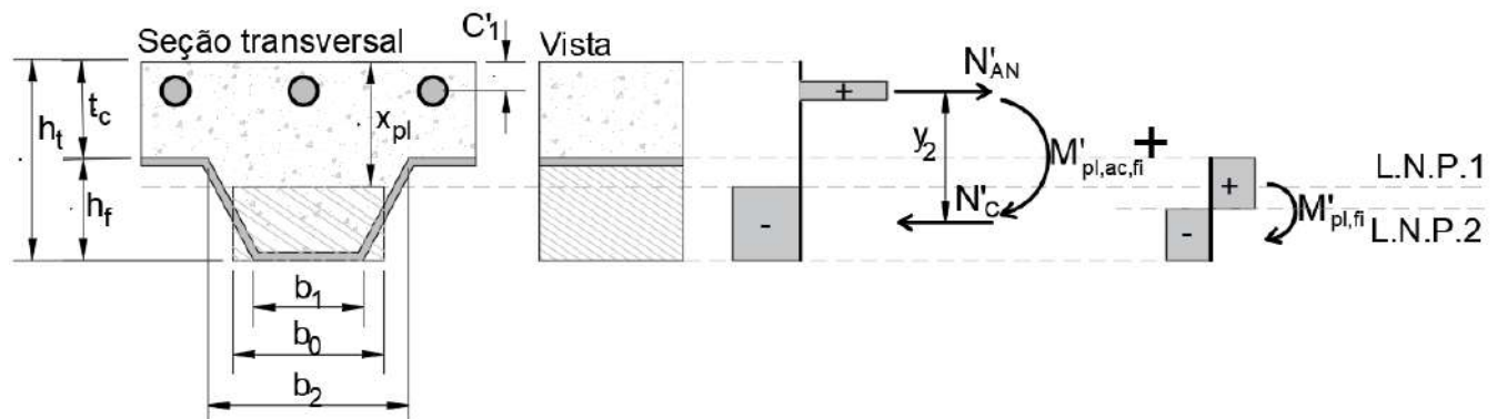
Figura 201 – Momento resistente negativo: armaduras negativas (caso II)
