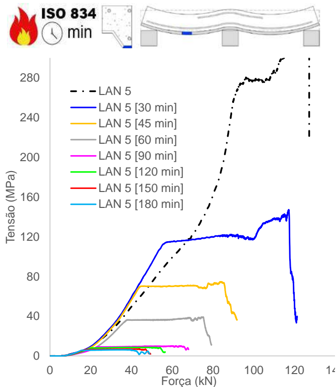
(d) Tensão chapa, mesa inferior (vão)
