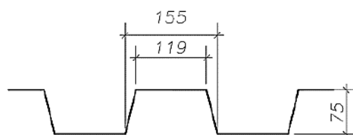
Figura 138 – Geometria da chapa perfilada com h_f = 75\text{mm}
