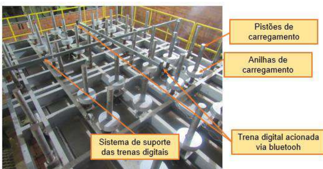
Figura 62 – Sistema de aplicação de carga e medição das deformações
