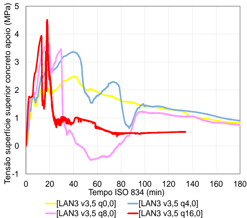
Figura 195 – Tensões no concreto, apoio intermediário (Co.5): vão 3,5 m
