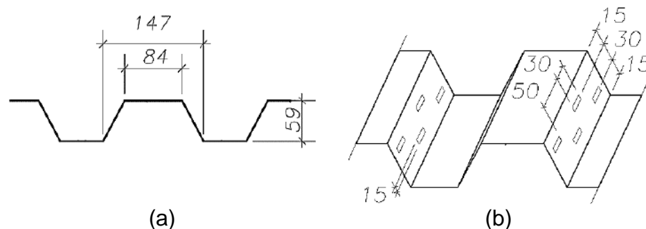
Figura 42 – Detalhe: (a) seção da chapa e (b) distribuição das mossas
