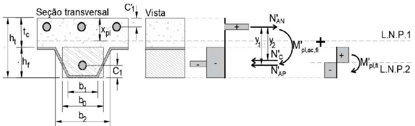
Figura 202 – Momento resistente negativo: armaduras positivas e negativas (I)
