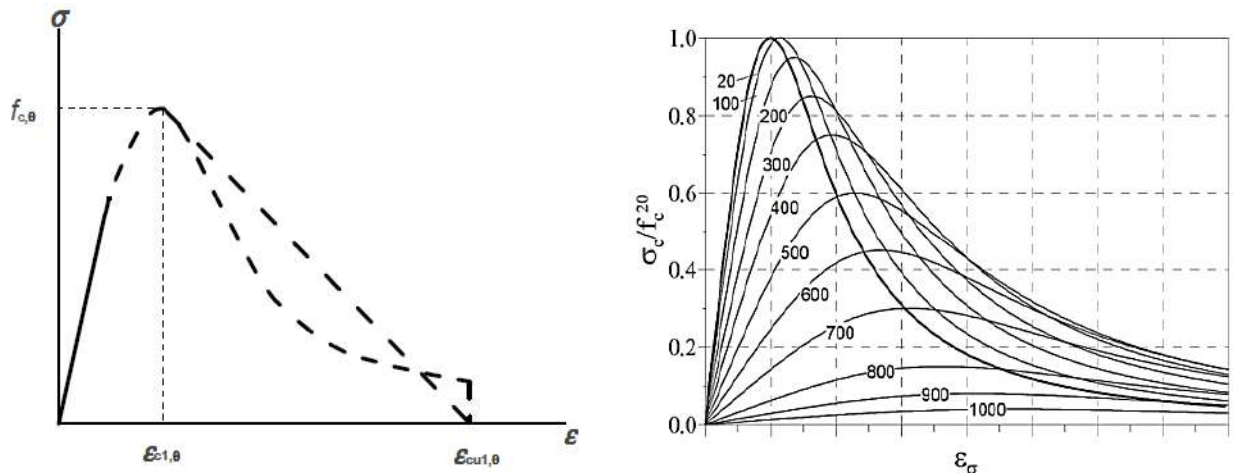
(a) Curva tensão vs deformação hipotética para o concreto proposto pela EN 1992-1.2
