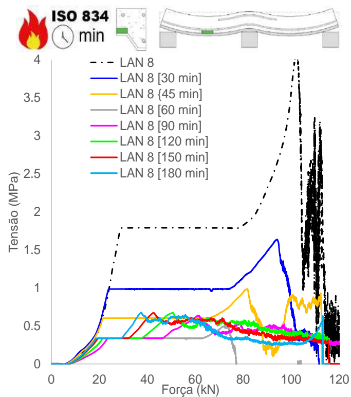
(n) Tensão concreto, adjacência mesa superior chapa (vão)
