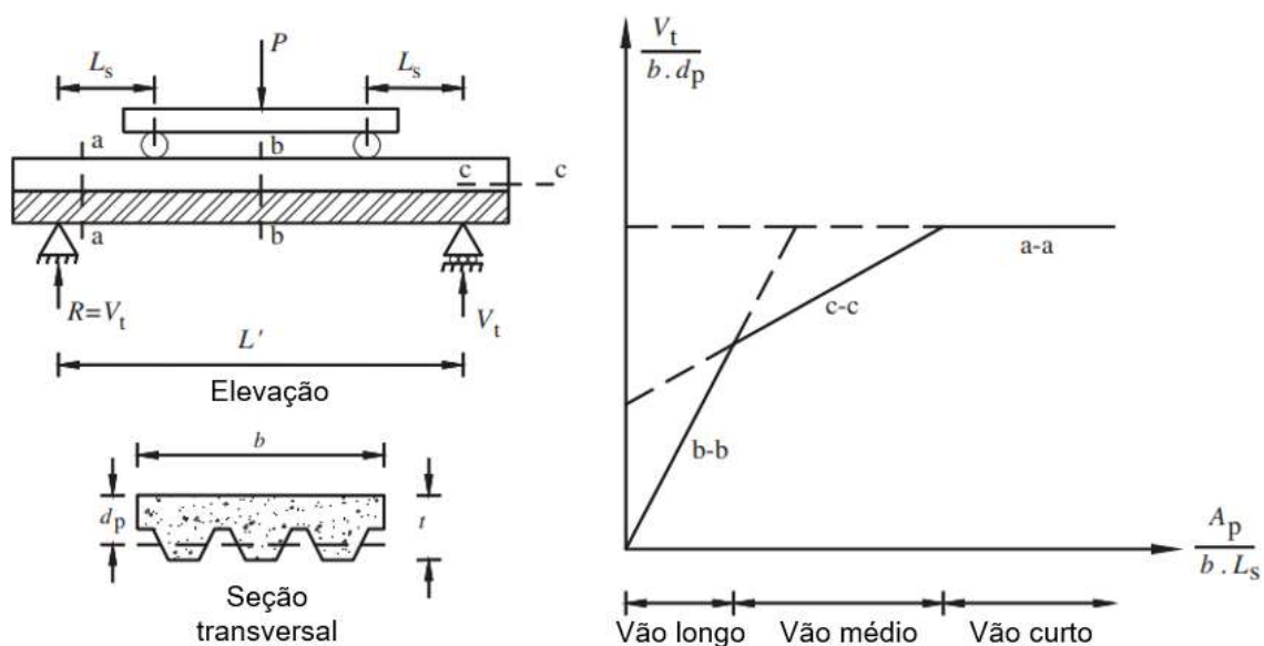
Figura 8 – Modos de ruptura de lajes mistas submetidas ao ensaio de flexão Fonte: adaptado de Gholamhoseini et al. (2014)
