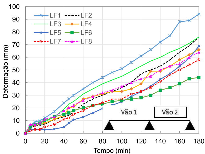
Figura 92 – Deformações (flechas) no vão 2 das lajes avaliadas em laboratório
