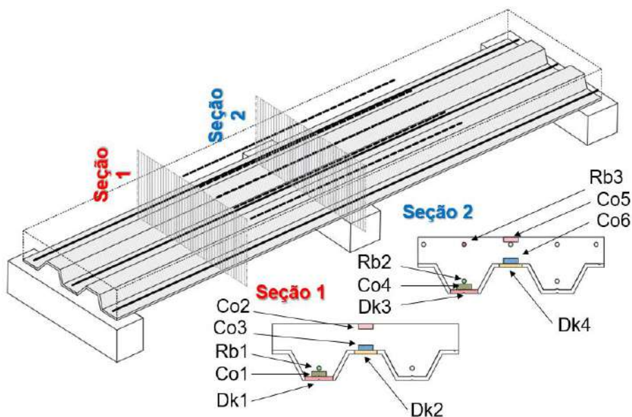
Figura 140 – Pontos de medição das tensões: lajes numericamente analisadas
