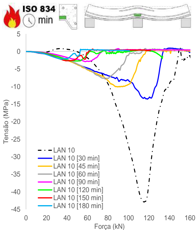
(k) Tensão concreto, adjacência mesa superior chapa (apoio)
