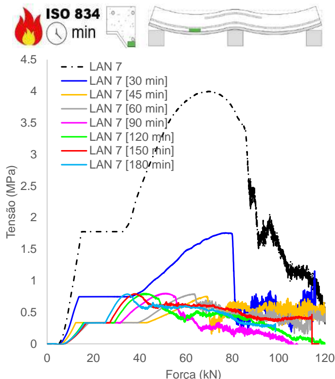
(k) Tensão concreto, adjacência mesa inferior chapa (vão)
