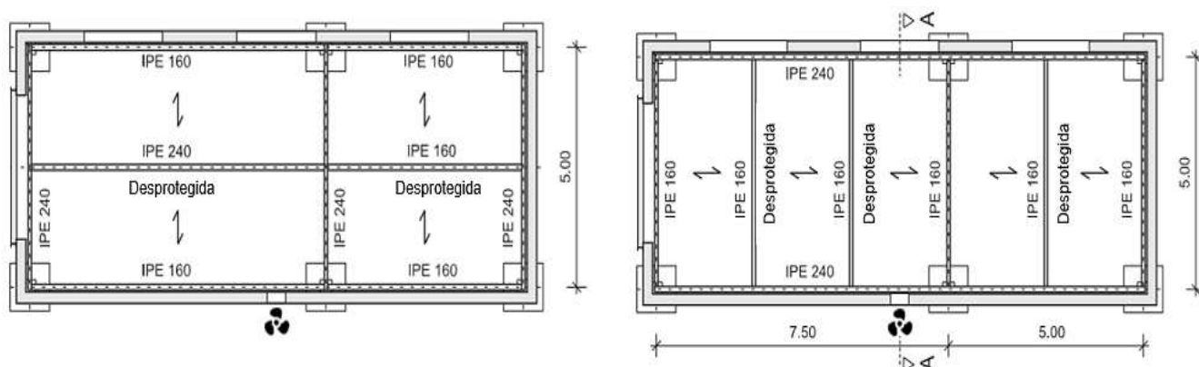
(a) Configuração do primeiro protótipo de laje
