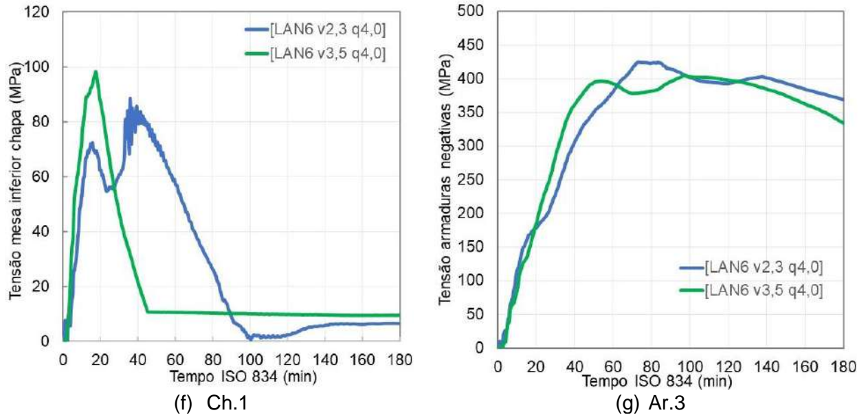
Figura 180 – Tensões na [LAN 6 v2,3 q4,0]
