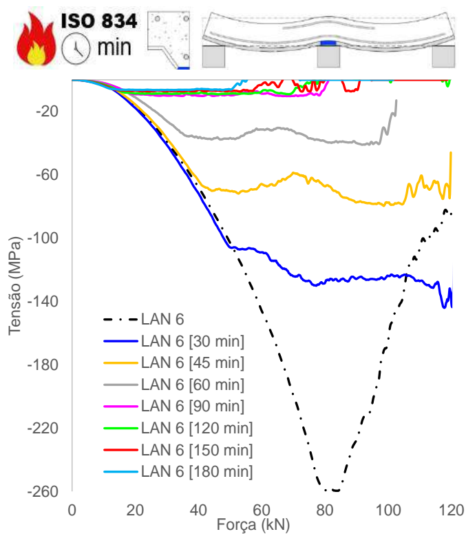
(f) Tensão chapa, mesa inferior (apoio)
