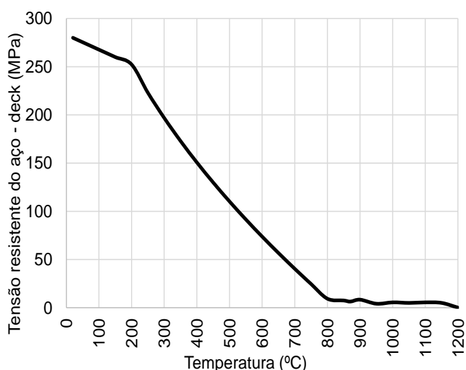
Figura 122 – Tensão resistente do aço da chapa: modelo numérico
