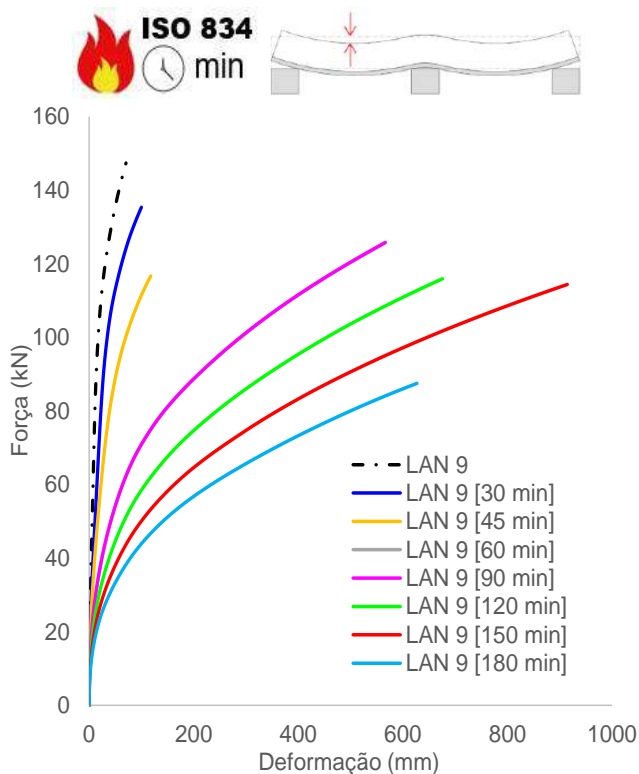
(a) Deformações verticais (flechas)
