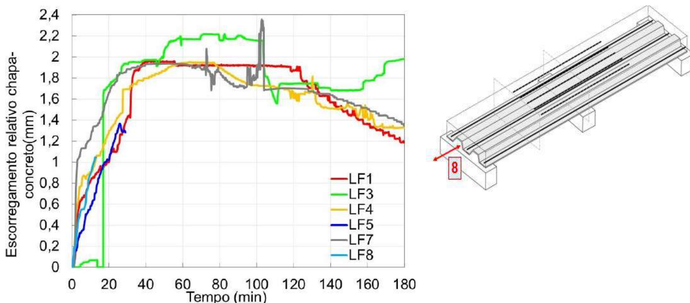
Figura 93 – Escorregamento relativo entre a chapa e o concreto
