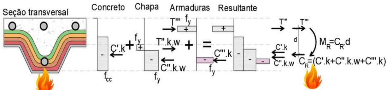
Figura 174 – Barras positivas e a continuidade ao incêndio (apoio intermediário)
