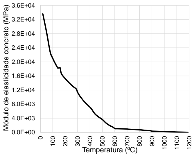
Figura 112 – Módulo de elasticidade longitudinal do concreto: modelo numérico
