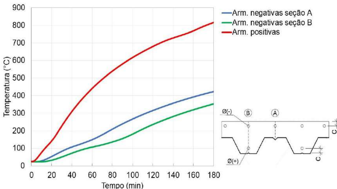
Figura 162 – Modelo numérico: temperaturas nas armaduras
