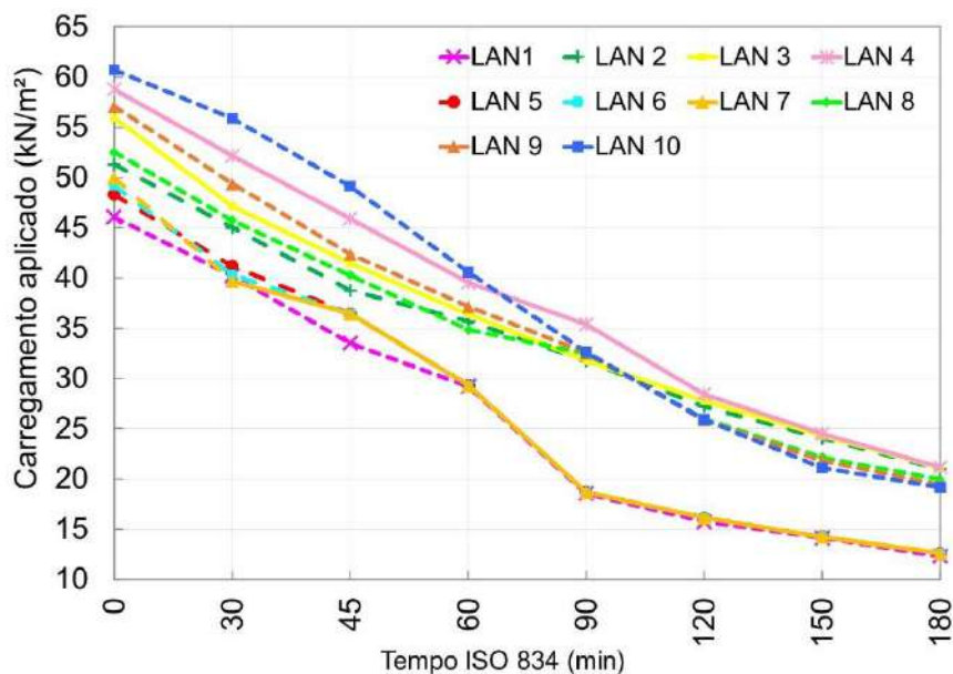
Figura 166 – Carregamentos últimos para diferentes tempos da ISO 834
