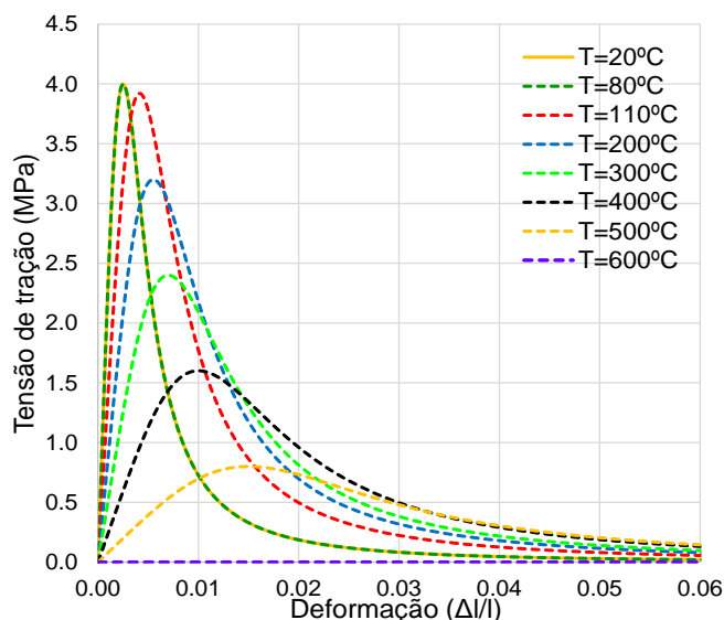
Figura 111 – Diagrama tensão-expansão do concreto: modelo numérico
