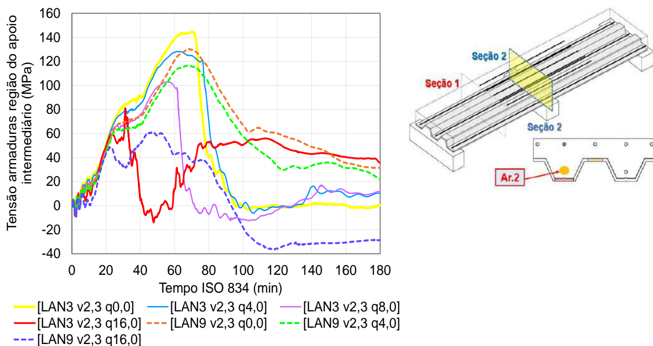
Figura 183 – Tensões produzidas nas armaduras positivas (Ar.2): vão de 2,3 m
