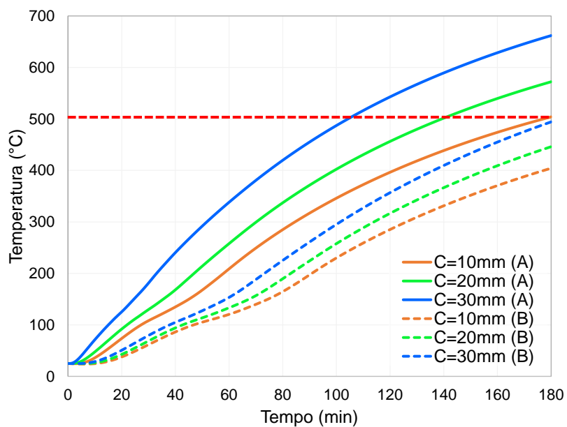
Figura 211 – Temperatura nas armaduras negativas, h_c=50\text{mm} e h_f=59\text{mm}
