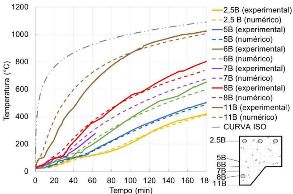
Figura 152 – Calibração das isotermas: alinhamento B da seção
