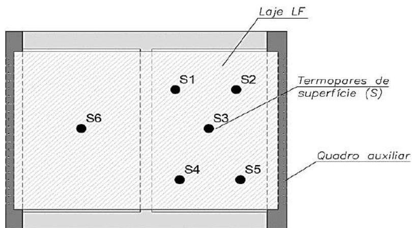
Figura 61 – Detalhe da locação dos termopares da superfície
