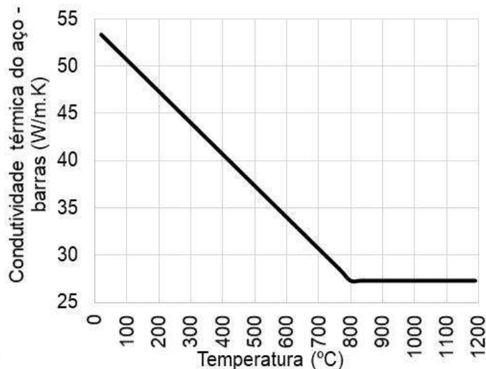
Figura 106 – Condutividade térmica do aço CA-50: modelo numérico
