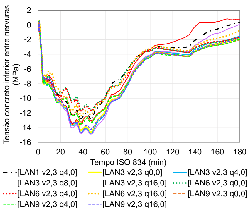
Figura 192 – Tensões produzidas no concreto, meio do vão (Co.3): 2,3 m
