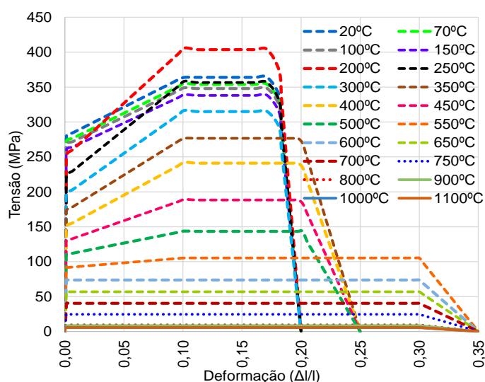
Figura 124 – Diagrama tensão-deformação da chapa: modelo numérico
