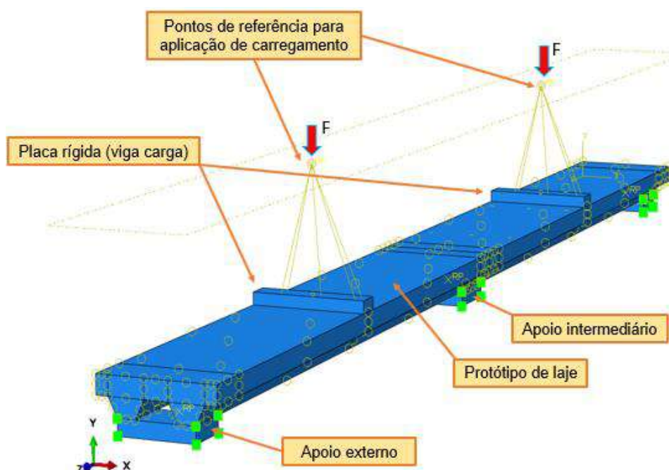
Figura 128 – Modelo de cálculo de calibração parâmetros mecânicos (modelo 1)
