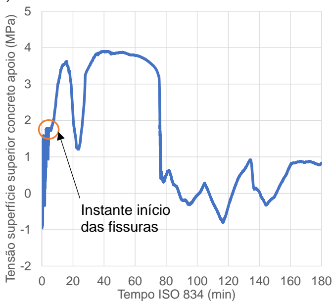
(b) tensões extraídas do modelo numérico
