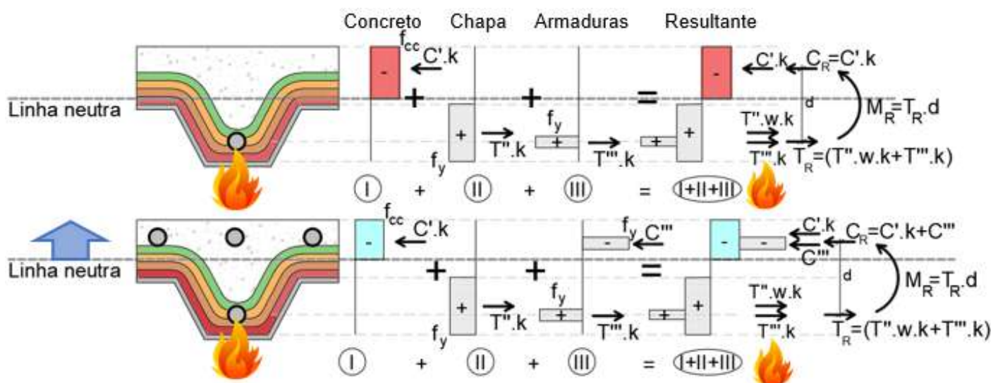
Figura 169 – Variação posição da linha neutra e as armaduras (meio do vão)
