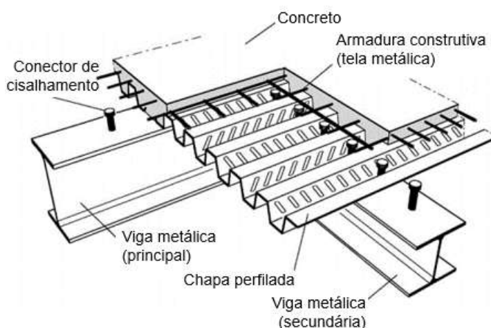
Figura 1 – Laje mista de aço e concreto Fonte: adaptado de Crisinel e Marimon (2004)
