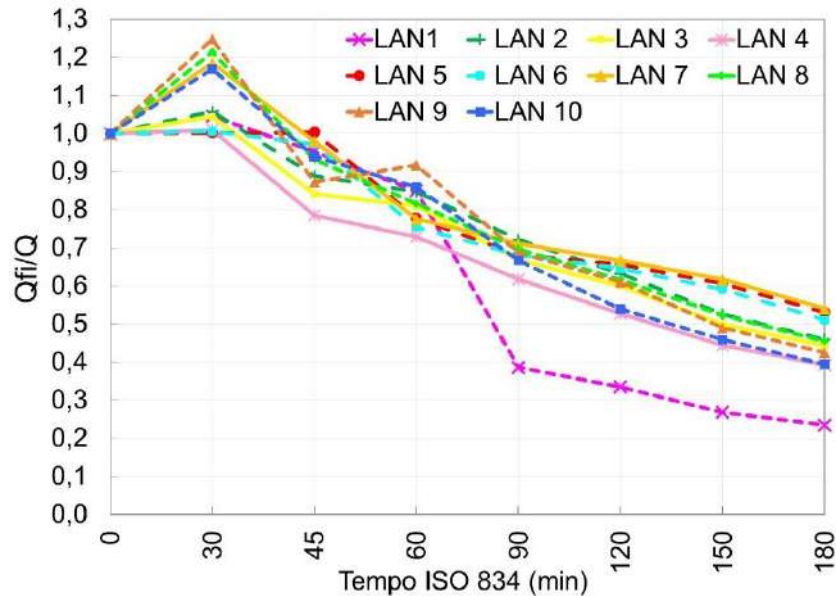
Figura 172 – Coeficiente de redução da resistência por laje
