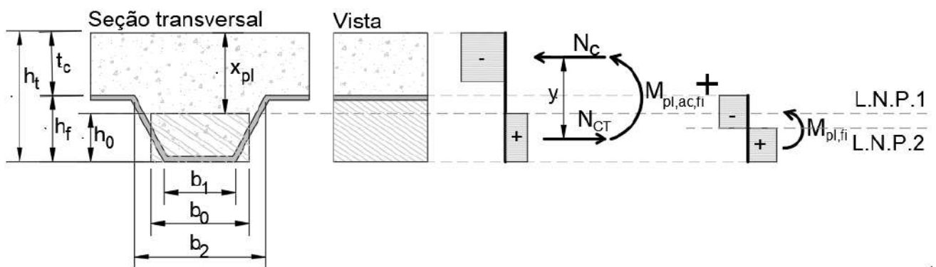
Figura 197 – Momento resistente positivo: sem armaduras (caso II)
