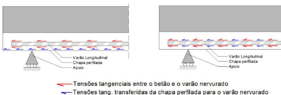
Figura 16 - Tensões (a) antes e (b) após a perda de atrito aço-concreto
