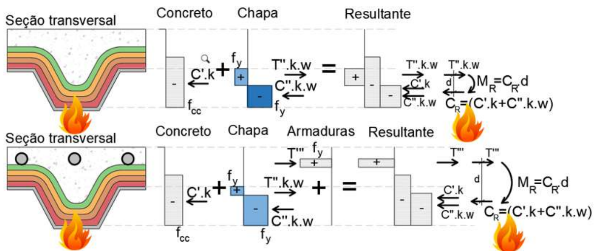
Figura 173 – Laje sem e com barras negativas: esforços na chapa
