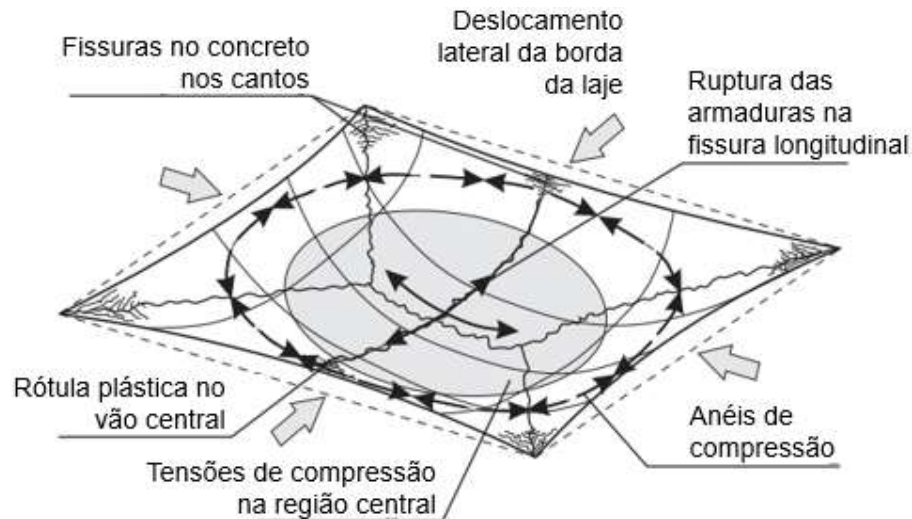
Figura 25 – Sistemática do comportamento de membrana Fonte: adaptado de Herraiz e Vogel (2016)
