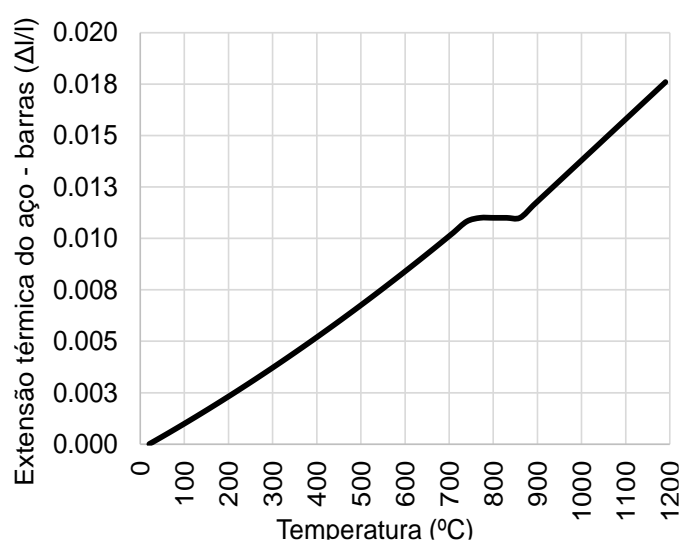
Figura 121 – Extensão térmica do aço CA-50: modelo numérico
