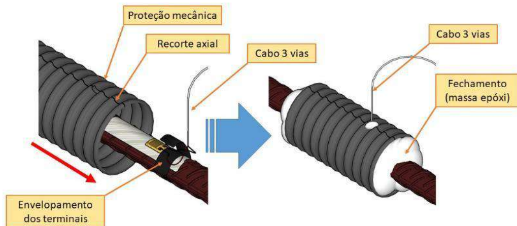
Figura 56 – Detalhe da instalação mecânica dos extensômetros
