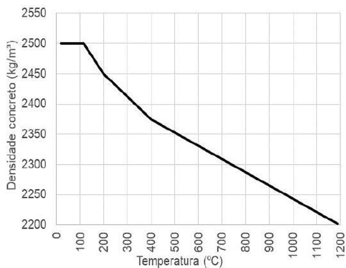
Figura 103 – Variação da densidade do concreto: modelo numérico
