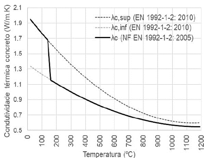
Figura 104 – Condutividade térmica do concreto: modelo numérico
