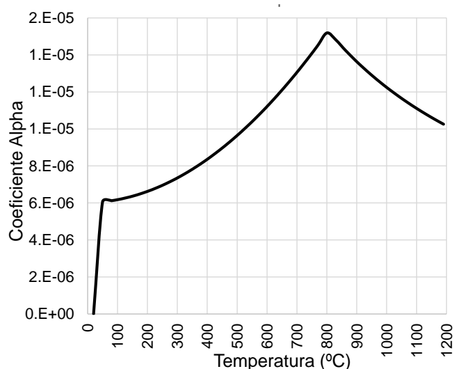
Figura 115 – Coeficiente alpha do concreto: modelo numérico
