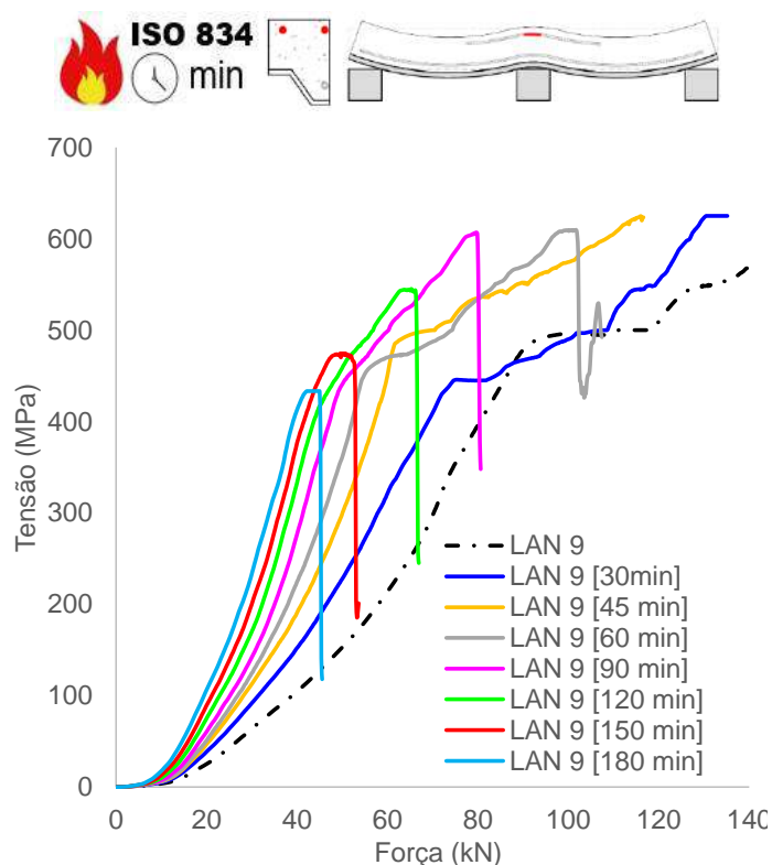
(d) Tensão armaduras negativas (apoio)
