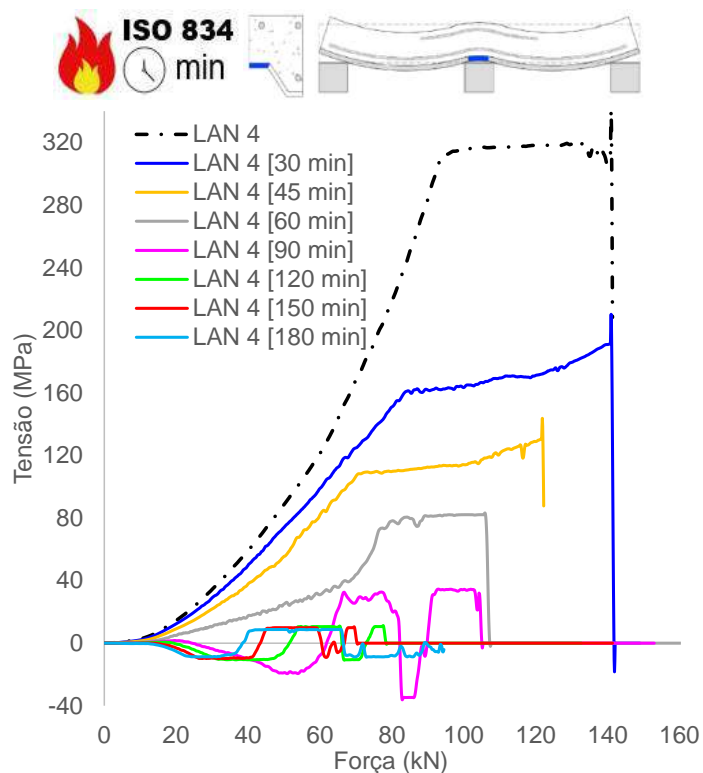
(g) Tensão chapa, mesa superior (apoio)
