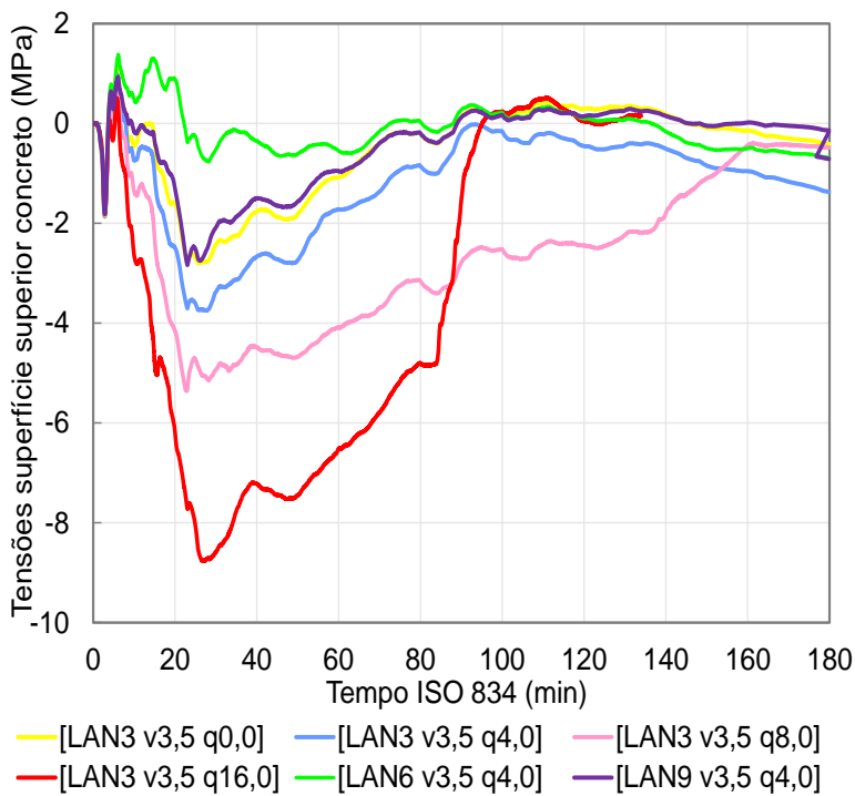
Figura 191 – Tensões no concreto, meio do vão (Co.2): vão 3,5 m
