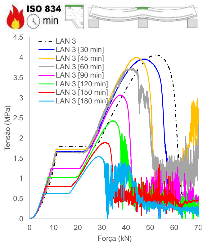
(i) Tensão concreto, superfície superior (apoio)
