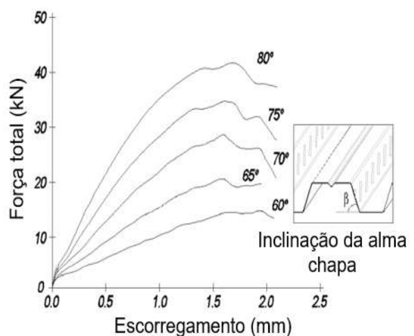
(d) inclinação da alma da chapa perfilada em relação a horizontal
