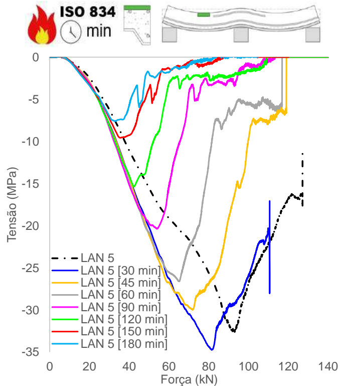
(l) Tensão concreto, superfície superior (vão)
