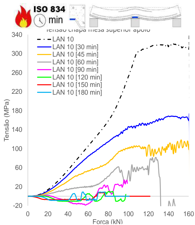
(g) Tensão chapa, mesa superior (apoio)
