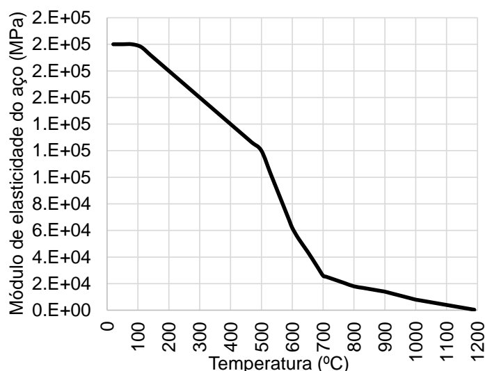
Figura 119 – Módulo elasticidade do aço CA-50: modelo numérico
