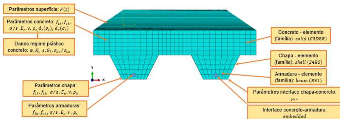
Figura 129 – Modelo de cálculo: análise numérica - parâmetros mecânicos
