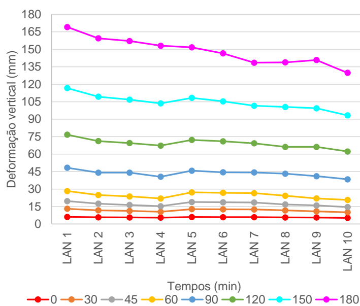
(b) Força aplicada de 50 kN
