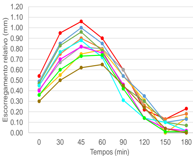
(a) Força aplicada de 25 kN
