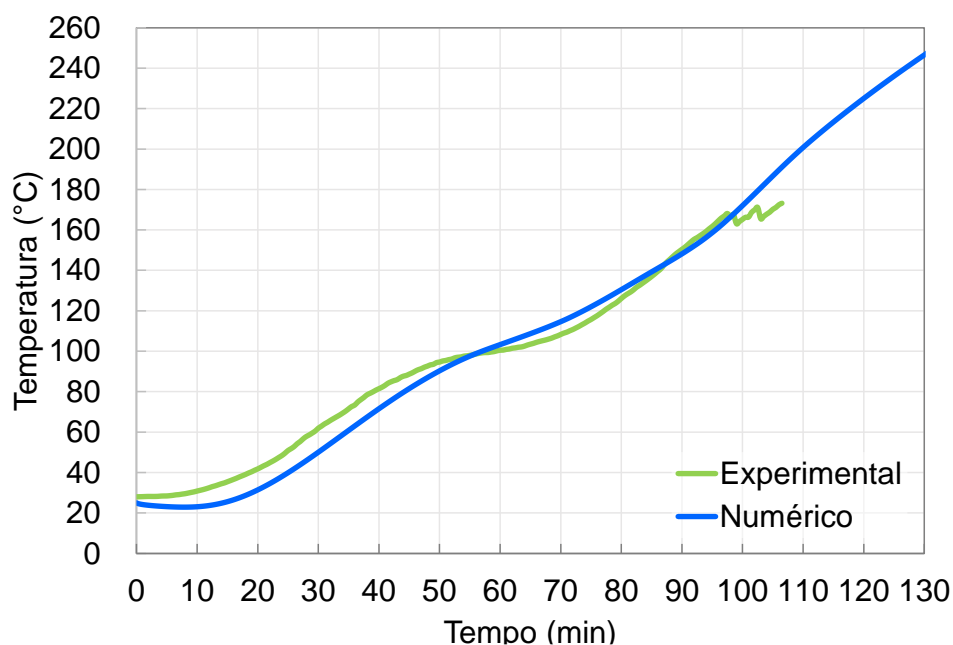
Figura 150 – Calibração do isolamento térmico
