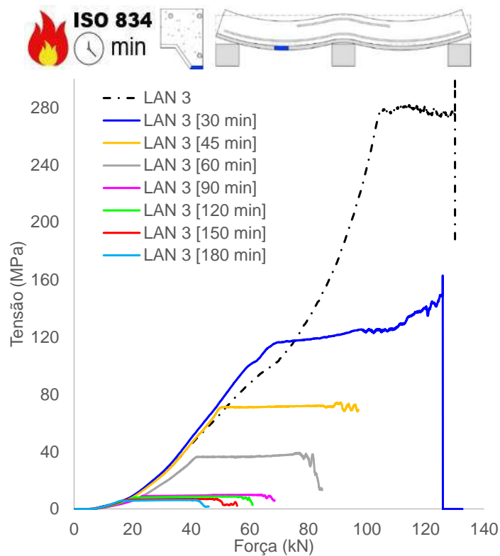
(f) Tensão chapa, mesa inferior (vão)
