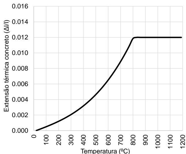
Figura 114 – Extensão térmica do concreto: modelo numérico
