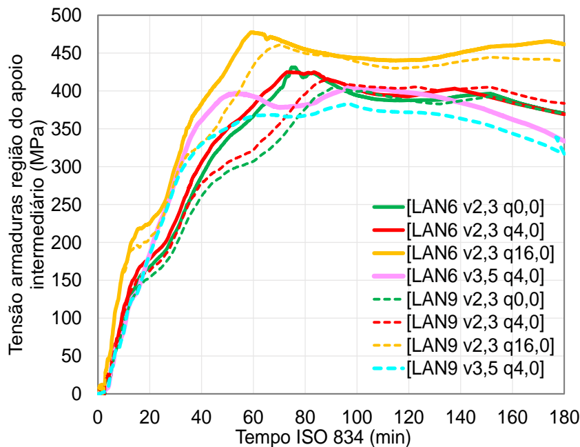
Figura 185 – Tensões produzidas nas armaduras negativas (Ar.3)
