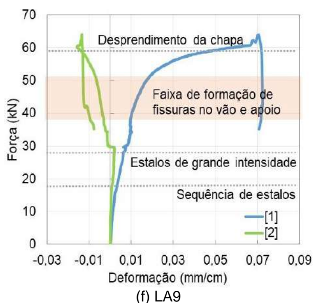
Figura 64 – Alongamento da mesa superior e inferior da chapa no meio do vão
