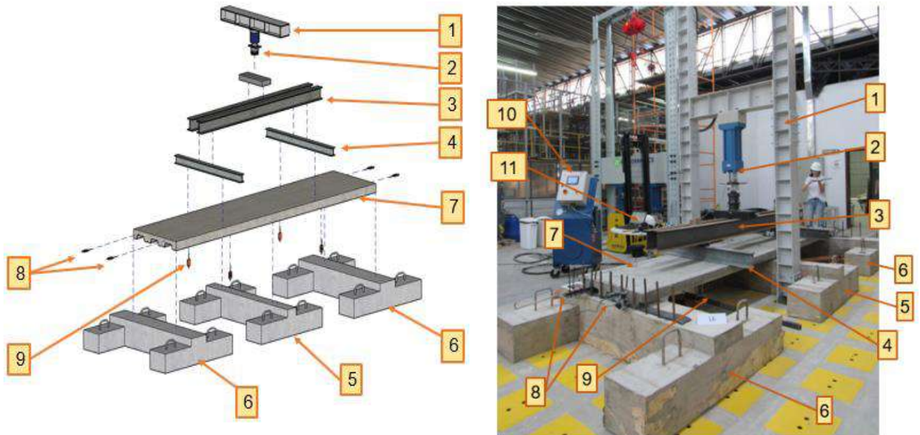
Figura 49 – Esquema do ensaio de laje mista contínua para análise da LA
