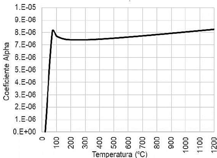
Figura 127 – Coeficiente alpha do aço da chapa: modelo numérico
