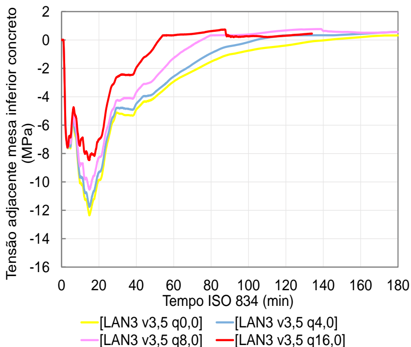
Figura 189 – Tensões produzidas no concreto, meio do vão (Co.1): vão 3,5 m
