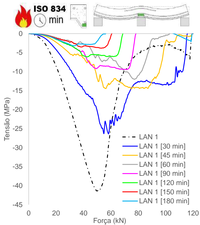
(h) Tensão concreto, adjacência mesa inferior chapa (apoio)
