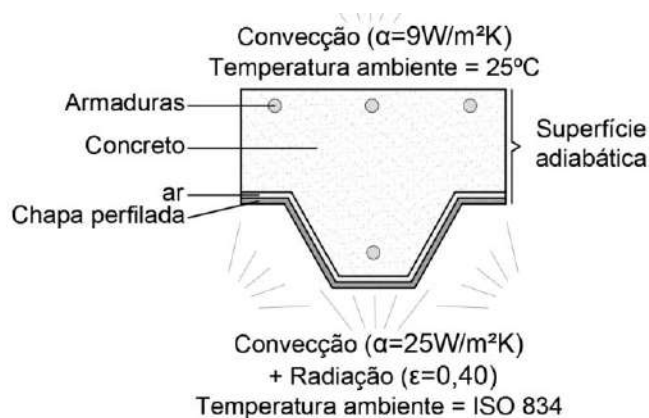
Figura 131 – Modelo de análise térmica da seção
