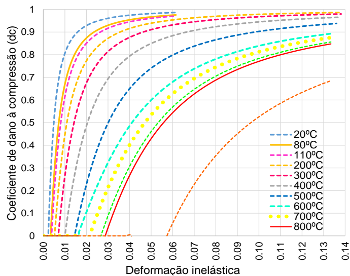
Figura 116 – Coeficiente de dano ao concreto comprimido: modelo numérico
