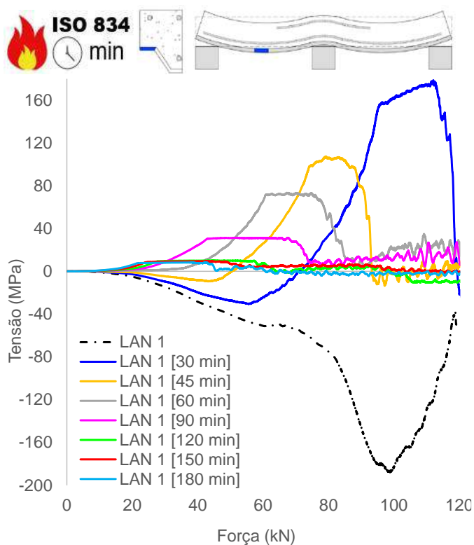
(c) Tensão chapa, mesa superior (vão)
