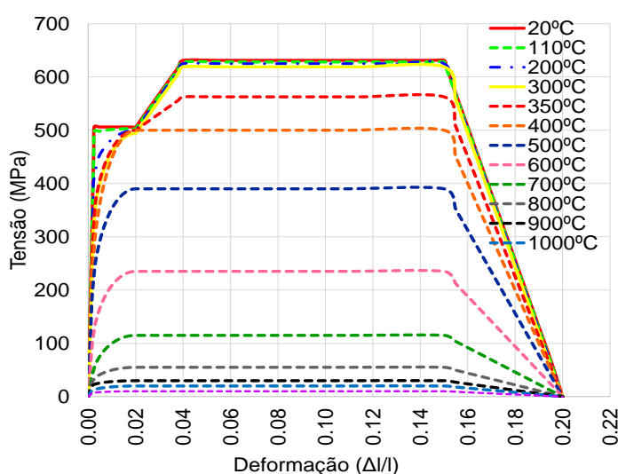
Figura 120 – Diagrama tensão-deformação do aço CA-50: modelo numérico
