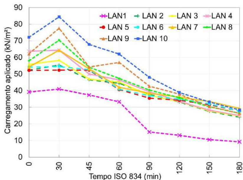
Figura 171 – Carregamentos últimos conforme a ISO 834
