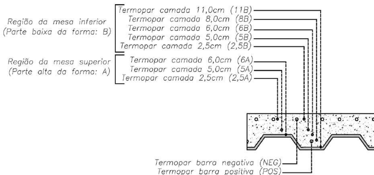
Figura 60 – Detalhe da locação dos termopares na seção da laje
