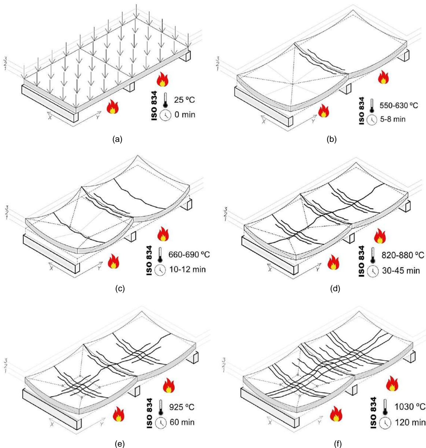
Figura 76 – Performance da laje na relação tempo-temperatura da ISO 834
