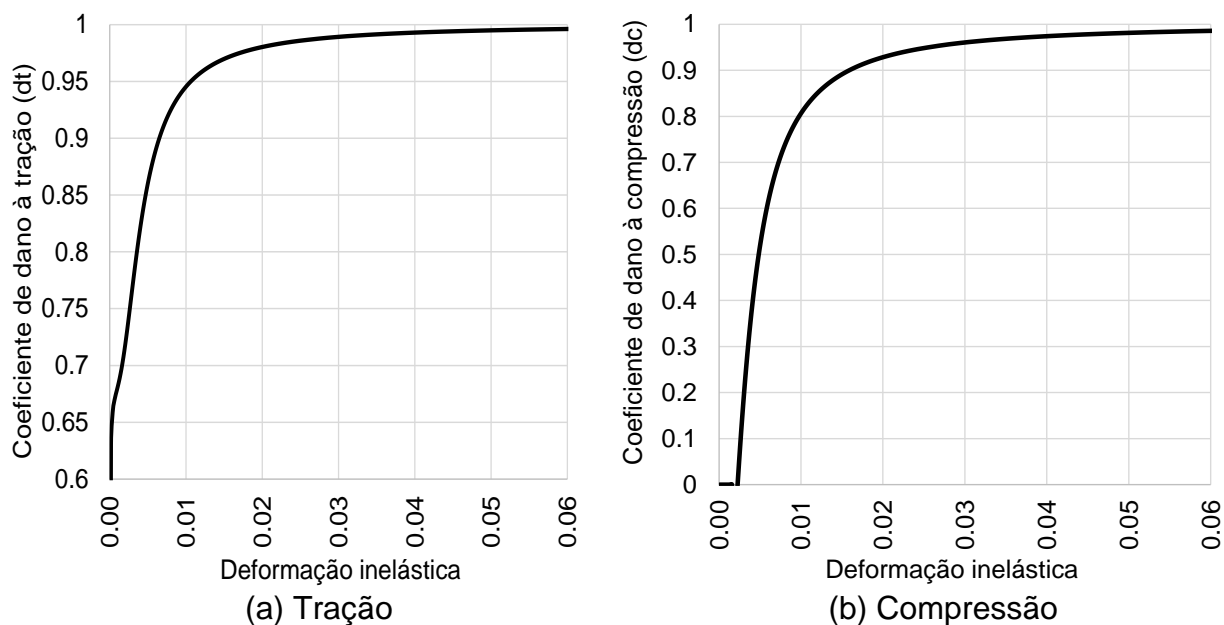
Figura 99 – Parâmetro de dano ao concreto
