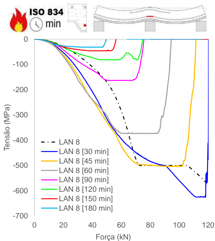
(c) Tensão armaduras positivas (apoio)
