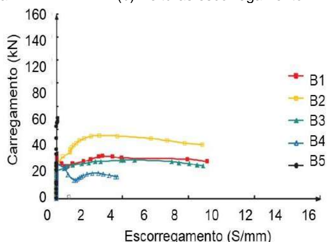
(d) Lajes com vão de 800 mm
