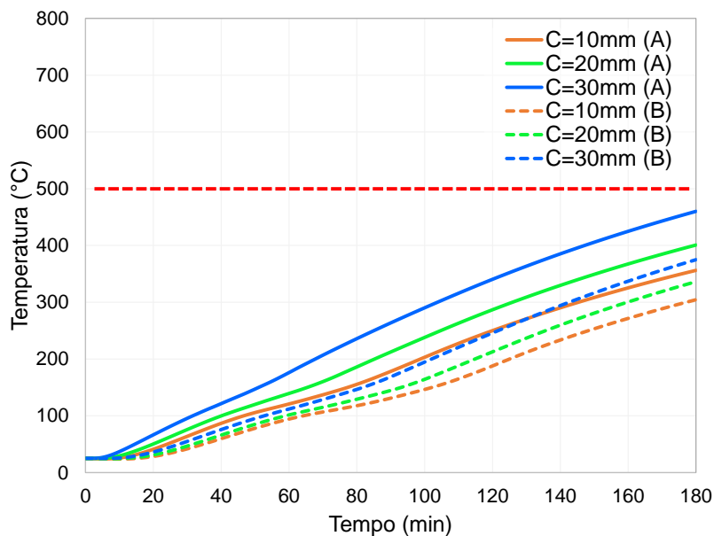
Figura 213 – Temperatura nas armaduras negativas, h_c=70\text{mm} e h_f=59\text{mm}
