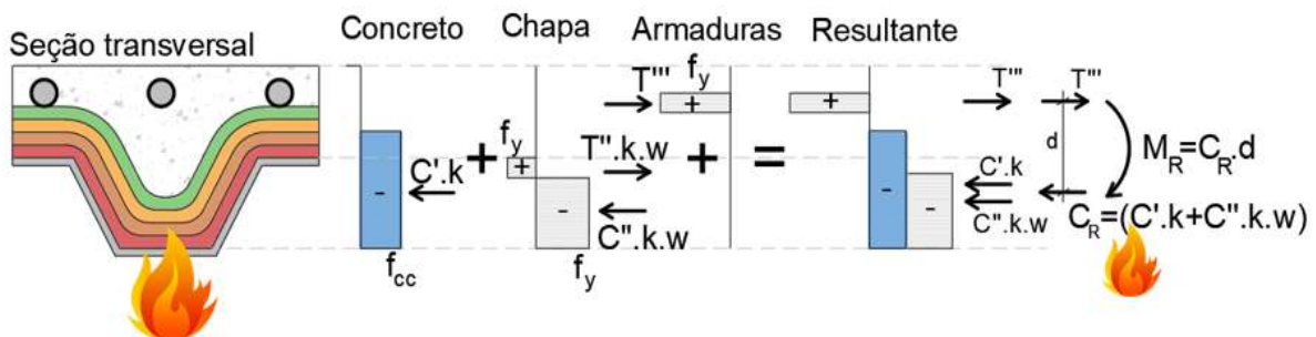
Figura 175 – Esforços concreto comprimido (apoio intermediário)
