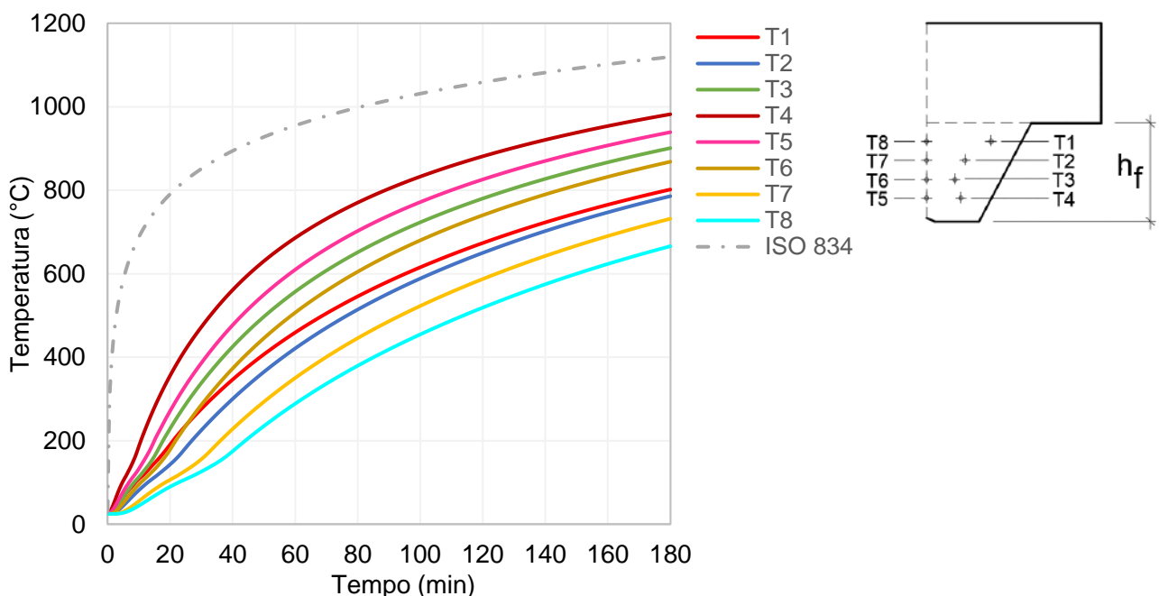
Figura 204 – Temperatura no concreto na nervura, laje com h_f = 59\text{mm}
