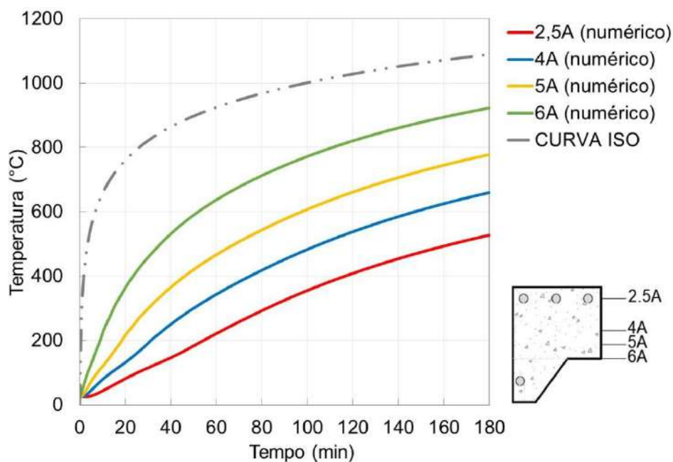
Figura 164 – Modelo numérico: temperaturas no concreto (linha A da seção)
