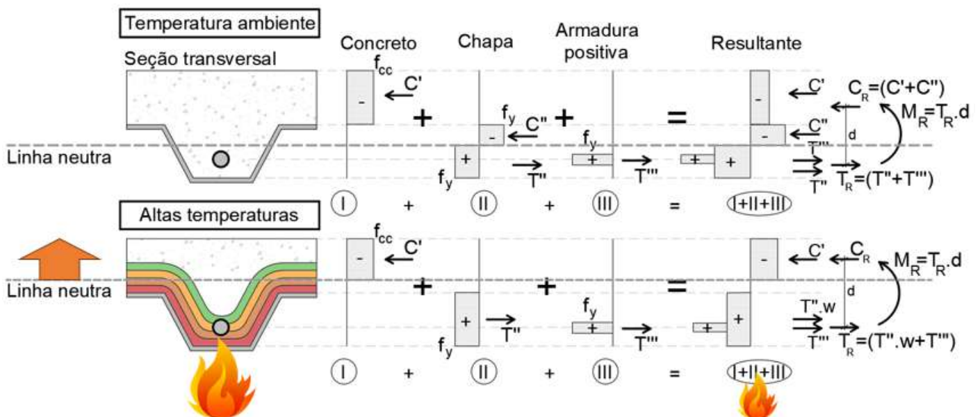
Figura 168 – Esforços na seção em altas temperaturas (meio do vão)
