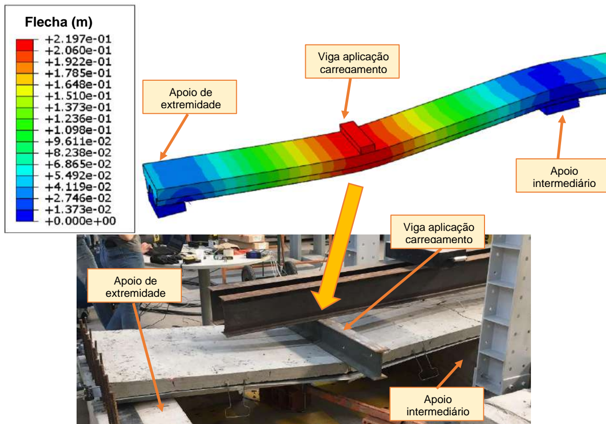
Figura 147 – Deformações verticais totais: comparativo entre ME e MN
