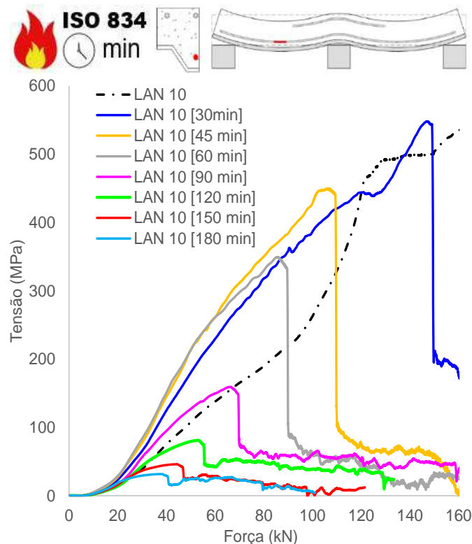
(b) Tensão armaduras positivas (vão)
