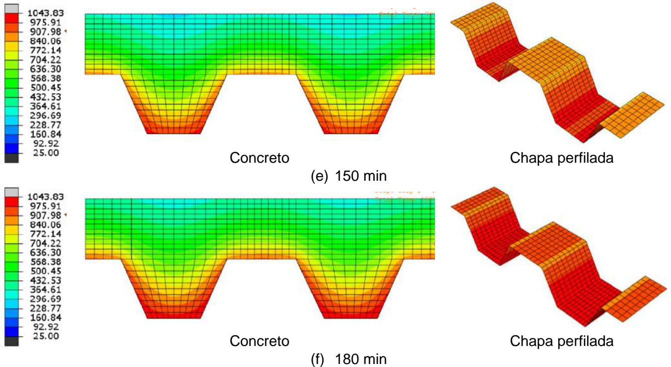
Figura 161 – Isotermas da seção para diferentes tempos da ISO 834
