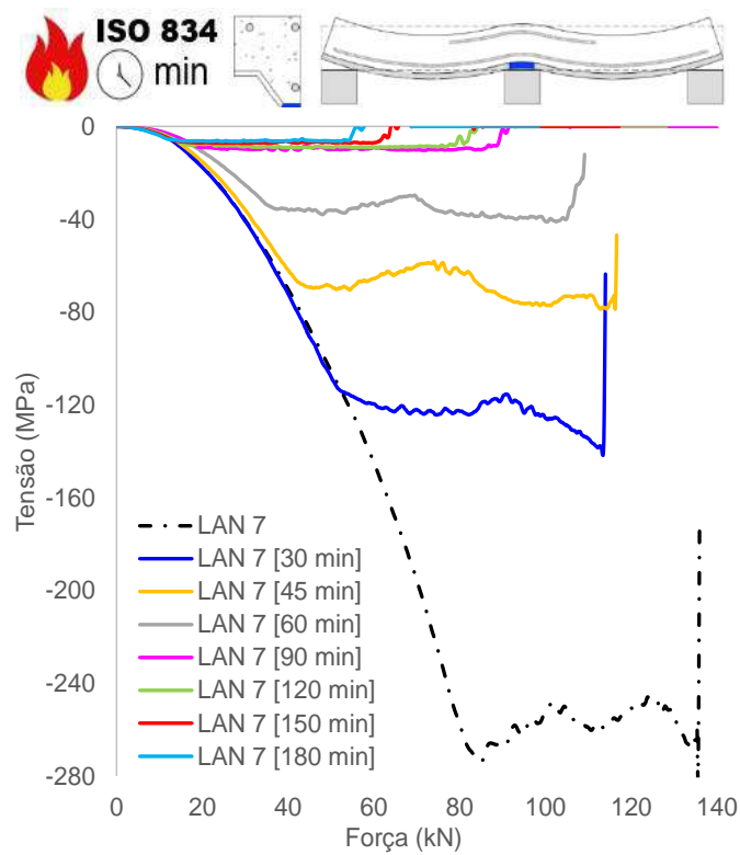
(f) Tensão chapa, mesa inferior (apoio)
