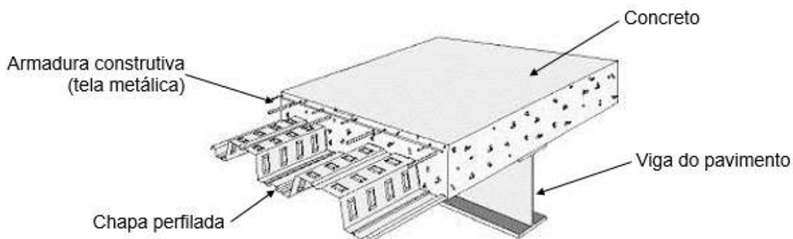
Figura 6 – Detalhe de uma laje mista de aço e concreto Fonte: Campos (2001)
