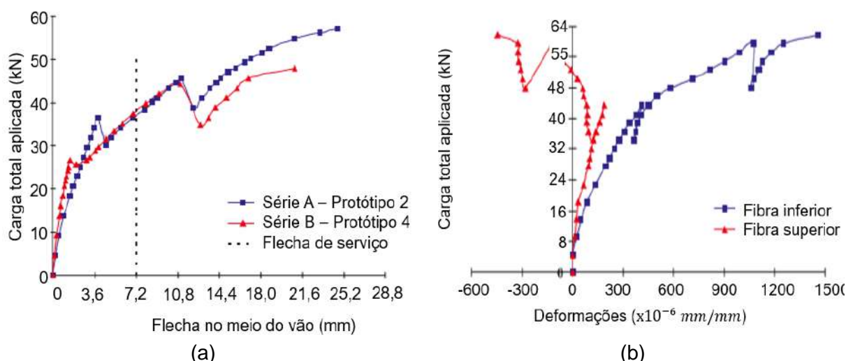
Figura 13 – Carregamento vs (a) flecha e (b) deformações longitudinais Fonte: Calixto, Brendolan e Pimenta (2009)
