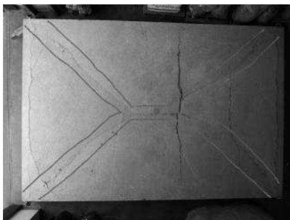
(c) Fissuras ensaio a temperatura ambiente
