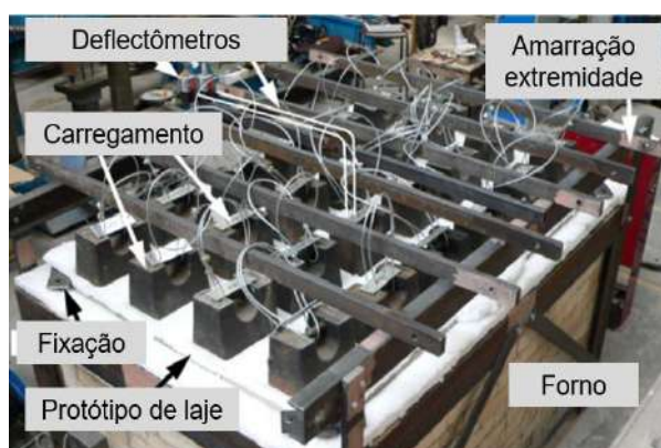
(a) Configuração do ensaio experimental
