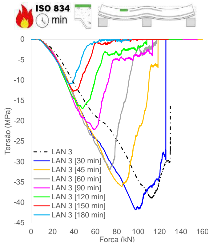
(b) Tensão concreto, superfície superior (vão)
