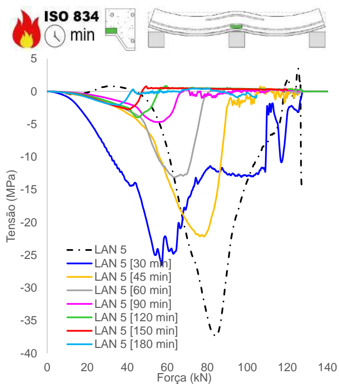
(i) Tensão concreto, adjacência mesa superior chapa (apoio)
