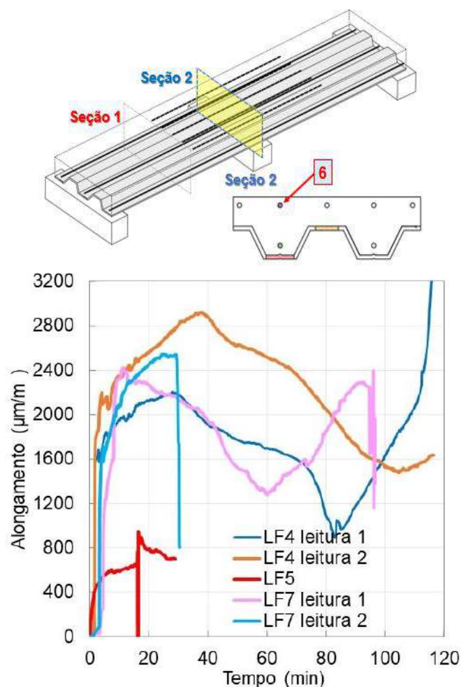
Figura 90 – Deformação longitudinal armaduras negativas
