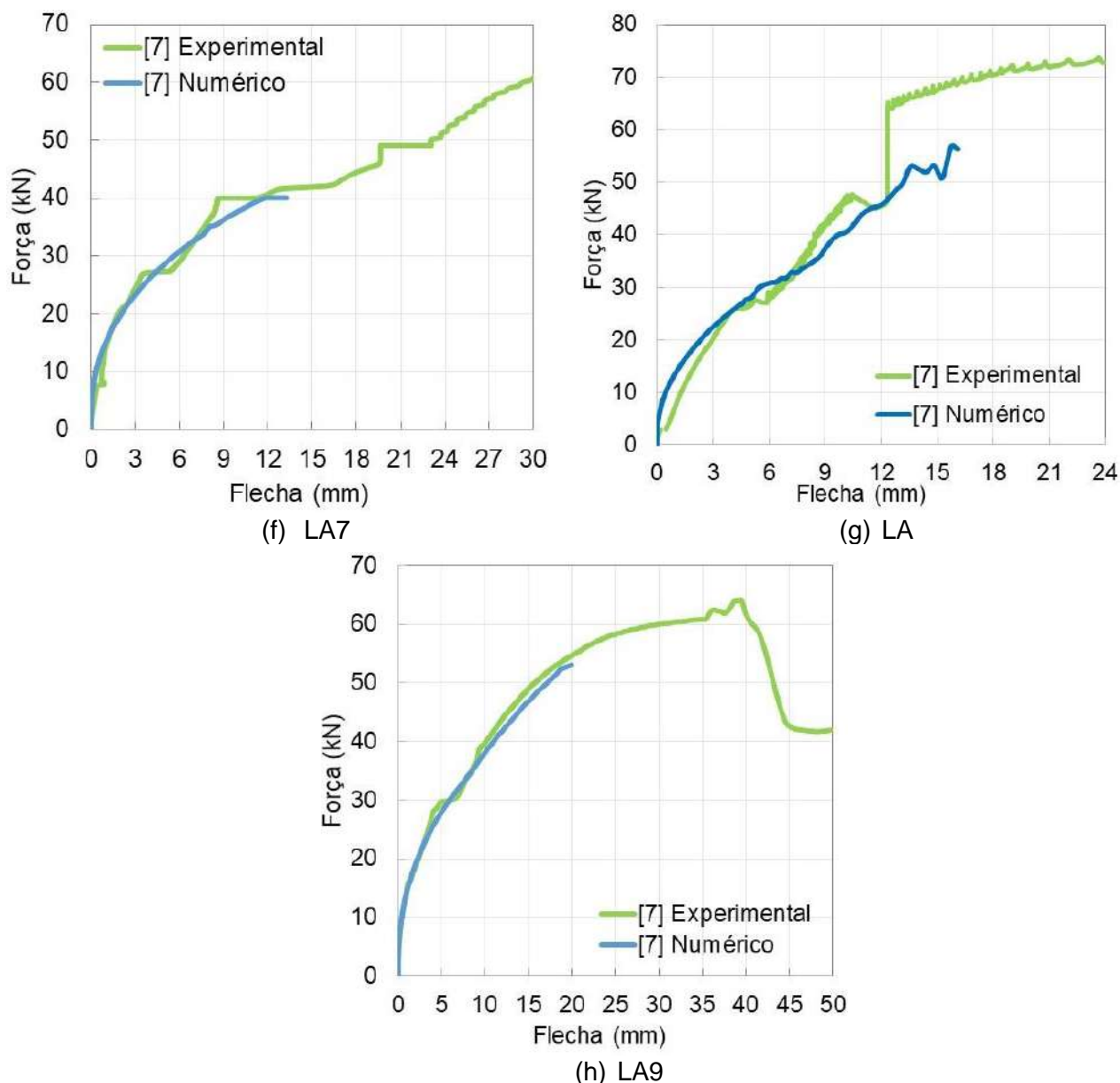
Figura 146 – Calibração da deformação vertical (flecha)
