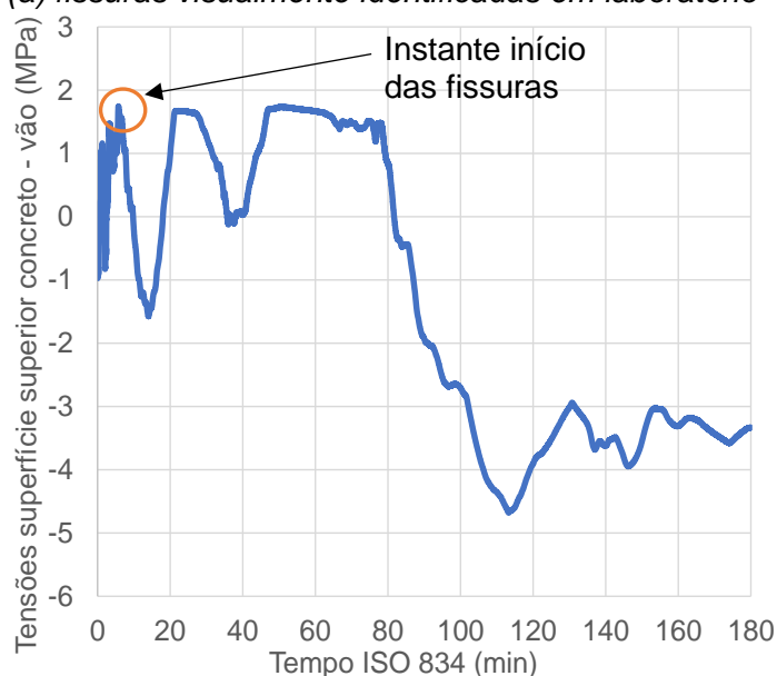
(b) tensões extraídas do modelo numérico
