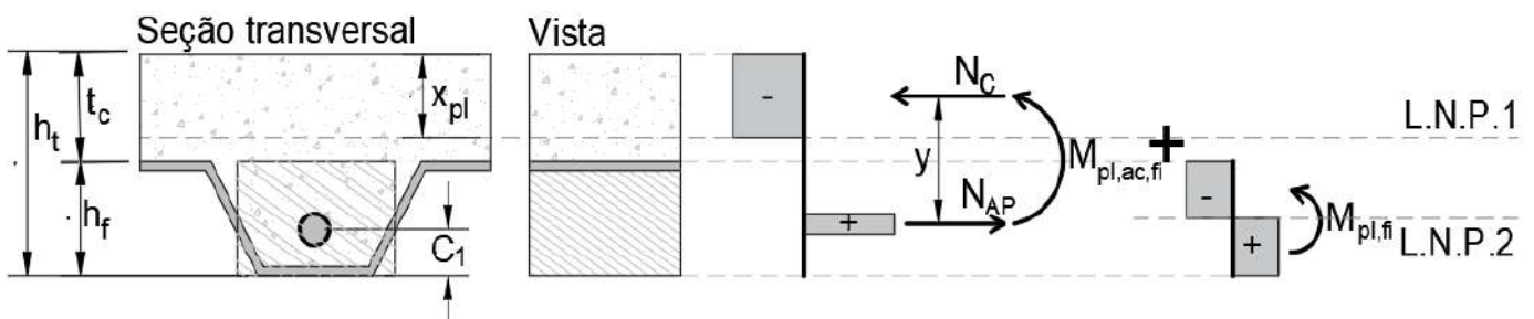
Figura 198 – Momento resistente positivo: armaduras positivas (caso I)
