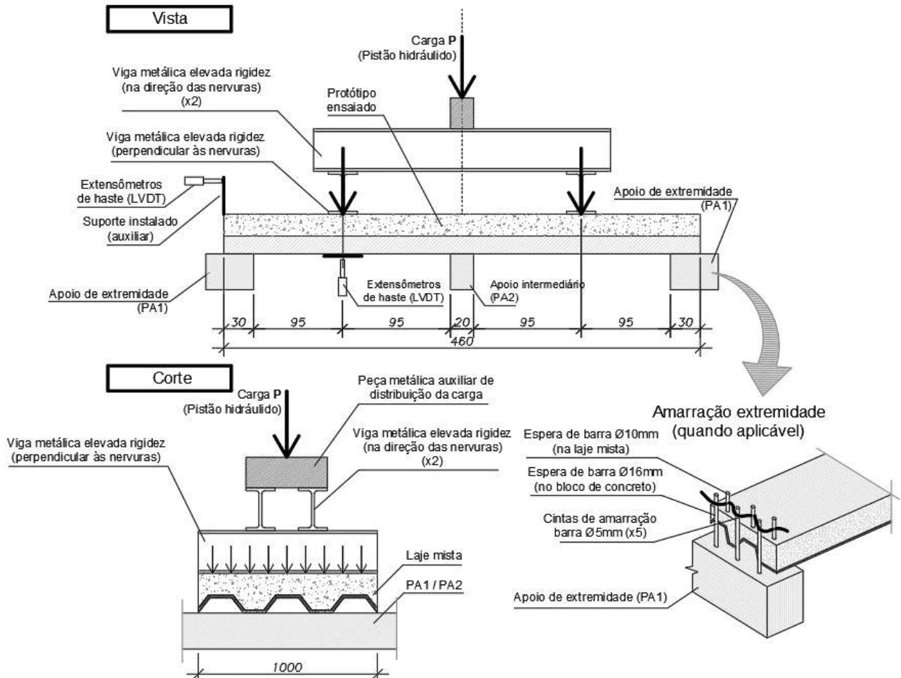
Figura 49 – Esquema do ensaio de laje mista contínua para análise da LA
