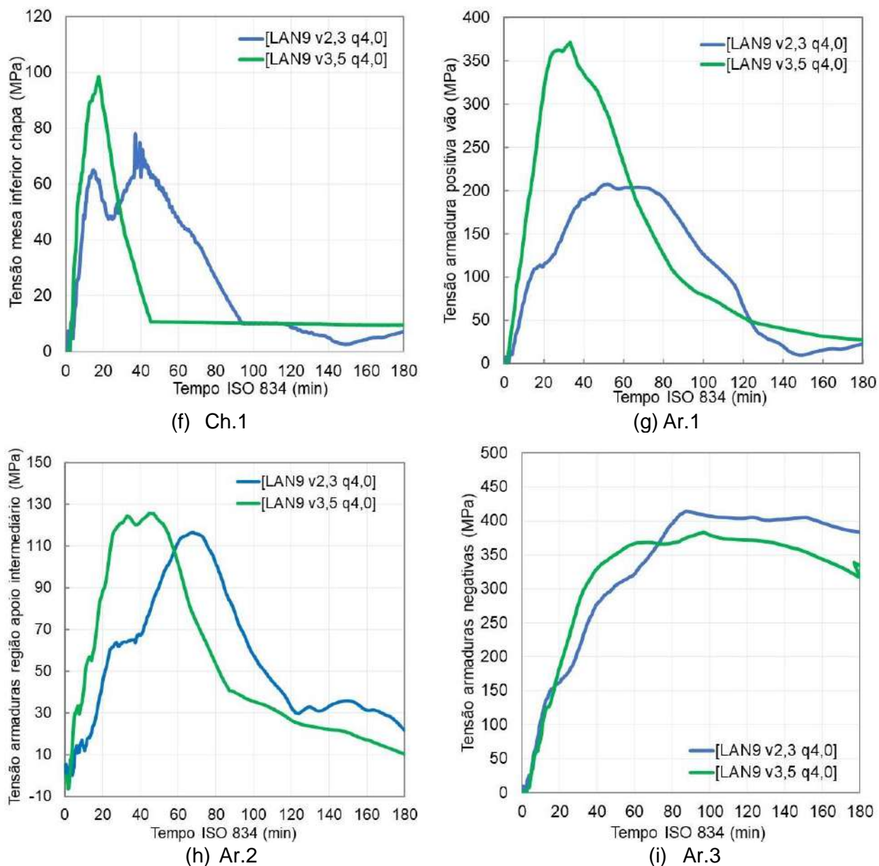
Figura 181 – Tensões na [LAN 9 v2,3 q4,0]
