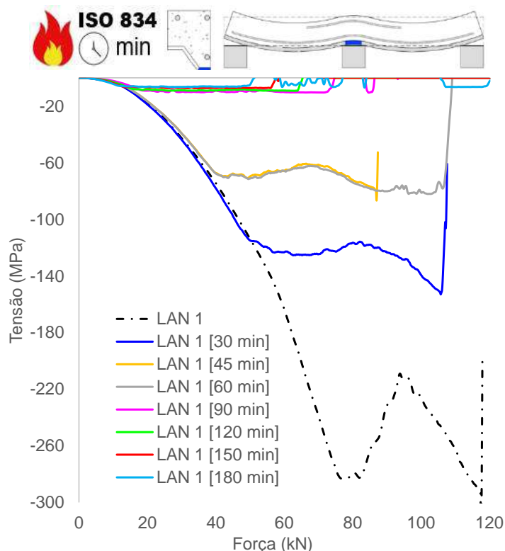
(f) Tensão chapa, mesa inferior (apoio)
