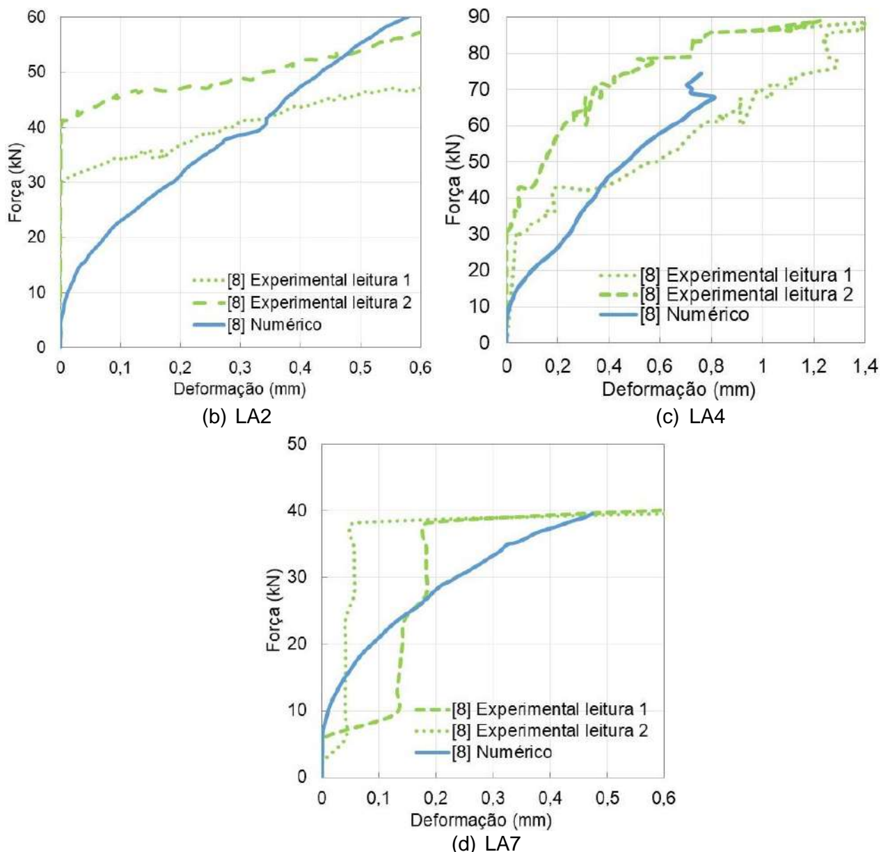
Figura 148 –Calibração do escorregamento relativo chapa-concreto
