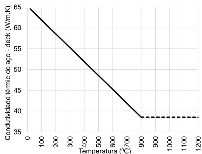
Figura 125 – Condutividade térmica do aço da chapa: modelo numérico
