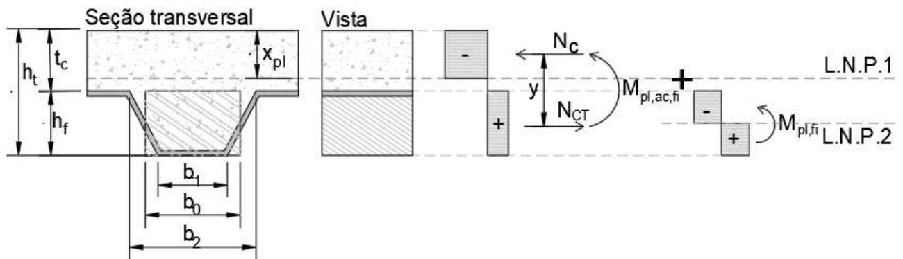
Figura 196 – Momento resistente positivo: sem armaduras (caso I)
