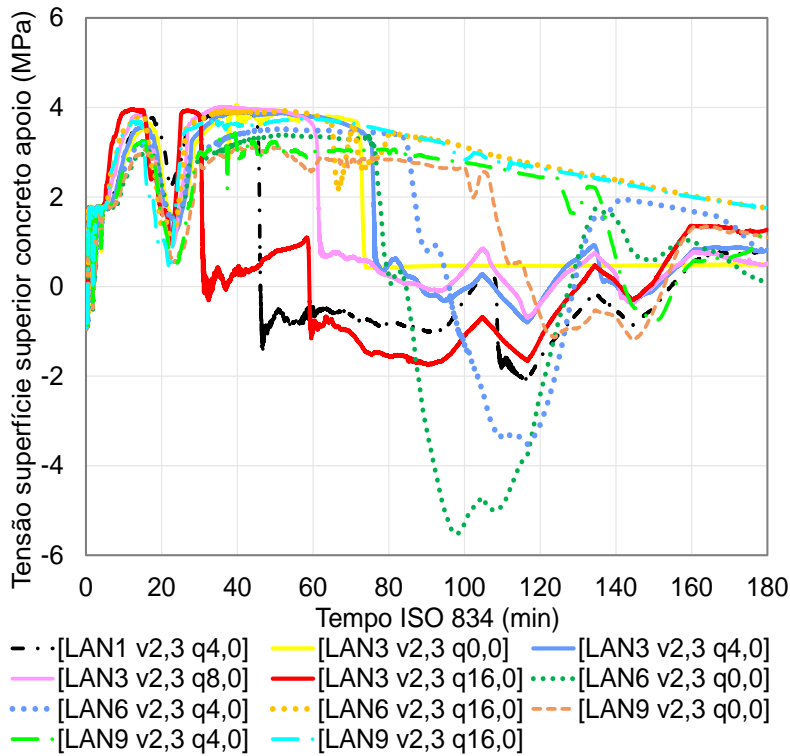
Figura 194 – Tensões no concreto, apoio intermediário (Co.5): vão 2,3 m
