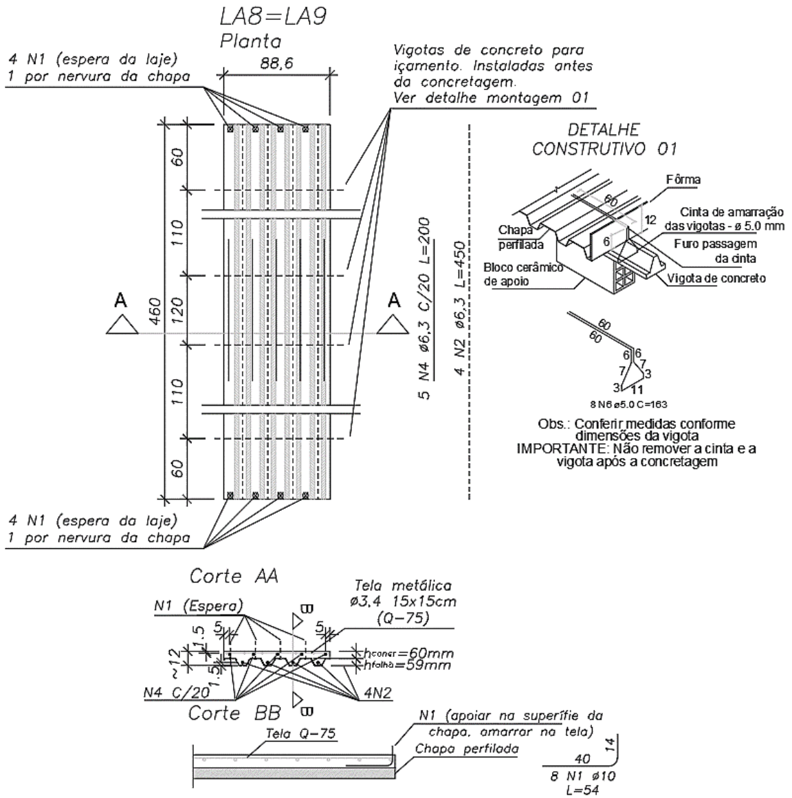
Figura 43 – Detalhamento estrutural das lajes LA8 e LA9
