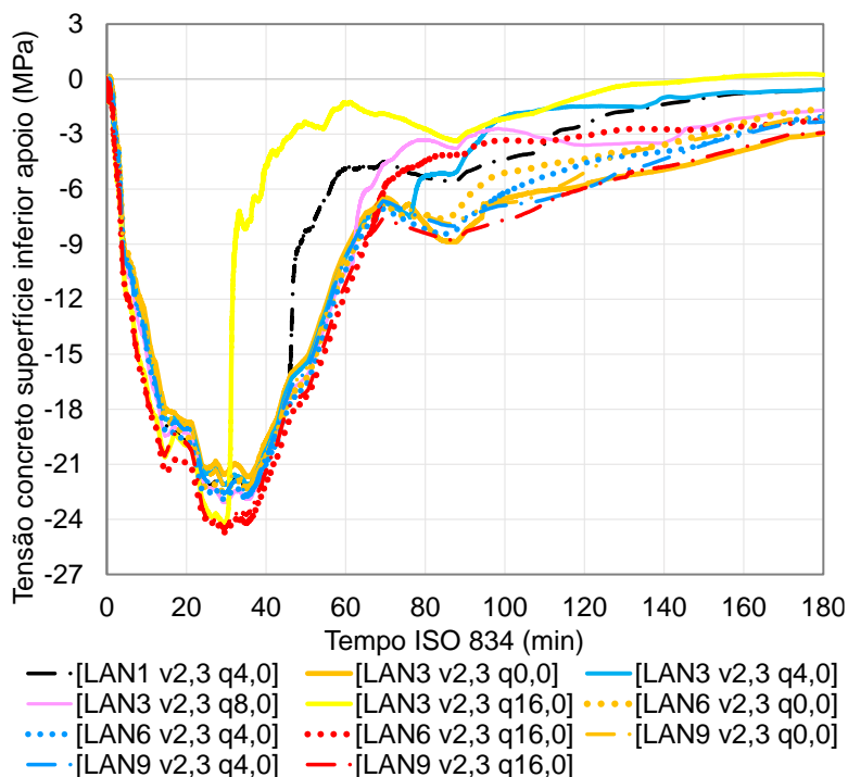
Figura 193 – Tensões no concreto, apoio intermediário (Co.4): vão 2,3 m
