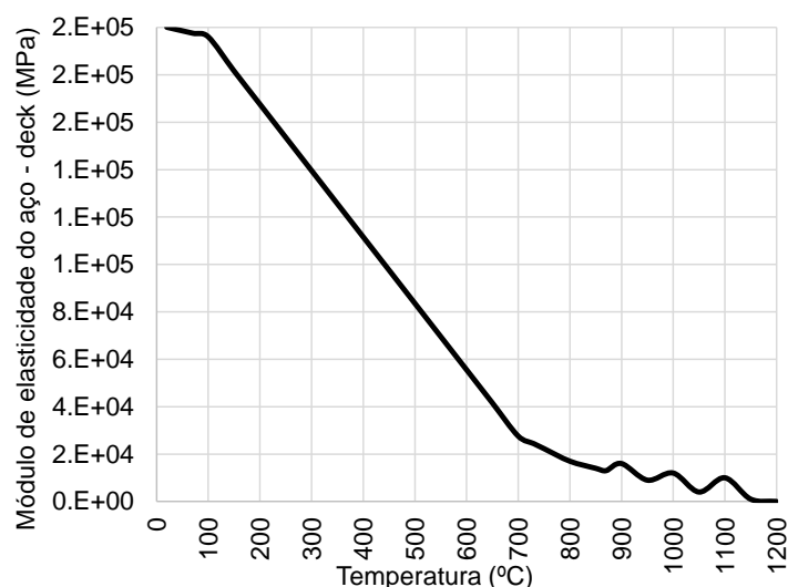
Figura 123 – Módulo elasticidade do aço da chapa: modelo numérico
