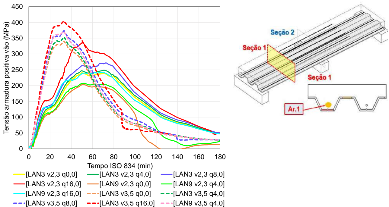
Figura 182 – Tensões produzidas nas armaduras positivas (Ar.1)
