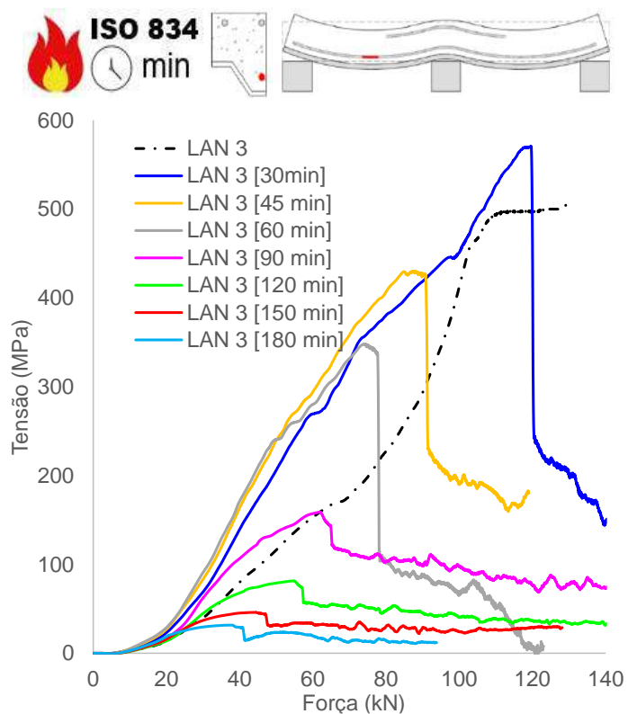
(c) Tensão armaduras positivas (vão)
