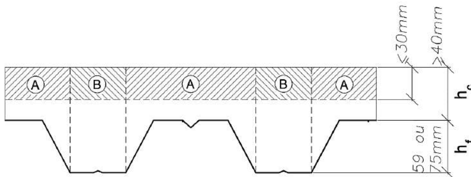
Figura 215 – Referência para determinação do fator C_f
