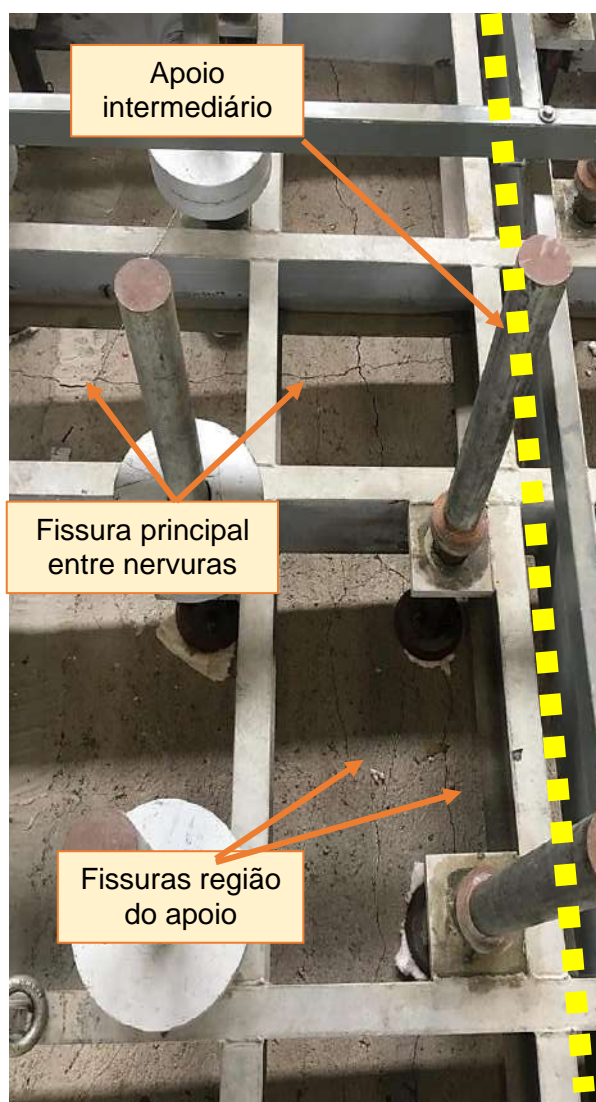
(c) respectivo registro em laboratório
