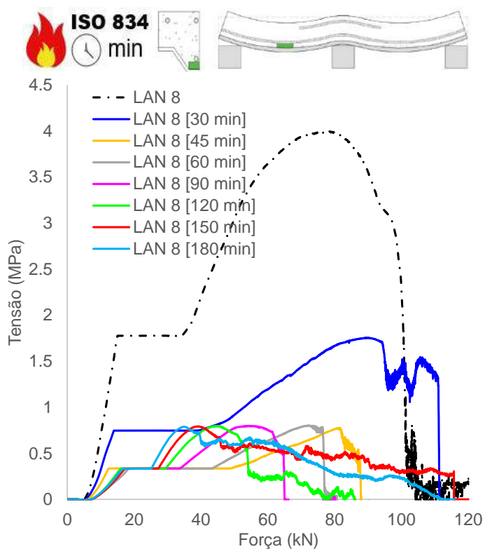
(m) Tensão concreto, adjacência mesa inferior chapa (vão)
