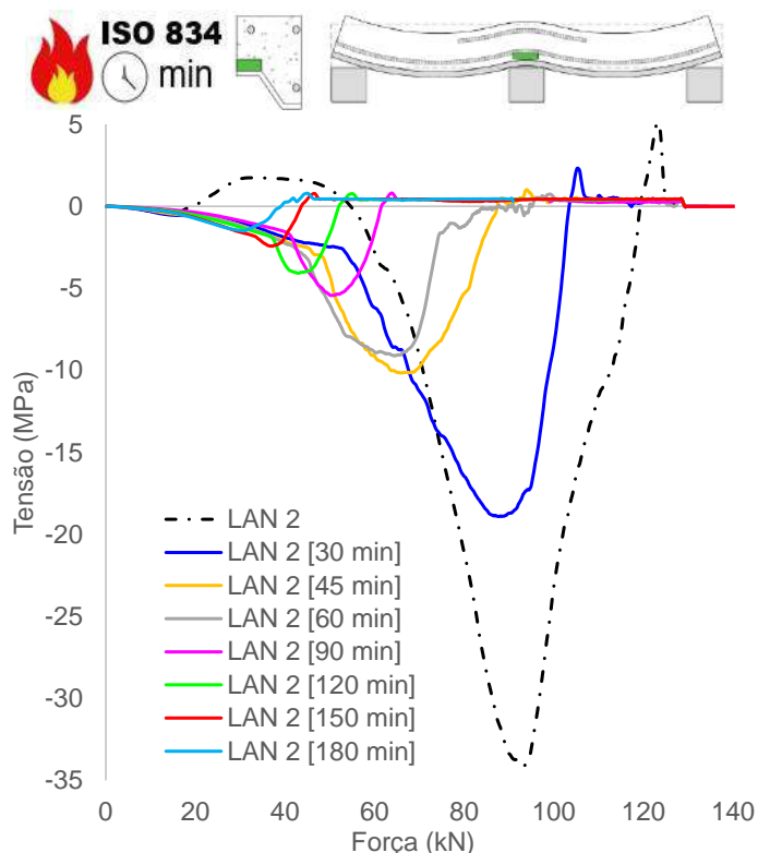
(k) Tensão concreto, adjacência mesa superior chapa (apoio)
