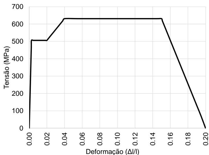
Figura 100 – Relação tensão vs deformação do aço das armaduras
