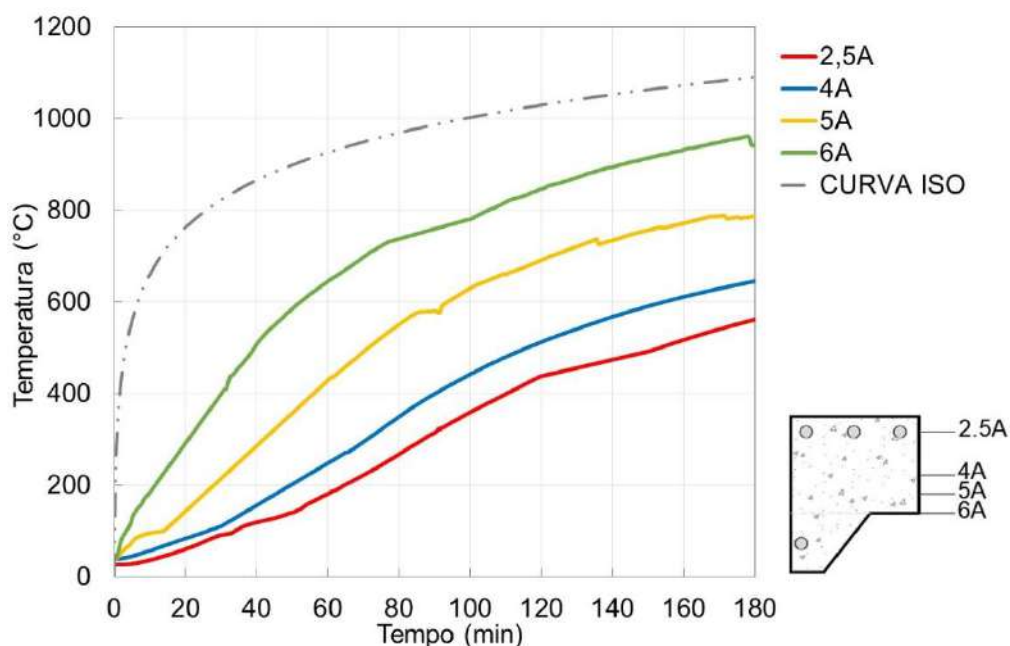
Figura 82 – Temperatura no concreto do alinhamento A da seção
