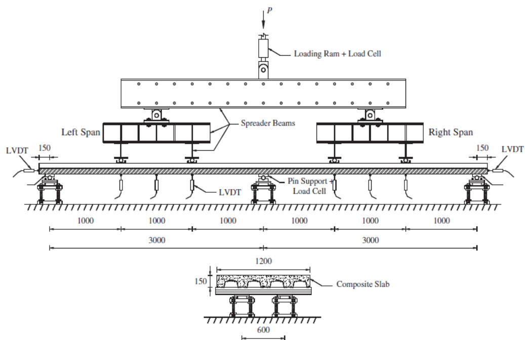
(a) Configuração do ensaio experimental
