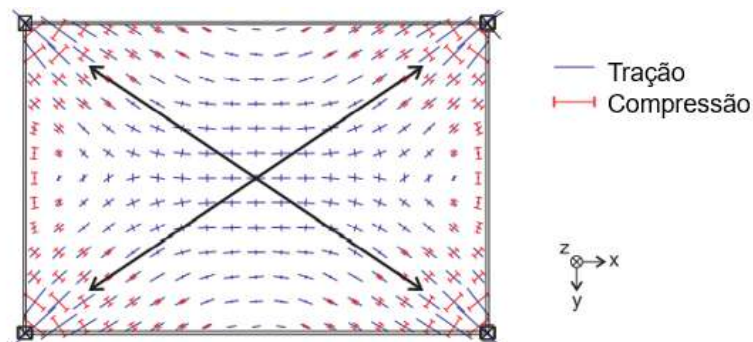
Figura 26 – Distribuição dos esforços e a mobilização do efeito de membrana Fonte: adaptado de Stadler (2012)
