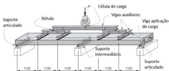
(b) Configuração do ensaio experimental
