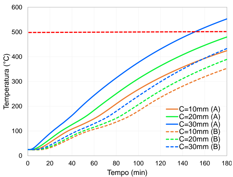
Figura 212 – Temperatura nas armaduras negativas, h_c=60\text{mm} e h_f=59\text{mm}
