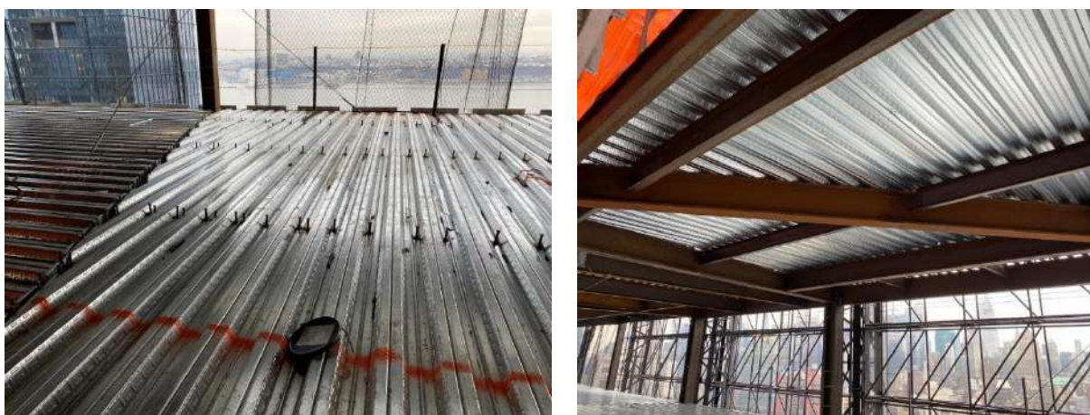
(a) Vista superior (antes da concretagem)
