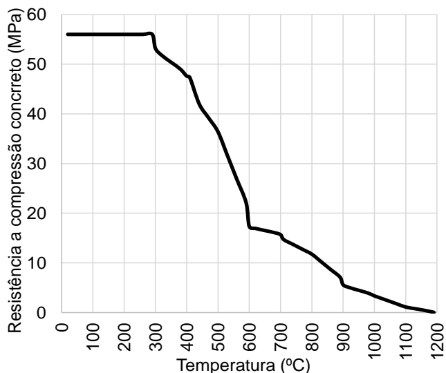
Figura 108 – Resistência a compressão do concreto: modelo numérico
