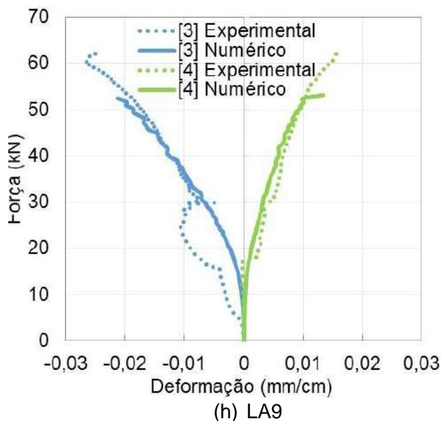
Figura 143 – Calibração alongamento da chapa junto ao apoio intermediário
