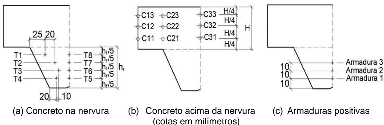
Figura 139 – Pontos de leitura das temperaturas na proposição das equações
