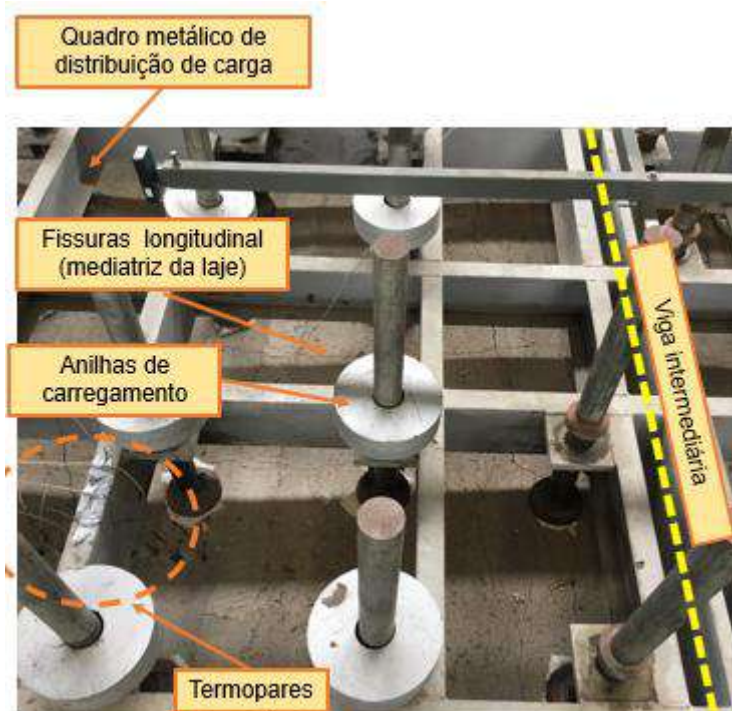
Figura 80 – Fissura longitudinal
