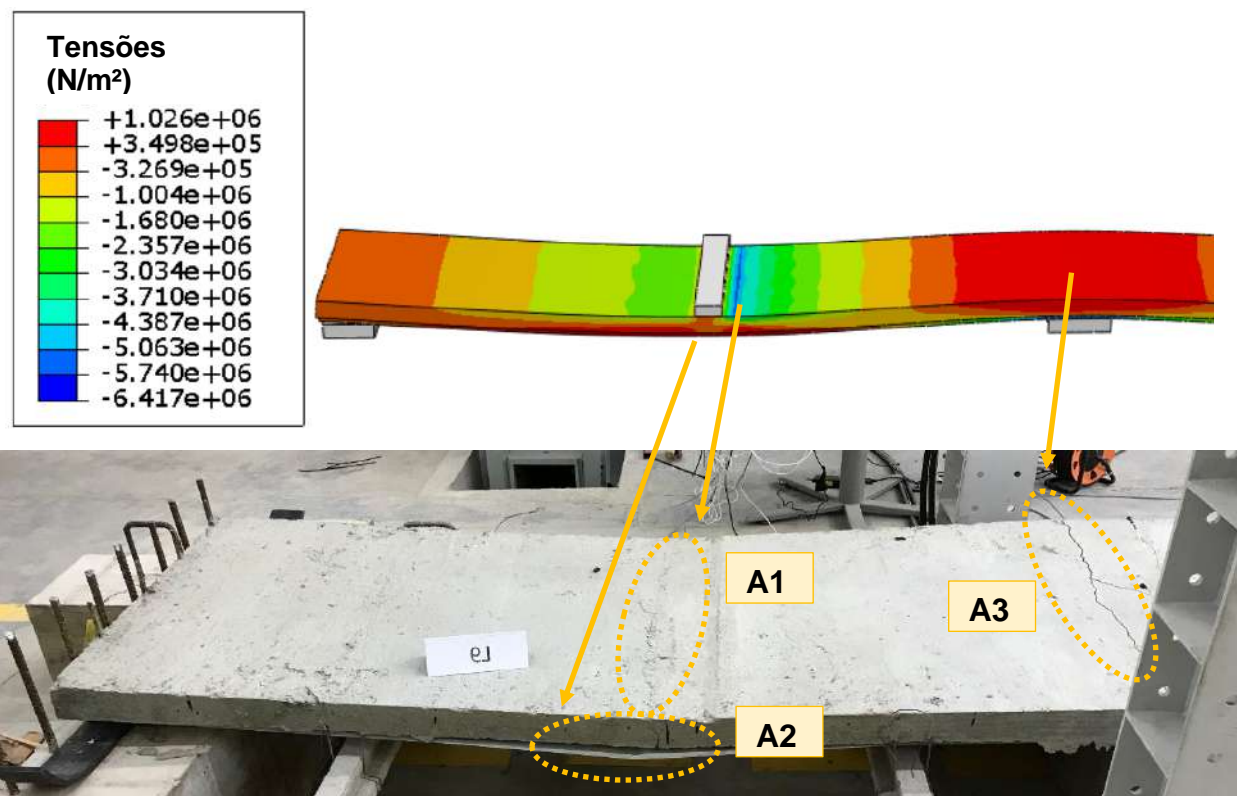
Figura 149 – Comparativo esforços no concreto
