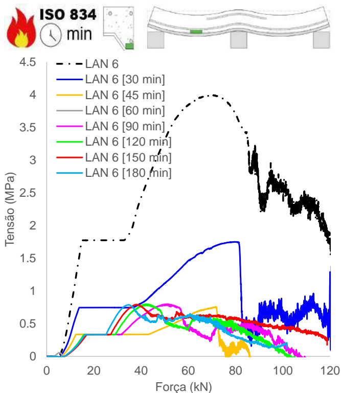
(k) Tensão concreto, adjacência mesa inferior chapa (vão)
