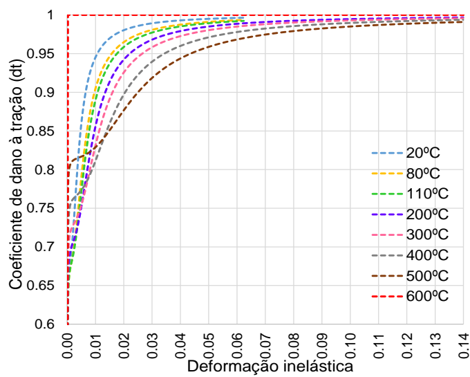
Figura 117 – Coeficiente de dano ao concreto tracionado: modelo numérico
