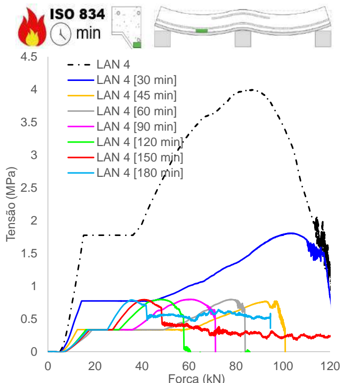
(l) Tensão concreto, adjacência mesa inferior chapa (vão)
