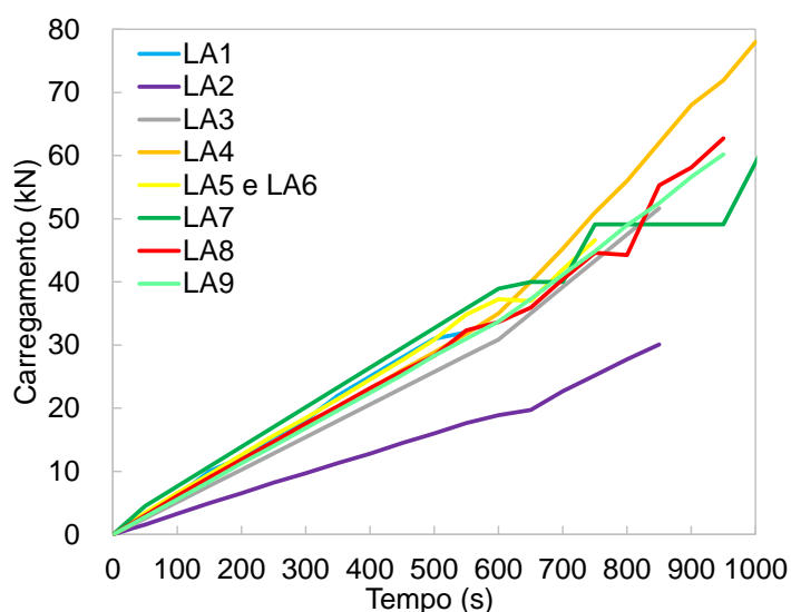
Figura 63 – Carregamento vs tempo: análises numéricas e experimentais
