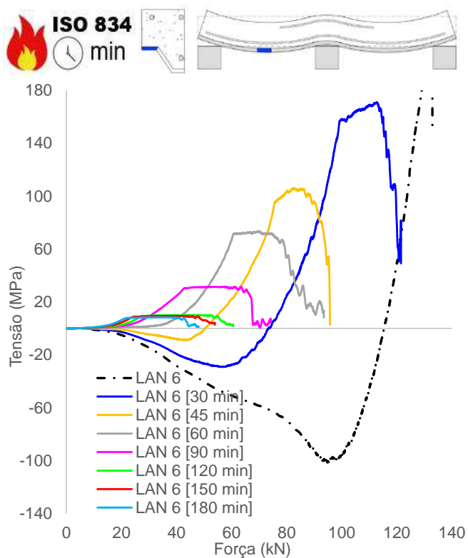
(c) Tensão chapa, mesa superior (vão)
