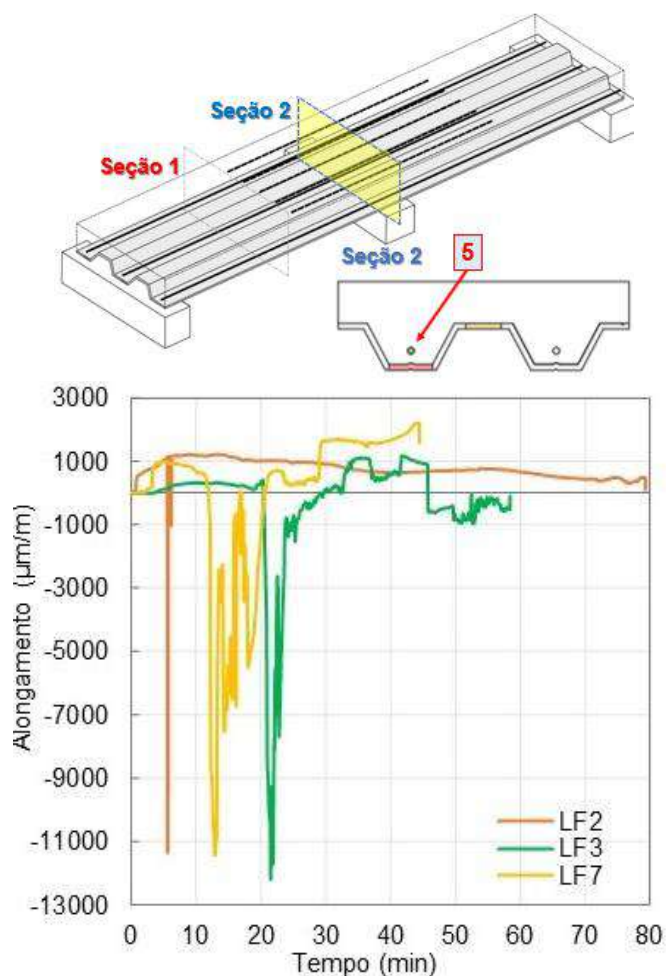
Figura 89 – Deformação longitudinal armaduras positivas
