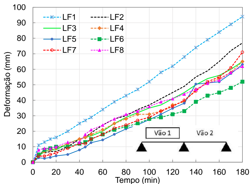
Figura 91 – Deformações (flechas) no vão 1 das lajes avaliadas em laboratório
