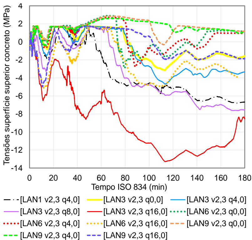
Figura 190 – Tensões no concreto, meio do vão (Co.2): vão 2,3 m
