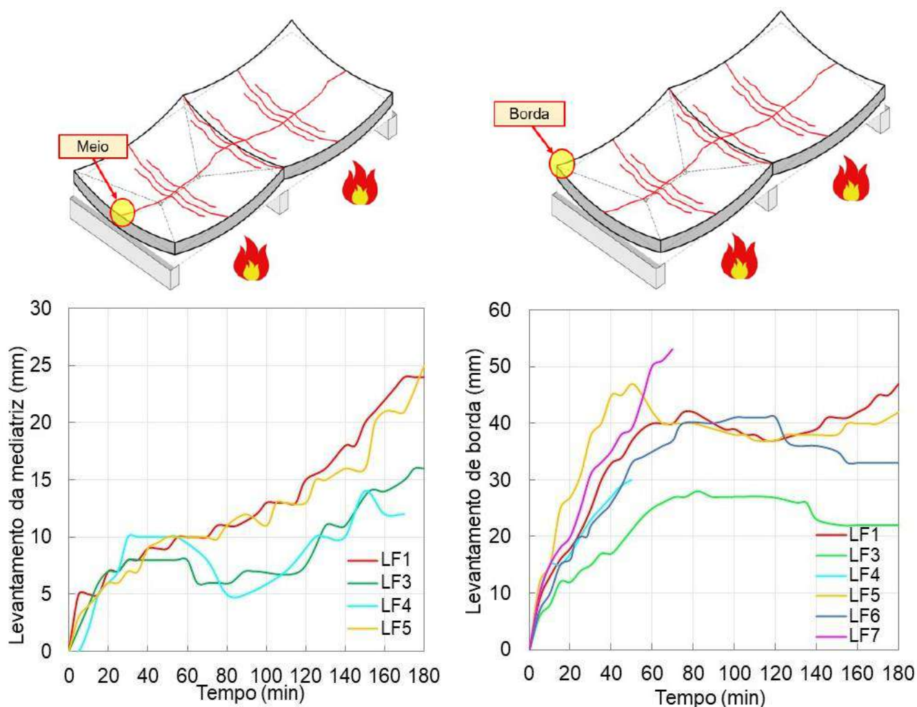
Figura 94 – Levantamento mediatriz (meio) das lajes avaliadas em laboratório
