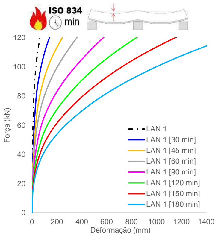
(a) Deformações verticais (flechas)
