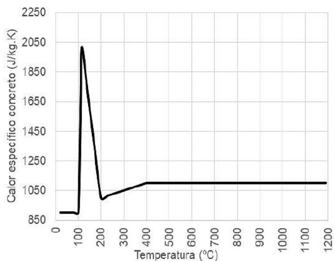
Figura 102 – Calor específico do concreto: modelo numérico
