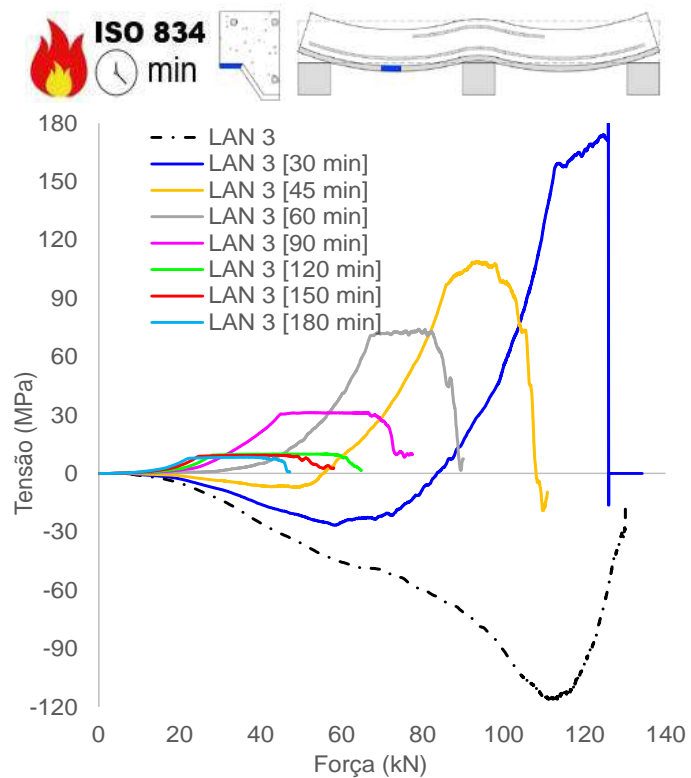
(e) Tensão chapa, mesa superior (vão)
