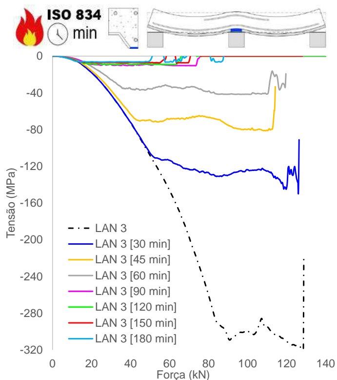
(g) Tensão chapa, mesa inferior (apoio)
