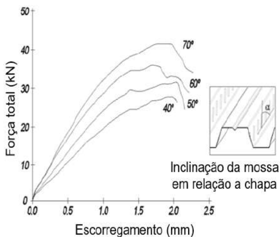
(c) inclinação da mocha em relação a chapa perfilada
