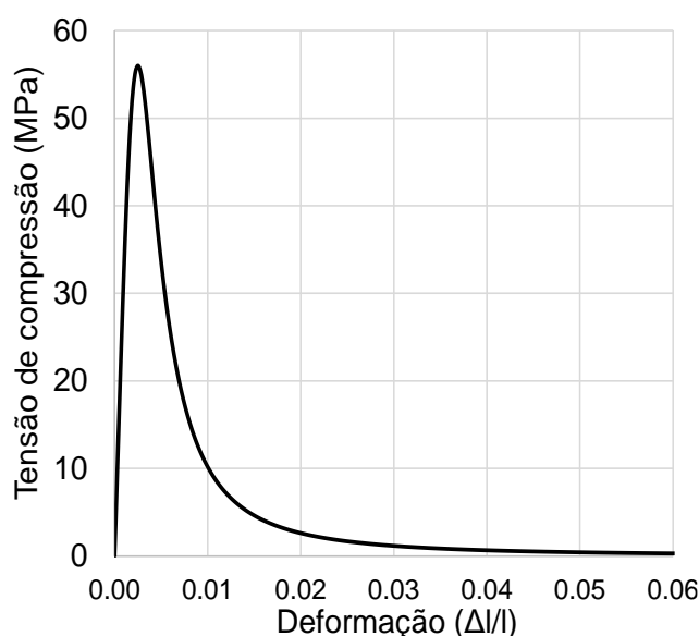
Figura 97 – Relação tensão-deformação do concreto à compressão
