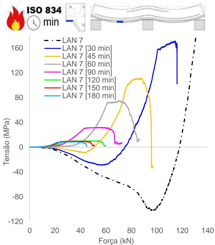
(c) Tensão chapa, mesa superior (vão)
