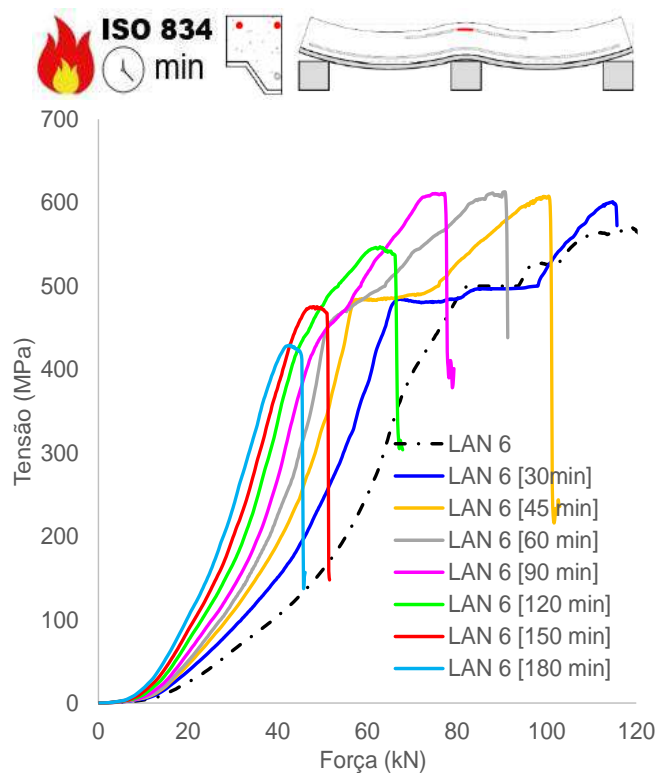
(b) Tensão armaduras negativas (apoio)
