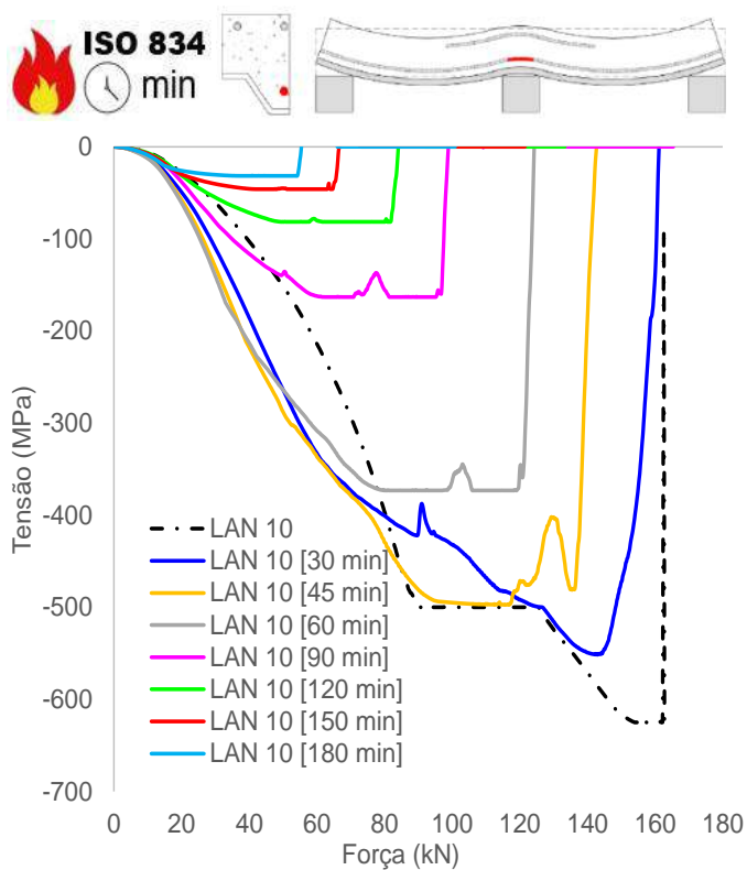
(c) Tensão armaduras positivas (apoio)
