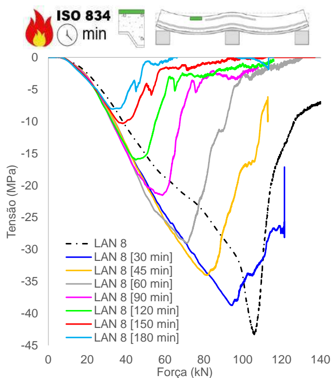
(l) Tensão concreto, superfície superior (vão)
