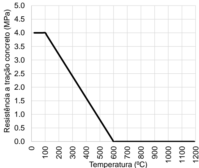
Figura 109 – Resistência a tração do concreto: modelo numérico
