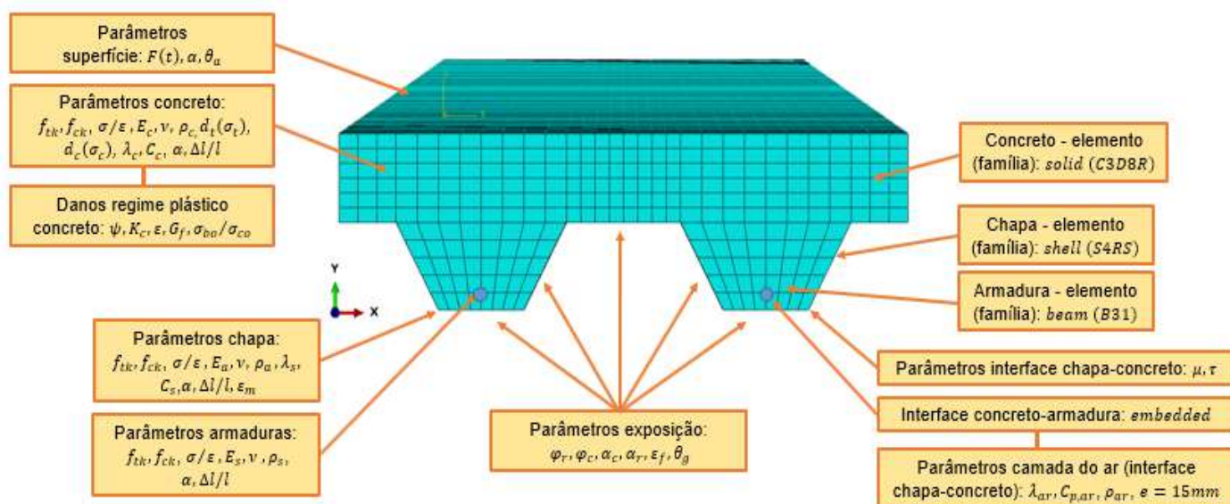
Figura 134 – Modelo de cálculo: análise numérica - parâmetros termomecânicos
