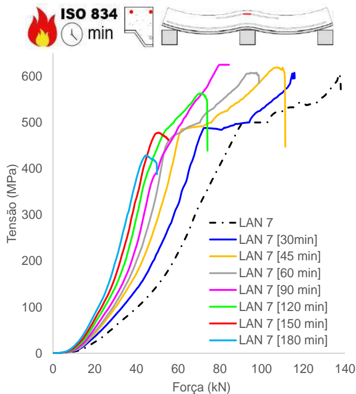
(b) Tensão armaduras negativas (apoio)
