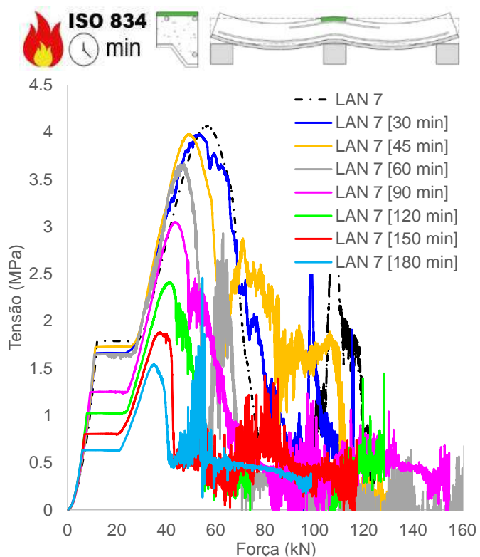
(g) Tensão concreto, superfície superior (apoio)
