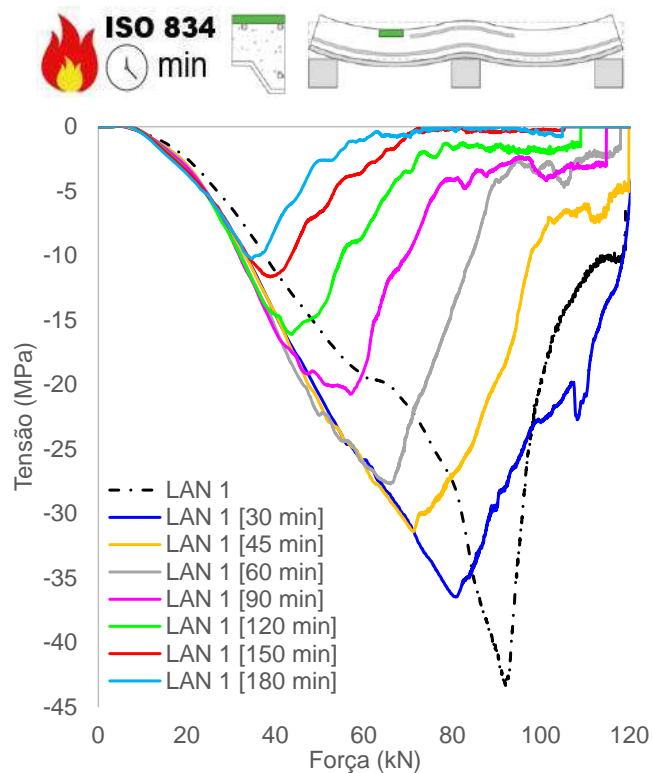
(b) Tensão concreto, superfície superior (vão)
