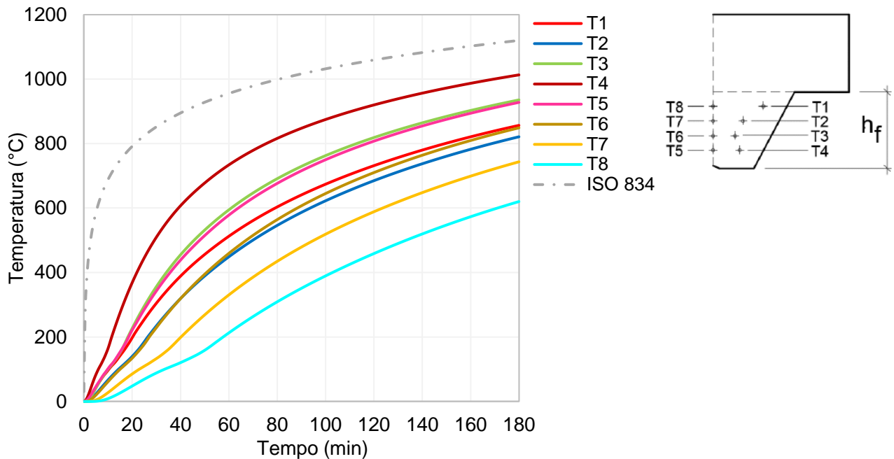
Figura 206 – Temperatura no concreto na nervura, laje com h_f = 75\text{mm}
