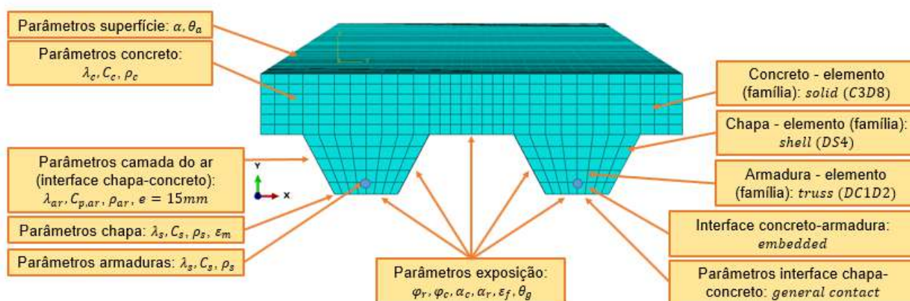
Figura 130 – Modelo de cálculo: análise numérica - parâmetros térmicos
