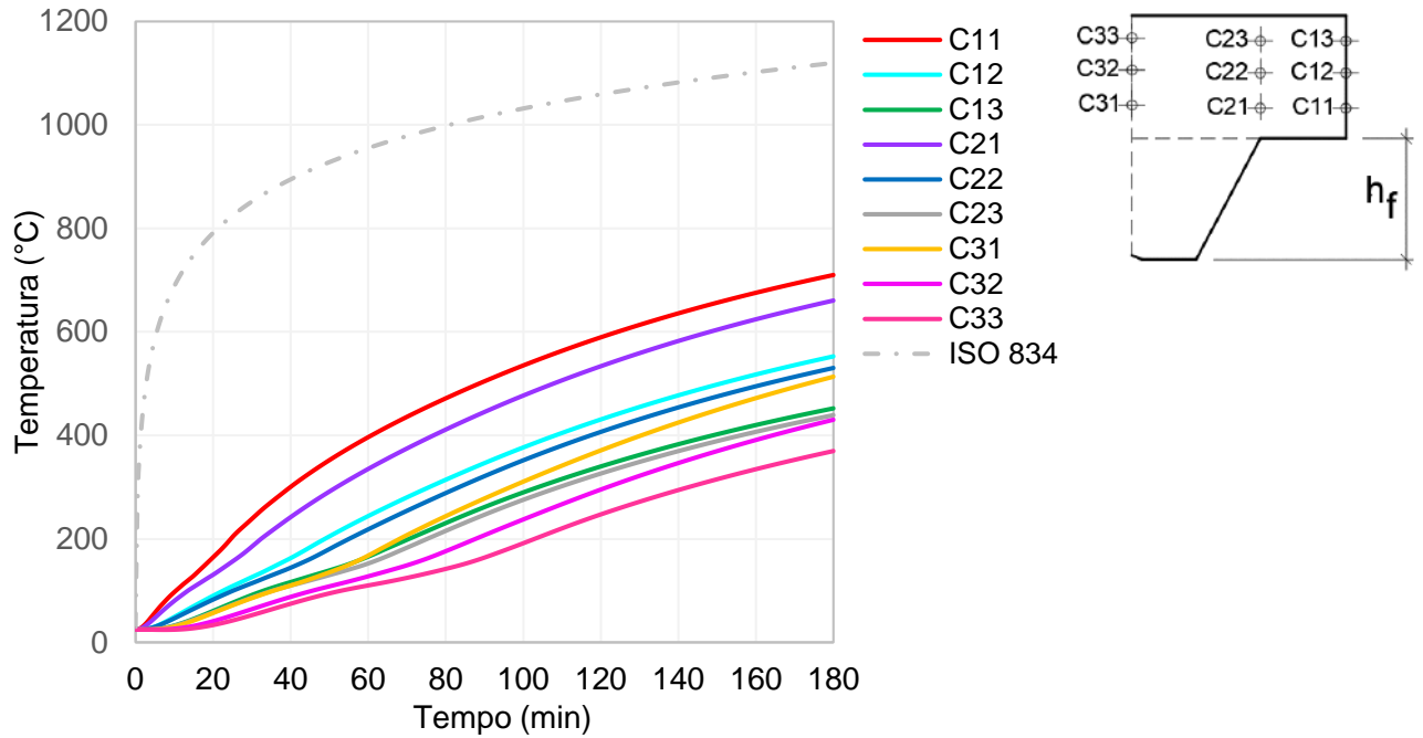
Figura 205 – Temperatura no concreto acima na nervura, laje com h_f = 59\text{mm}
