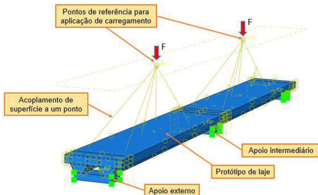
Figura 135 – Modelo de cálculo: análises termomecânicas (modelo 3b)
