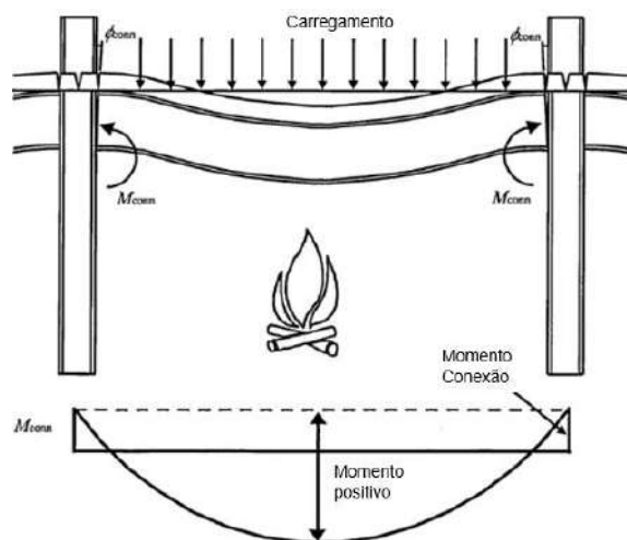
Figura 20 – Momento negativo desenvolvido na restrição à dilatação térmica Javaheriaif (2017)
