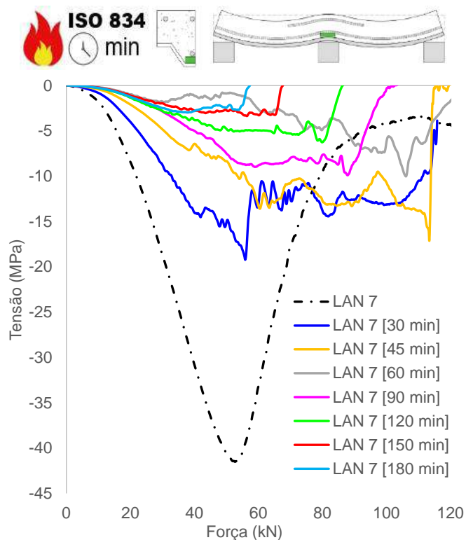
(h) Tensão concreto, adjacência mesa inferior chapa (apoio)
