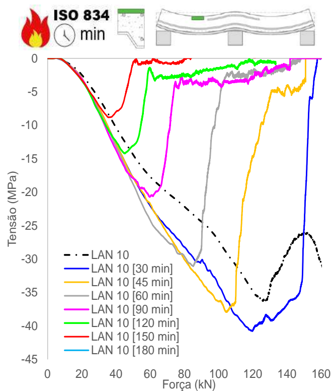
(l) Tensão concreto, superfície superior (vão)
