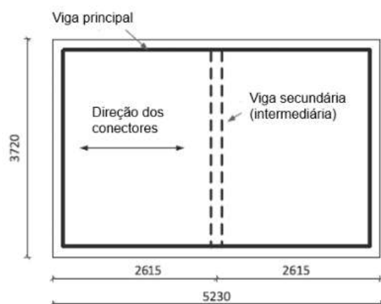
(a) Configuração do protótipo de laje
