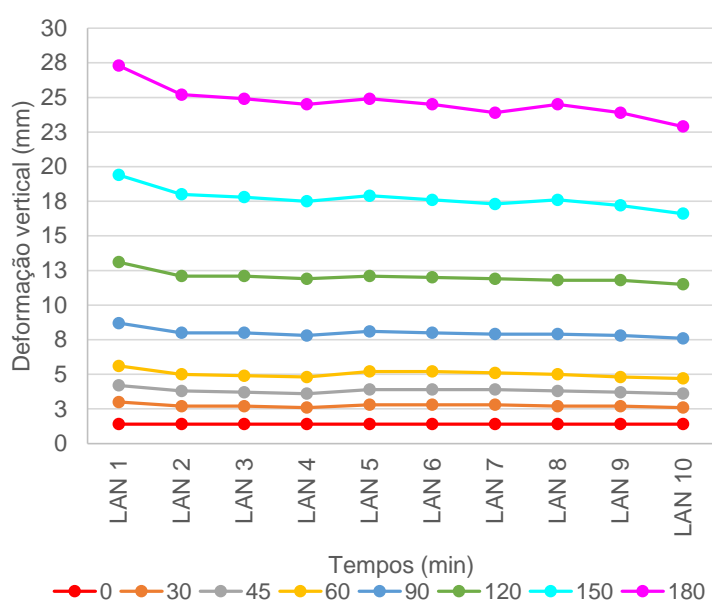
(a) Força aplicada de 25 kN
