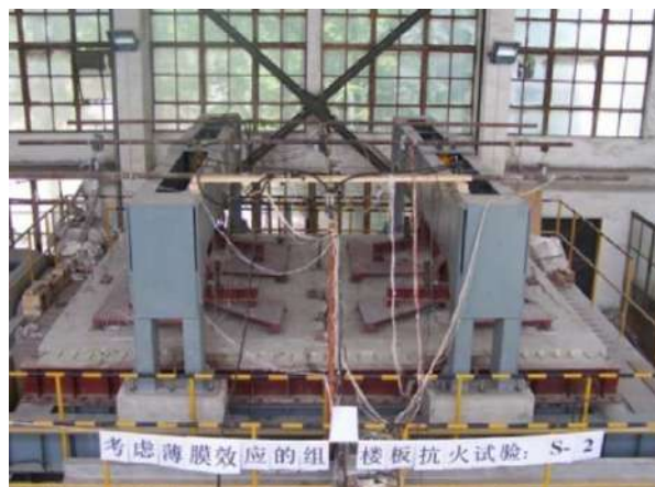
(b) Configuração do ensaio experimental
