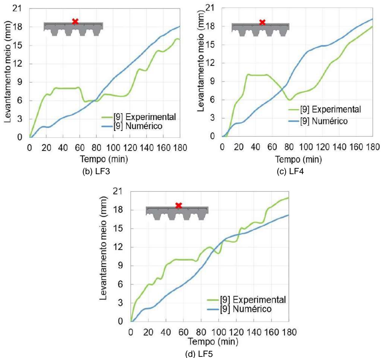
Figura 156 – Calibração da deformação da mediatriz
