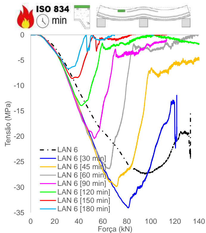
(j) Tensão concreto, superfície superior (vão)
