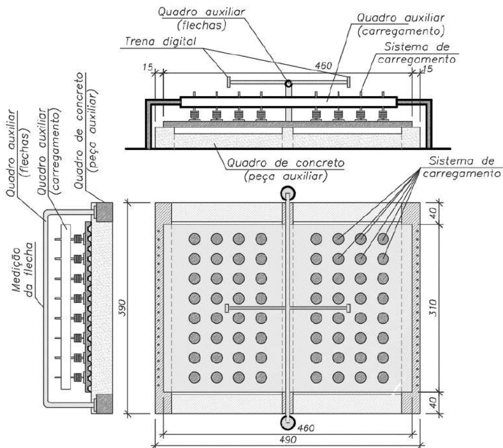
Figura 51 – Esquema do ensaio de laje mista contínua para análise da LF
