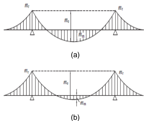
Figura 21 – Redistribuição dos momentos: (a) antes e (b) durante aquecimento Guo (2012)
