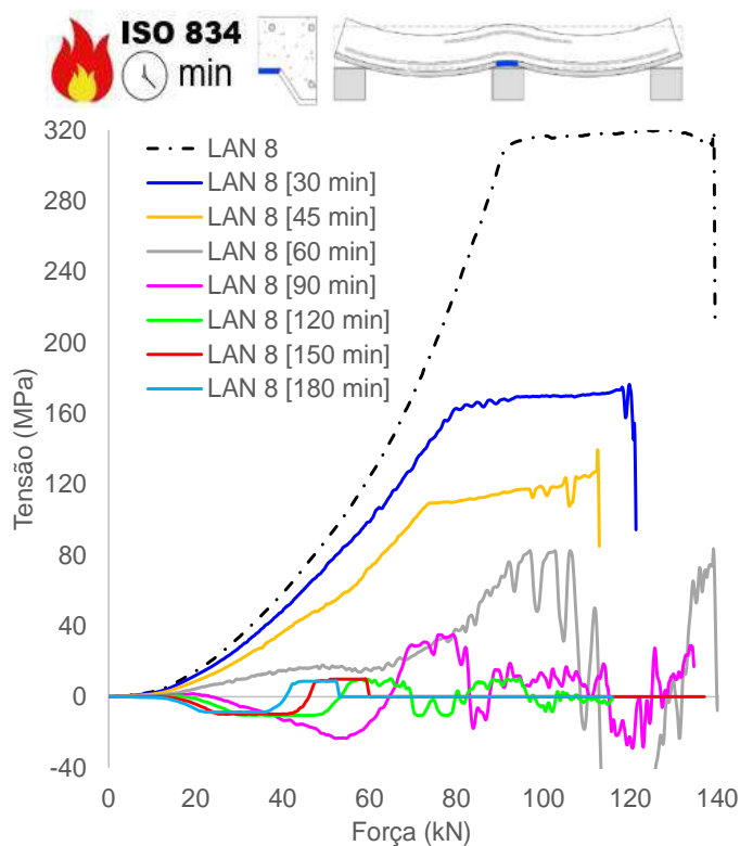
(g) Tensão chapa, mesa superior (apoio)
