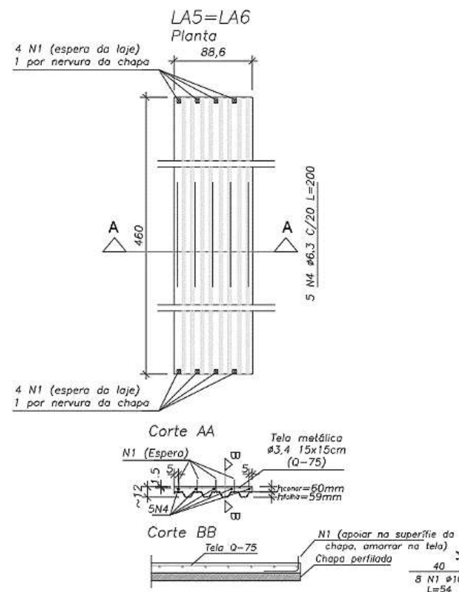
(d) LA5 e LA6
