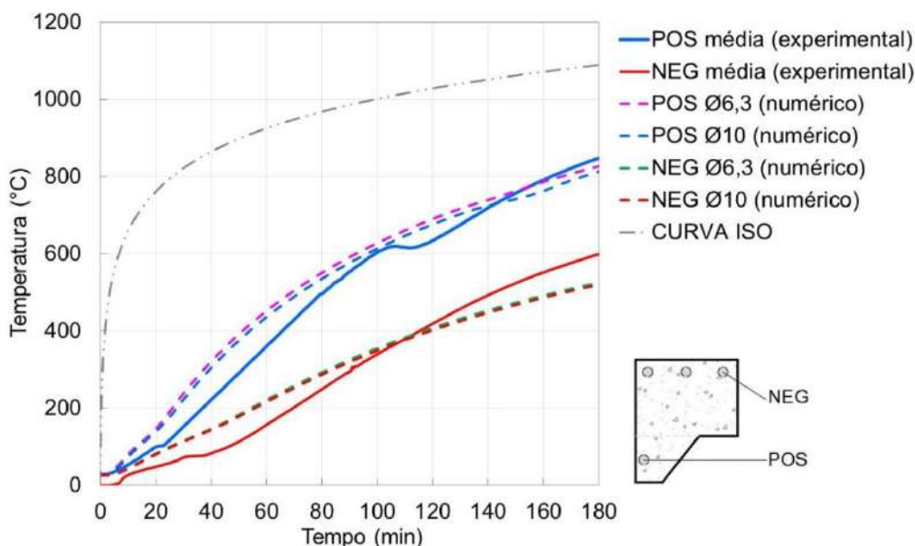
Figura 153 – Calibração das temperaturas nas armaduras
