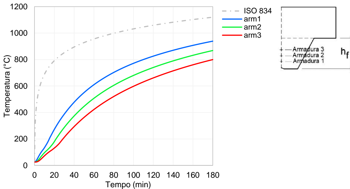
Figura 208 – Temperatura nas armaduras positivas, laje com h_f = 59\text{mm}
