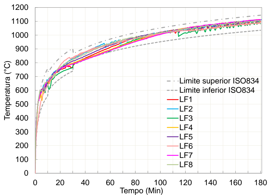
Figura 75 – Curva de temperatura do forno horizontal: ensaio lajes LF1 a LF8
