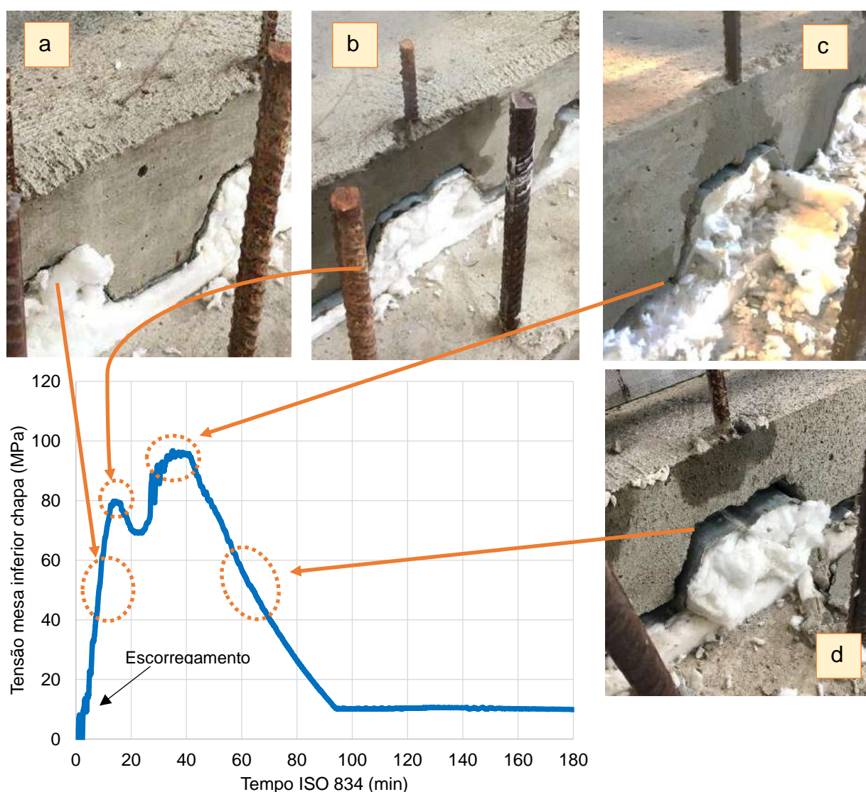
Figura 160 – Calibração do desprendimento da chapa
