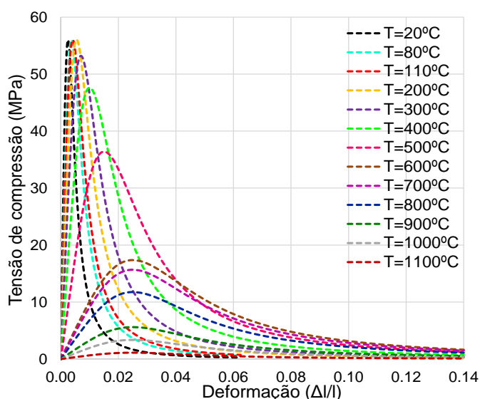
Figura 110 – Diagrama tensão-deformação do concreto: modelo numérico
