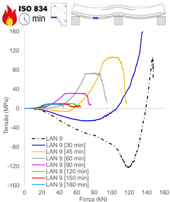
(e) Tensão chapa, mesa superior (vão)
