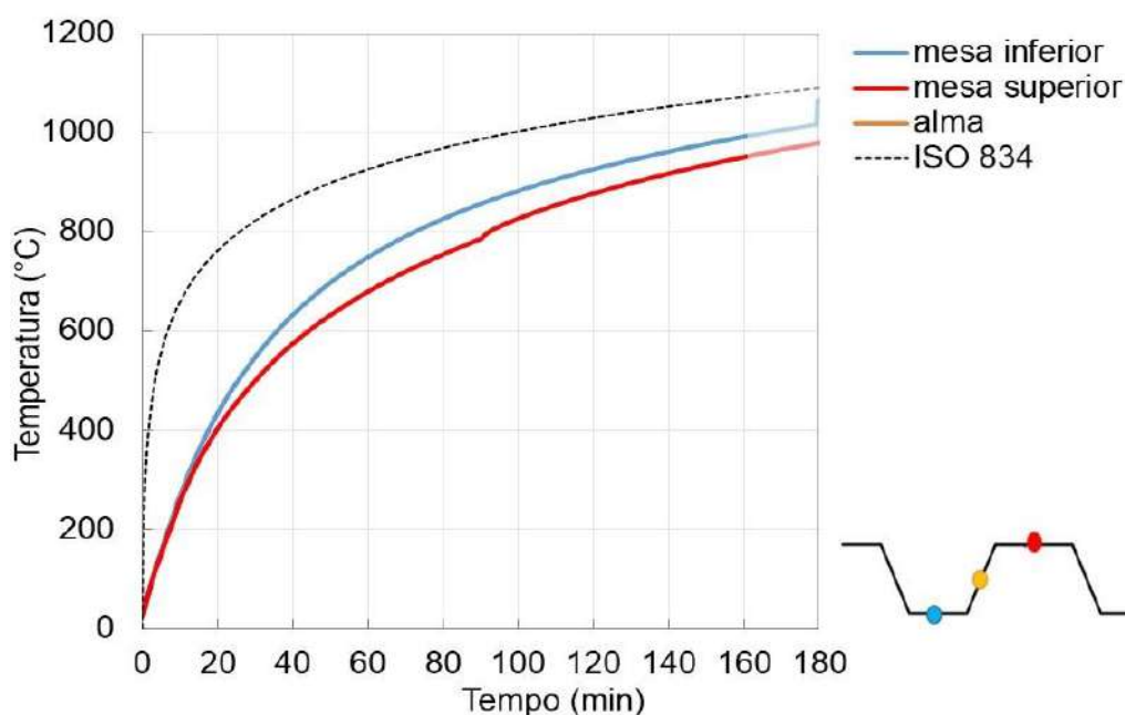
Figura 85 – Temperatura mesa inferior e superior da chapa perfilada
