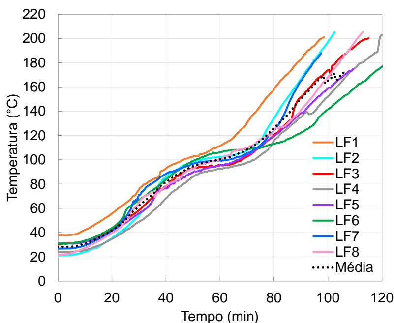
Figura 88 – Isolamento térmico das lajes experimentalmente avaliadas
