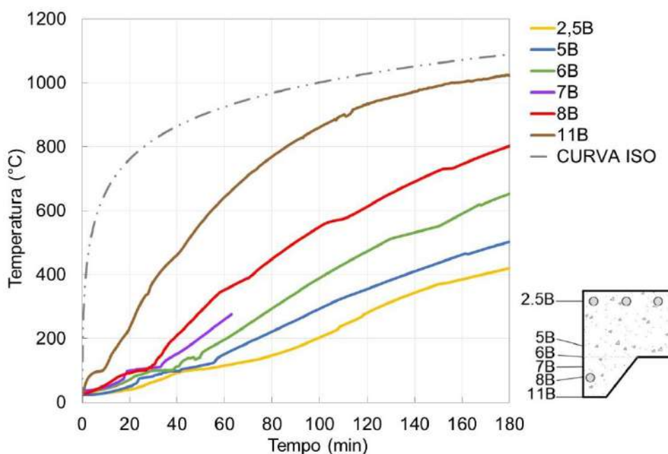
Figura 83 – Temperatura no concreto do alinhamento B da seção
