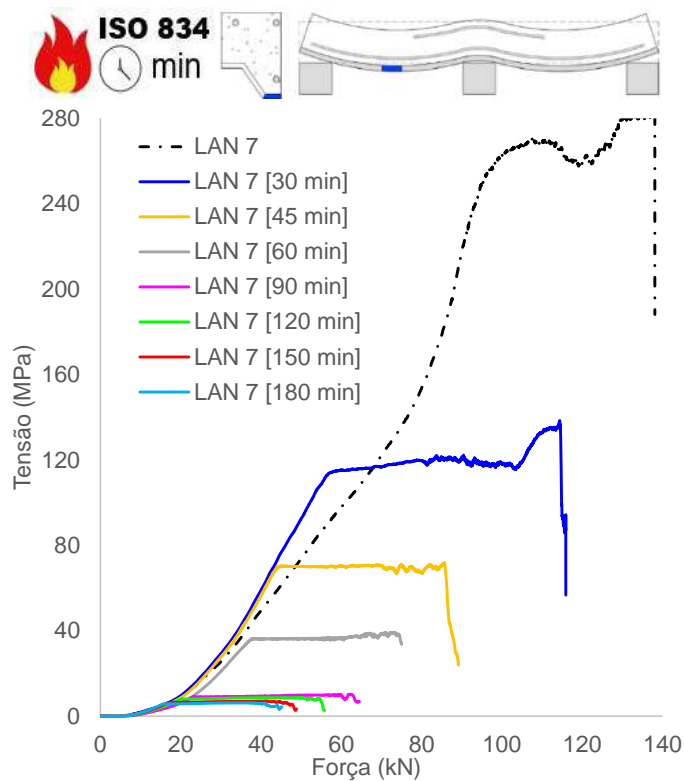
(d) Tensão chapa, mesa inferior (vão)
