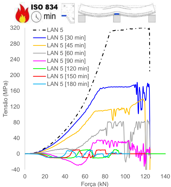
(e) Tensão chapa, mesa superior (apoio)
