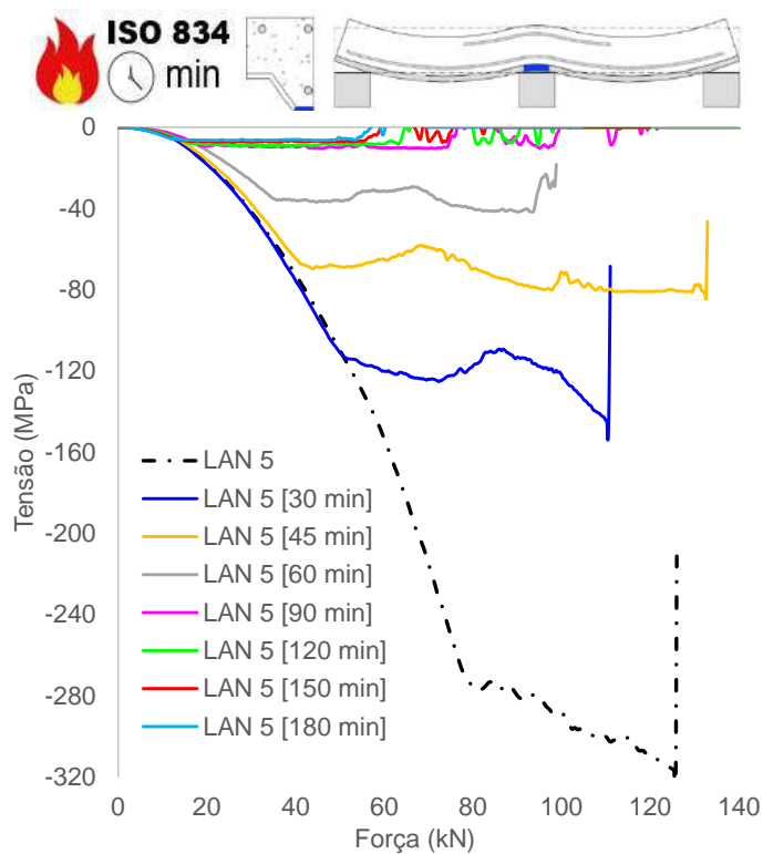
(f) Tensão chapa, mesa inferior (apoio)
