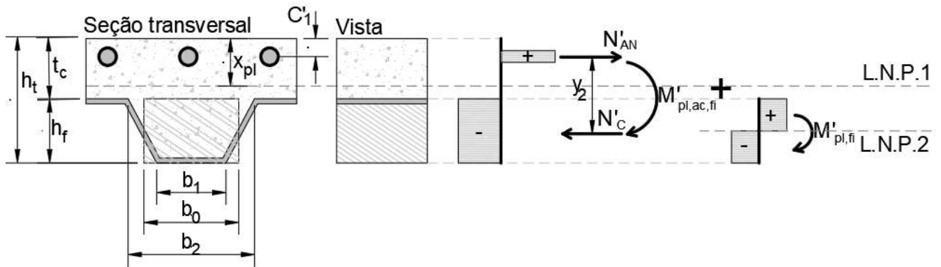
Figura 200 – Momento resistente negativo: armaduras negativas (caso I)
