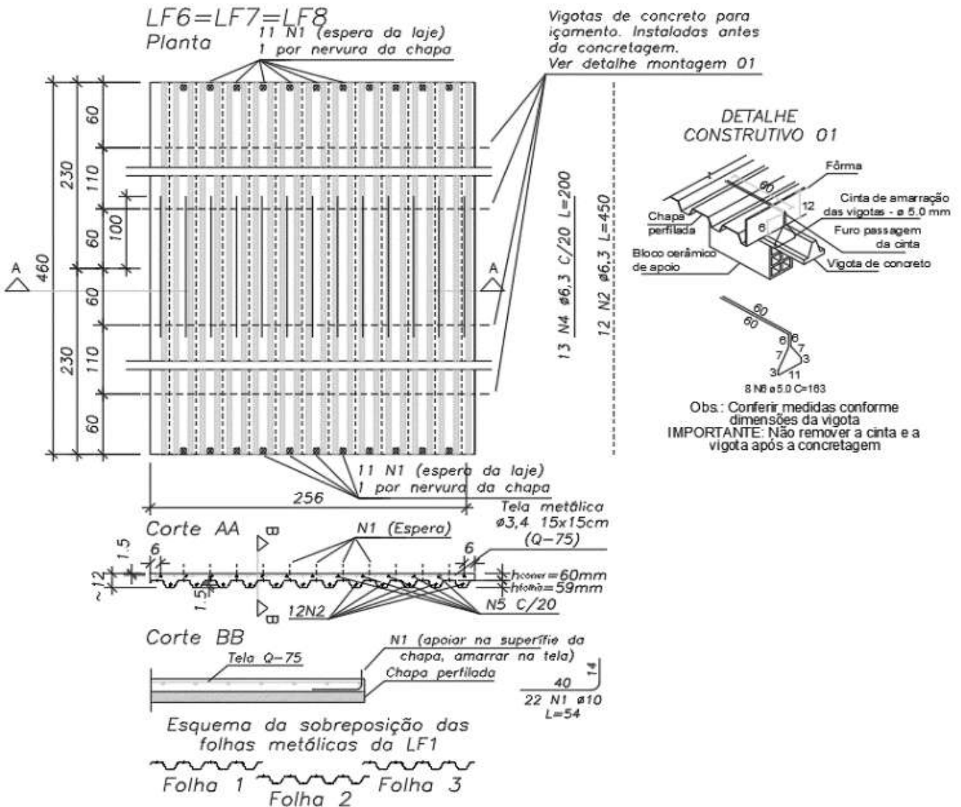
Figura 46 – Detalhamento estrutural da LF6, LF7 e LF8
