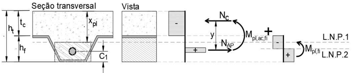
Figura 199 – Momento resistente positivo: armaduras positivas (caso II)
