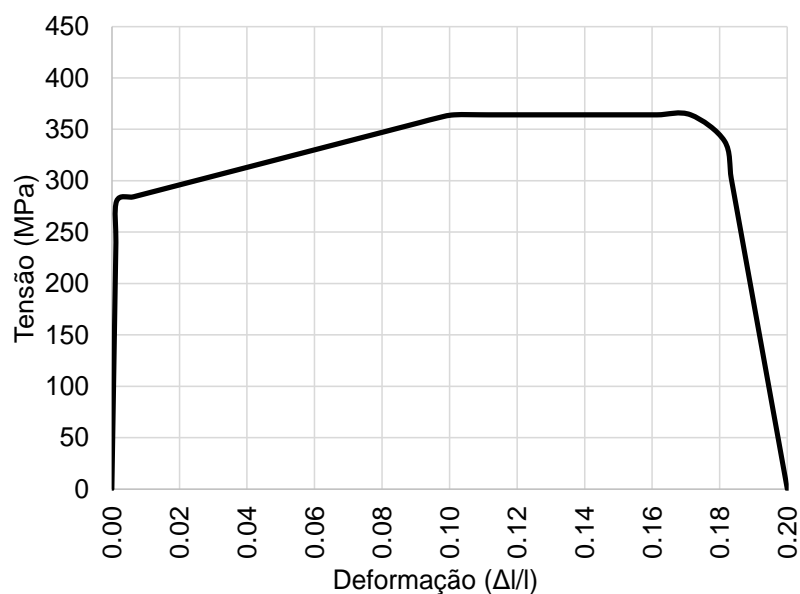
Figura 101 – Relação tensão vs deformação do aço da chapa
