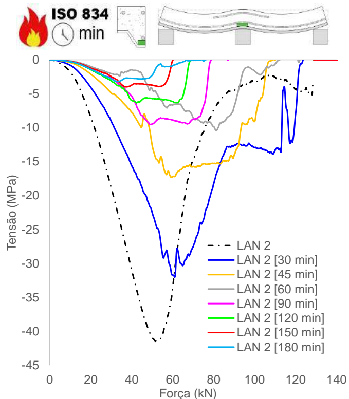
(j) Tensão concreto, adjacência mesa inferior chapa (apoio)
