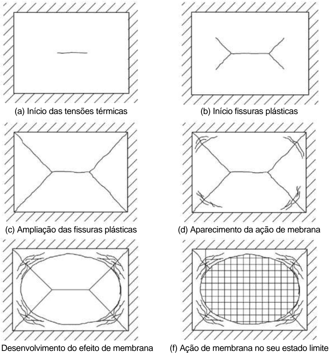
Figura 27 – O desenvolvimento da ação de membrana em laje mista
