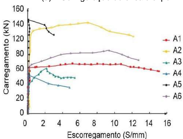
(c) Lajes com vão de 450 mm
