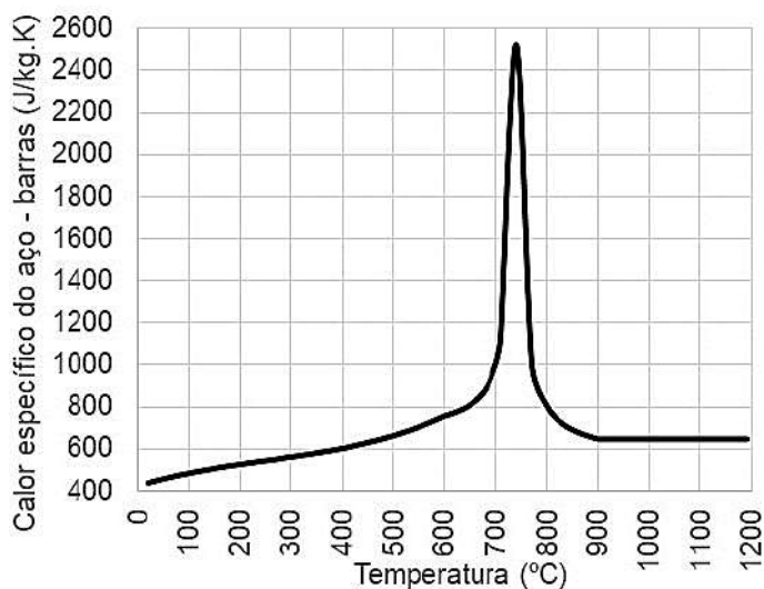
Figura 105 – Calor específico do aço CA-50: modelo numérico
