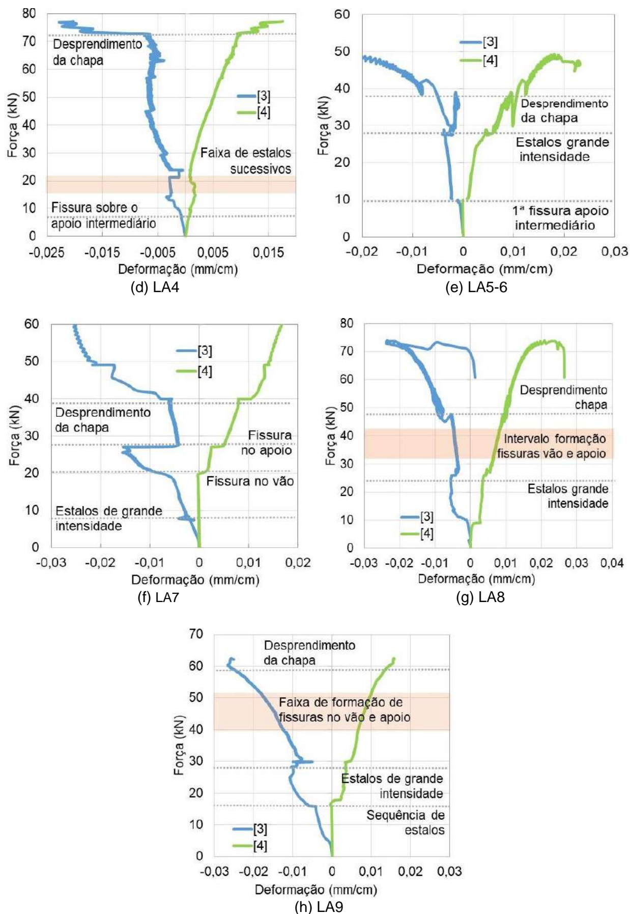
Figura 66 – Alongamento da chapa junto ao apoio: modelo experimental
