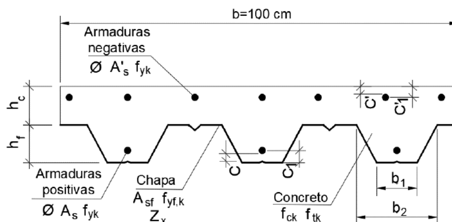
Figura 237 – Convenção das aplicações dos métodos de cálculo propostos
