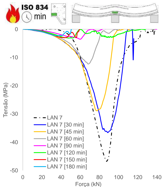
(i) Tensão concreto, adjacência mesa superior chapa (apoio)
