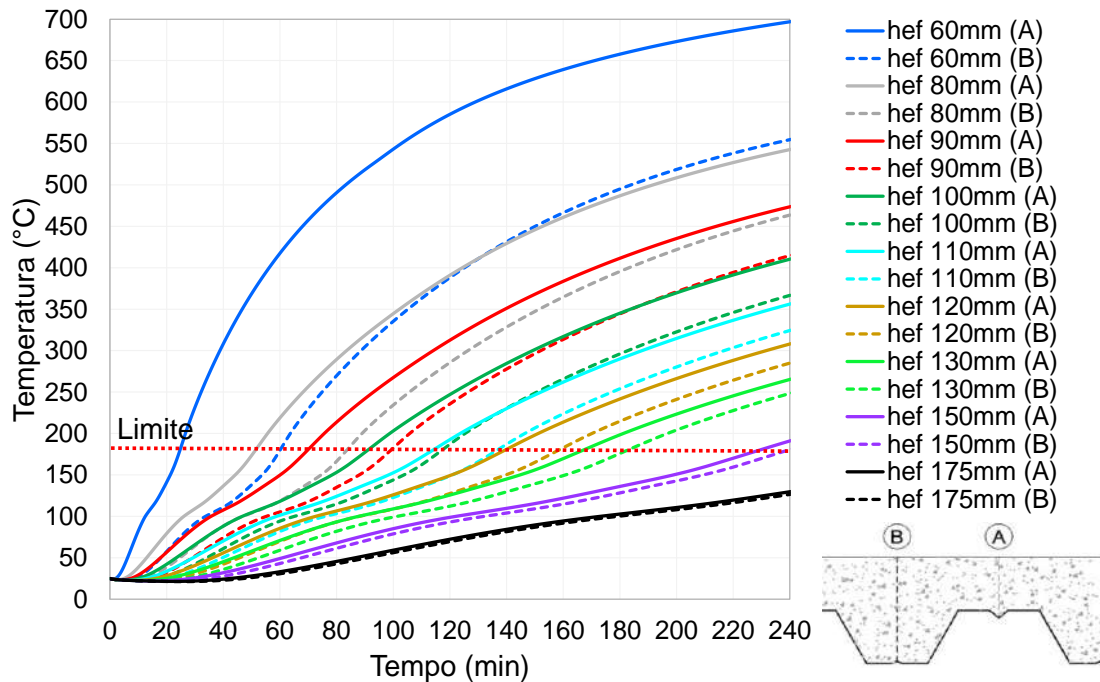
Figura 219 – Isolamento térmico: temperaturas pontuais (ponto A ou B)
