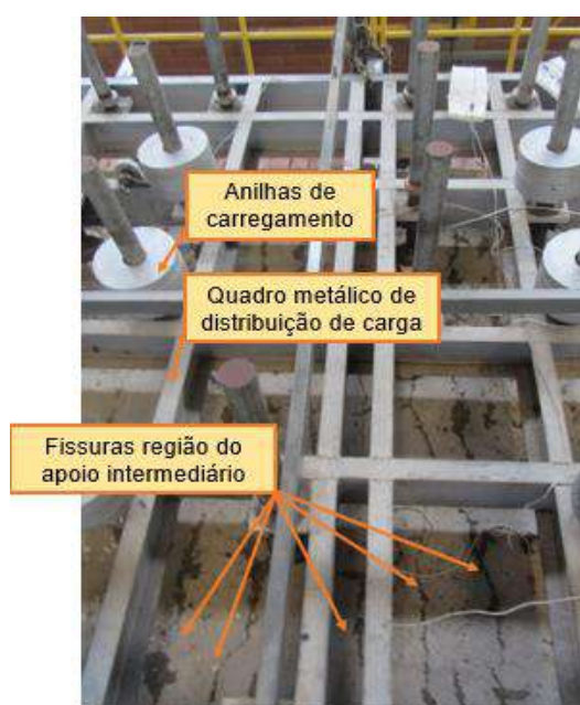
Figura 77 – Fissuras na laje na região do apoio intermediário
