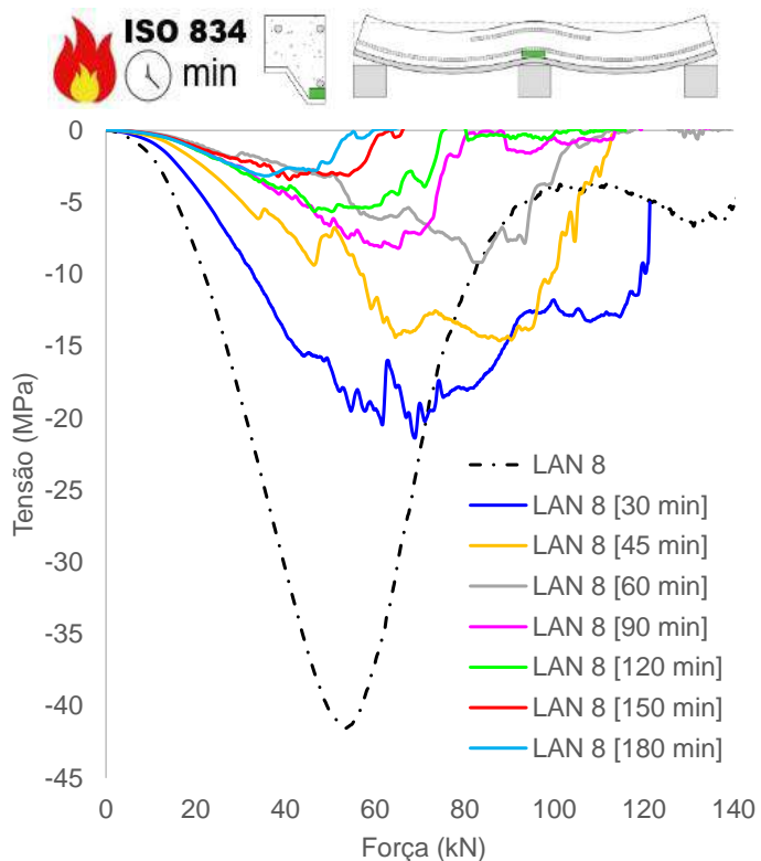
(j) Tensão concreto, adjacência mesa inferior chapa (apoio)
