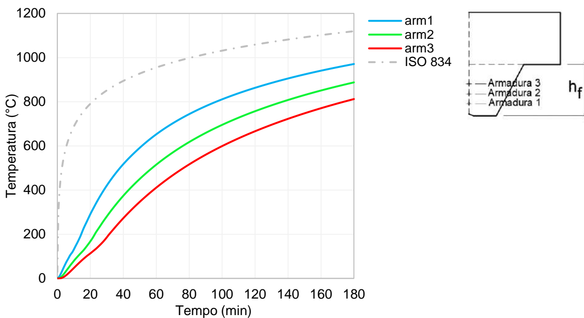
Figura 209 – Temperatura nas armaduras positivas, laje com h_f = 75\text{mm}
