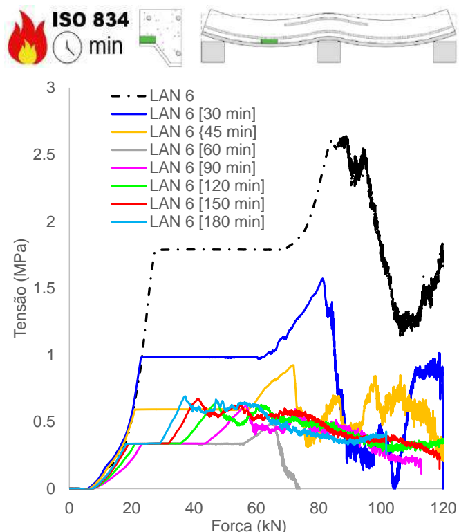
(l) Tensão concreto, adjacência mesa superior chapa (vão)
