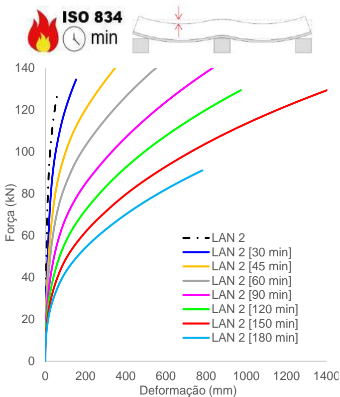
(a) Deformações verticais (flechas)
