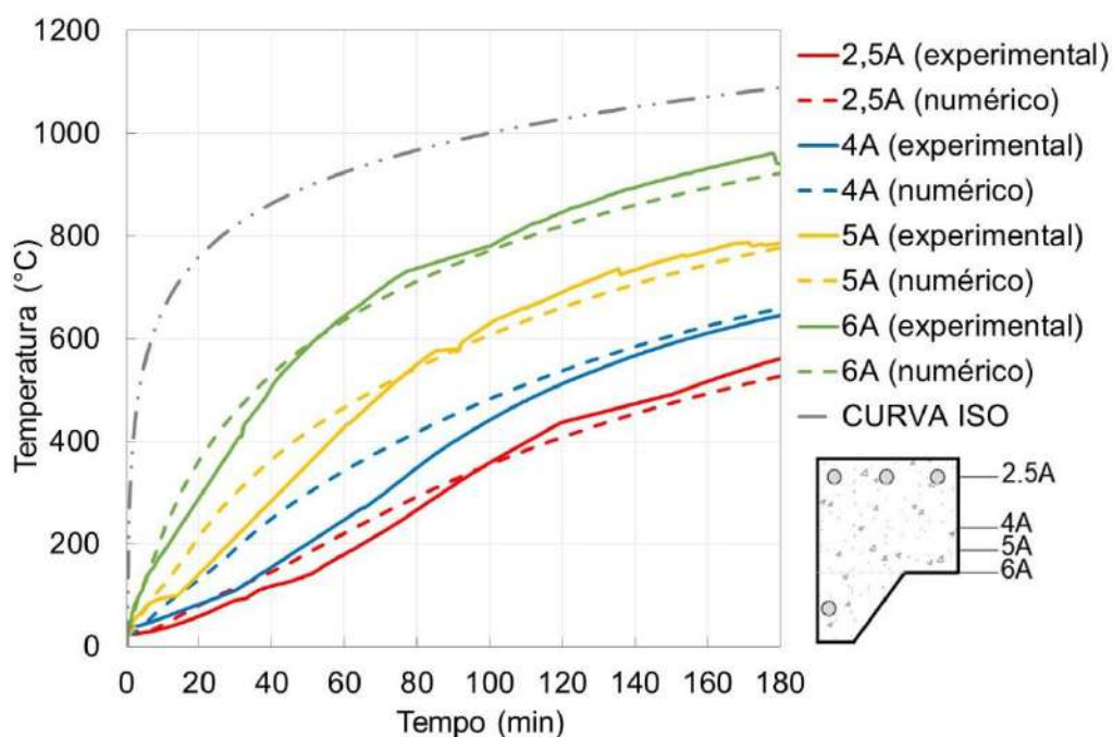
Figura 151 – Calibração das isotermas: alinhamento A da seção
