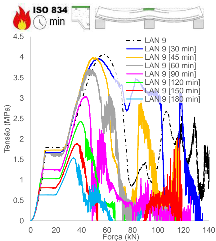
(i) Tensão concreto, superfície superior (apoio)
