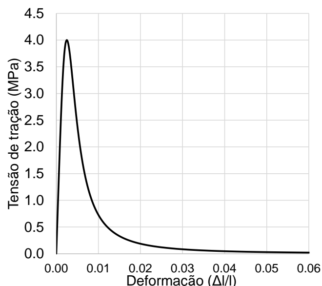
Figura 98 – Relação tensão-deformação do concreto à tração
