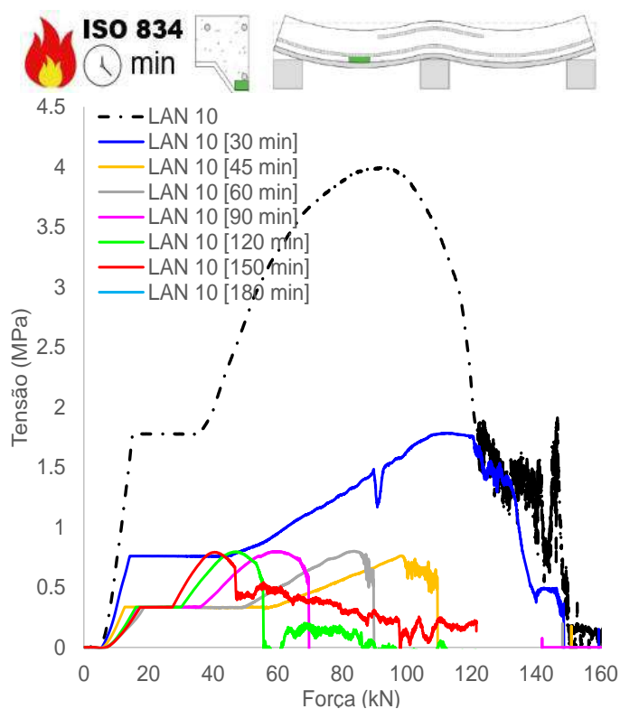
(m) Tensão concreto, adjacência mesa inferior chapa (vão)
