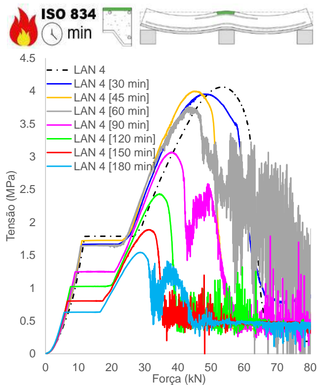
(i) Tensão concreto, superfície superior (apoio)
