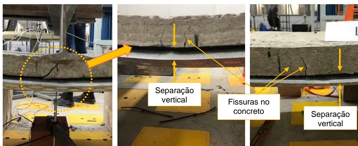
(a) LA1 (b) LA4 (c) LA9 Figura 71 – Fissuras no meio do vão, no ponto de aplicação do carregamento
