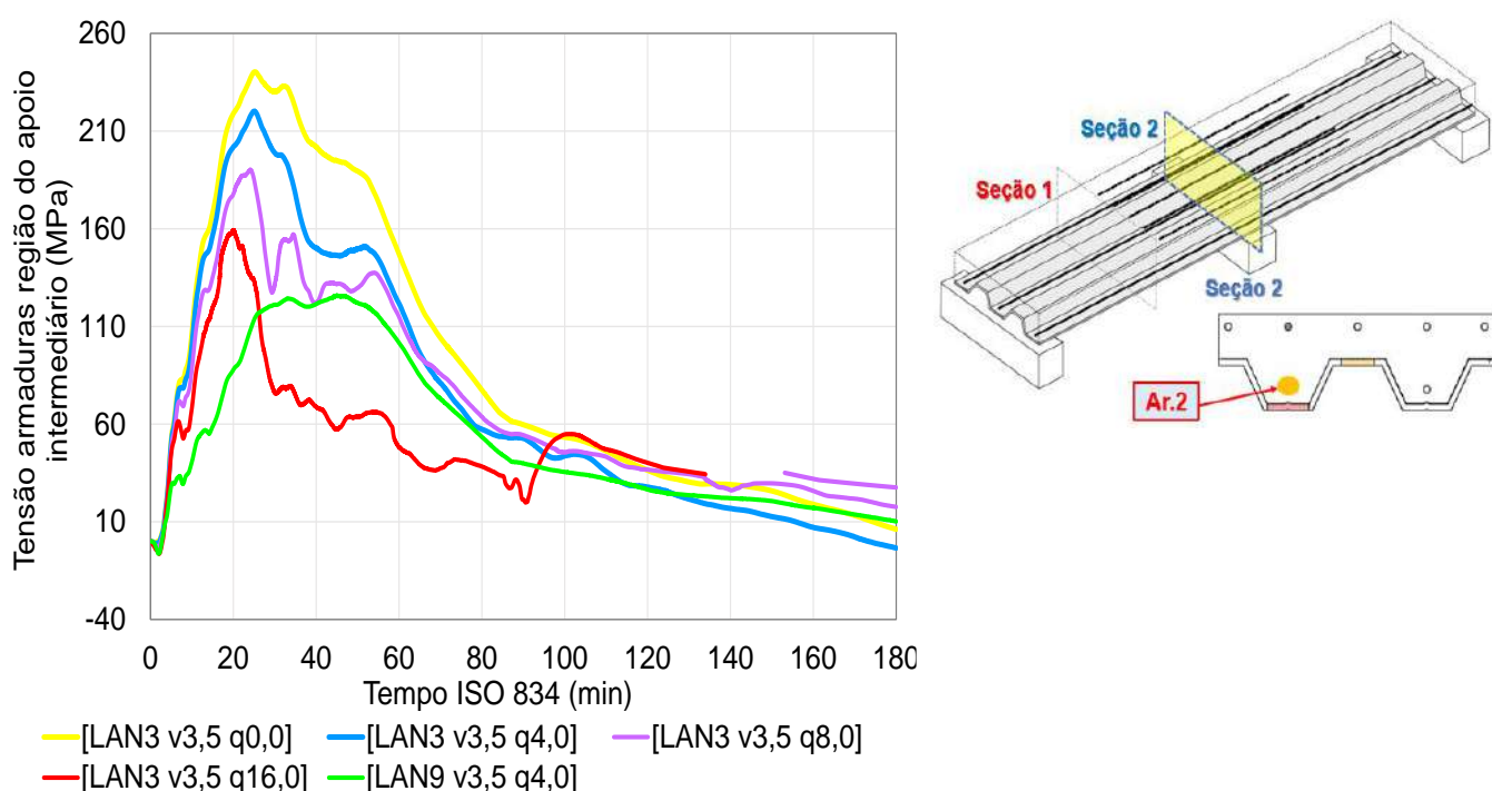
Figura 184 – Tensões produzidas nas armaduras positivas (Ar.2): vão de 3,5 m
