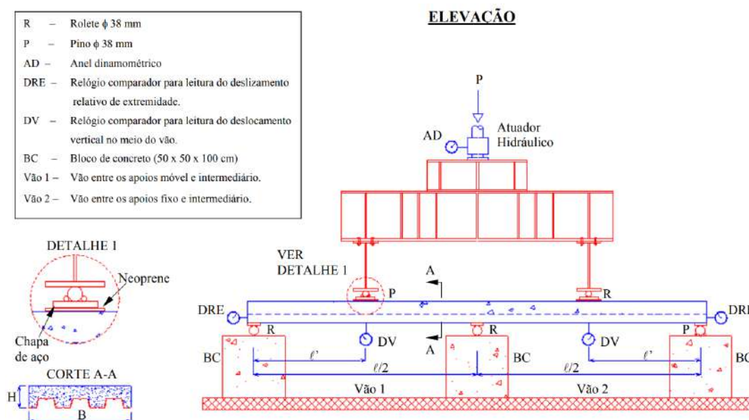
Figura 19 – Estudo do efeito de continuidade em lajes mistas com 2 vãos de 1,8 m Fonte: Campos (2001)
