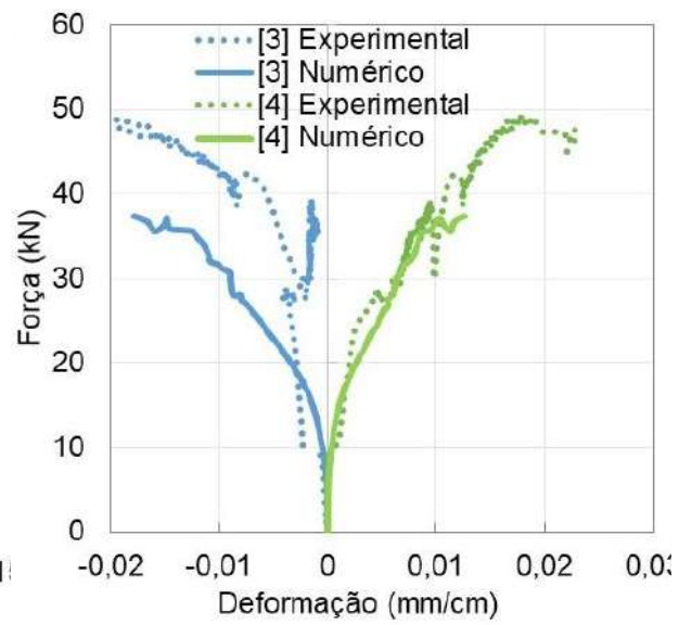
(e) LA5 e 6
