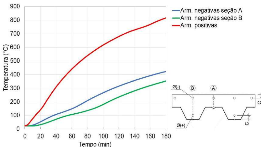
Figura 84 – Temperatura nas armaduras positivas e negativas
