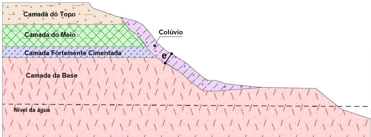
Figura 4.7 – Exemplo do perfil da Ponta do Pirambu com camada de colúvio
