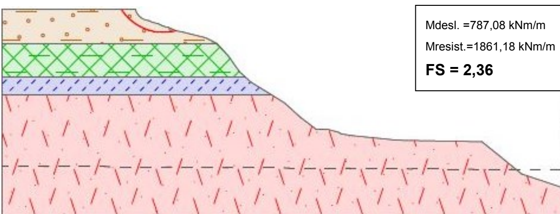
Figura 5.22 - Situação S6 da falésia da Ponta do Pirambu - após deslizamento de S5
