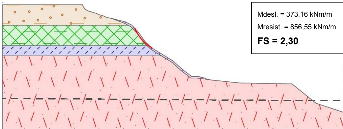
Figura 5.23 - Situação S6A0.5M da falésia da Ponta do Pirambu - com colúvio de 50cm
