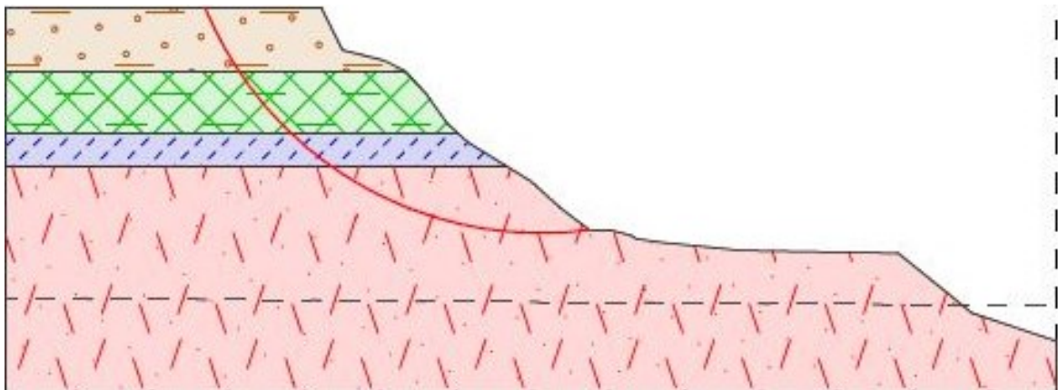
Figura 5.30 - Situação S1 com superfície de ruptura global gerada pela análise otimizada e repetida para as demais seções
