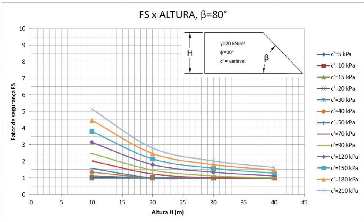
Figura 5.8 - Gráfico FS x H, para \beta = 80^\circ
