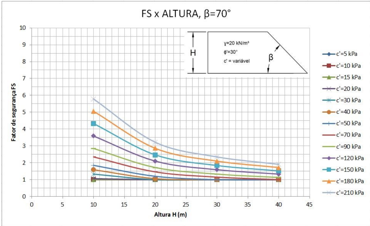
Figura 5.7 - Gráfico FS x H, para \beta = 70^\circ
