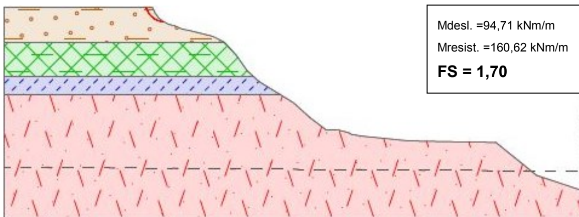
Figura 5.20 - Situação S4 da falésia da Ponta do Pirambu - após deslizamento de S3
