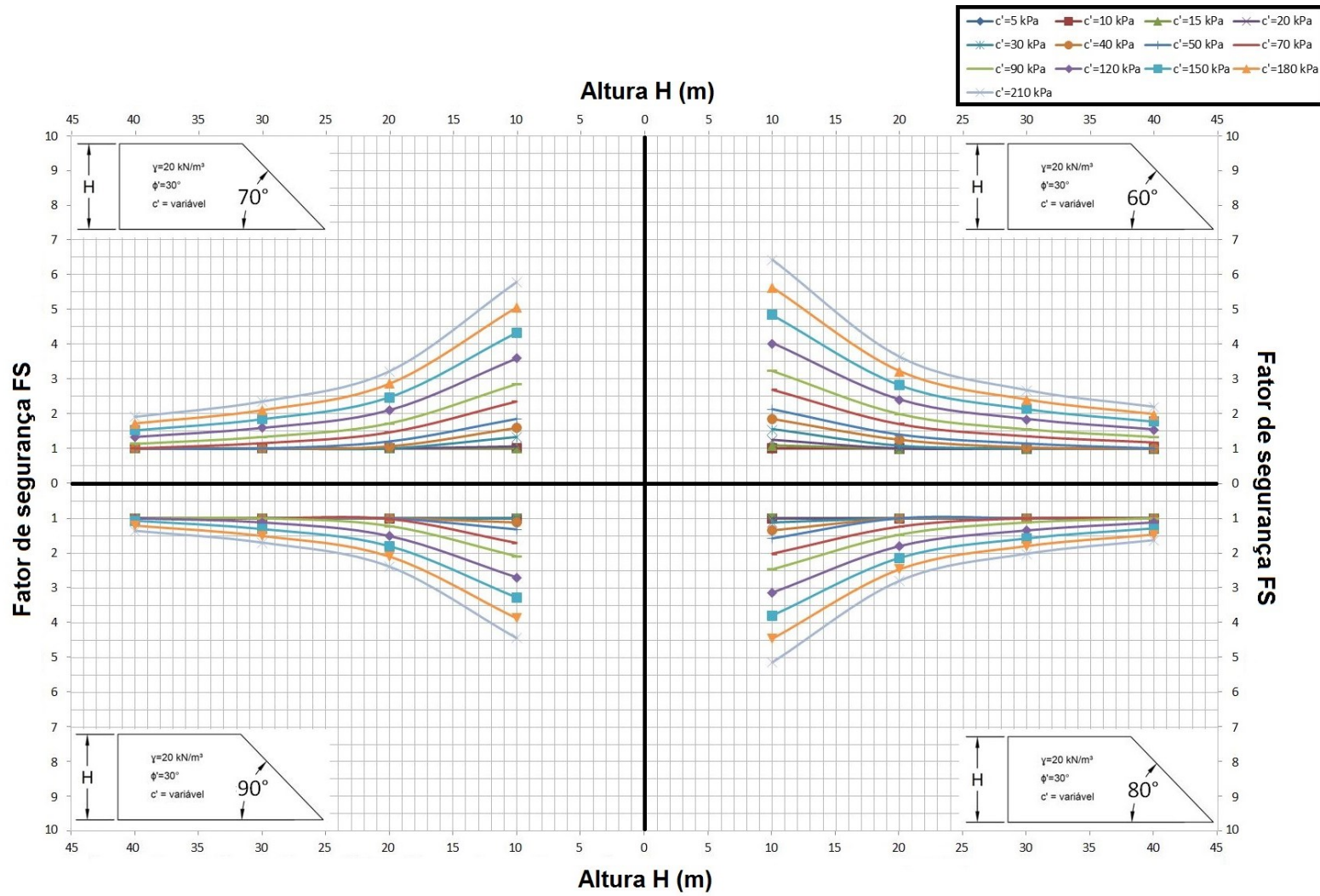
Figura 5.11 - Ábaco gerado a partir dos Gráficos FS x H, com \beta=60^\circ a 90^\circ
