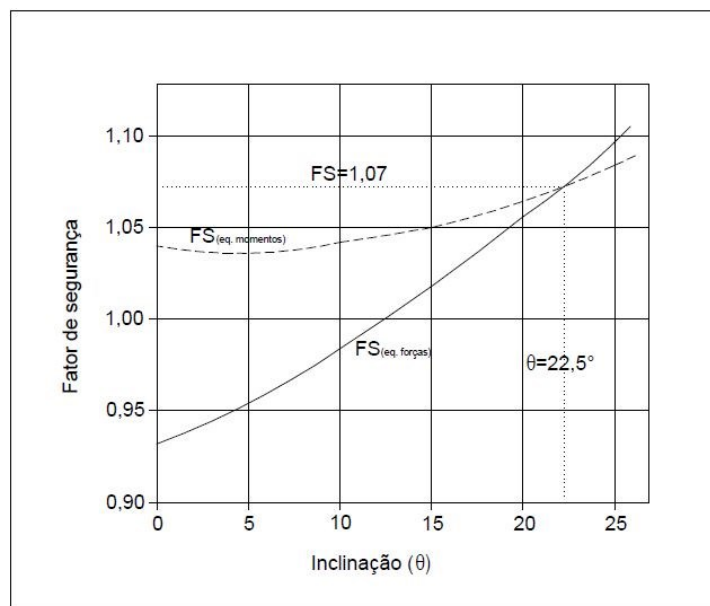
Figura 2.20 - Convergência do Método de Spencer.
