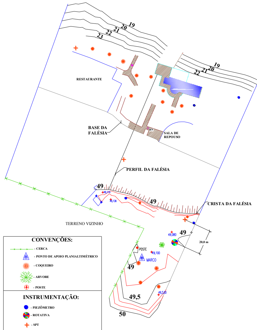
Figura 3.10 – Planta de levantamento topográfico (Severo, 2011)
