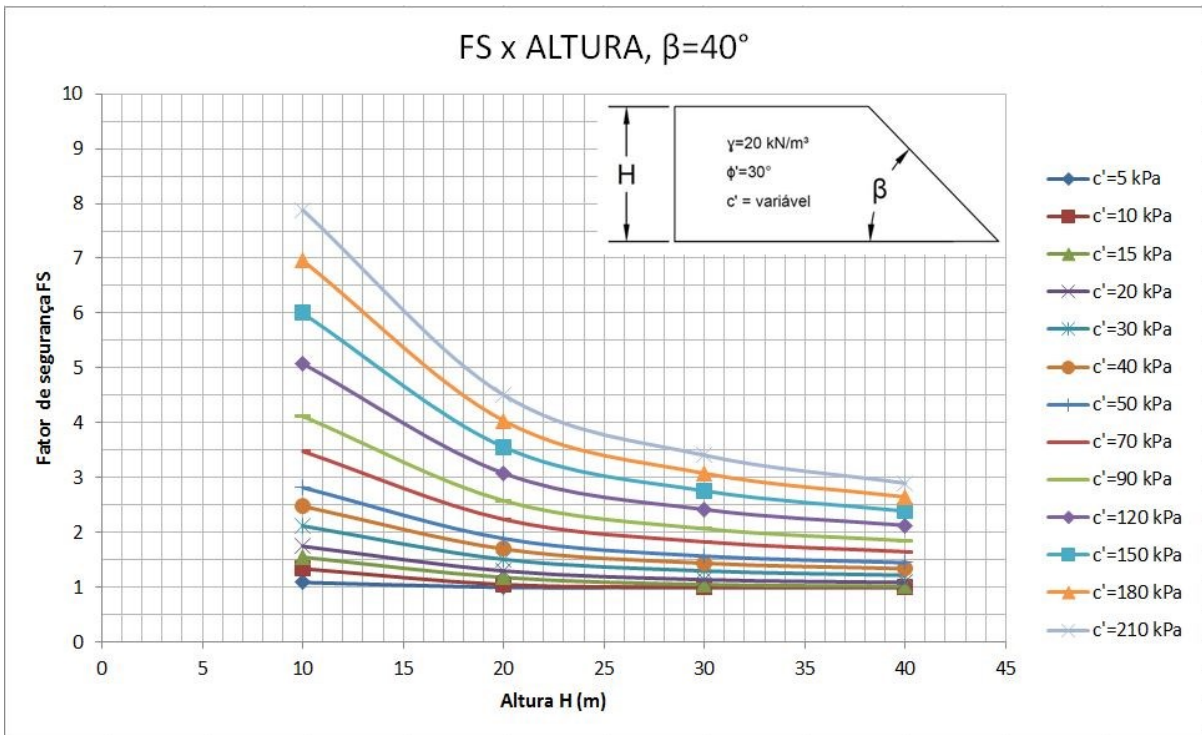
Figura 5.4 - Gráfico FS x H, para \beta = 40^\circ
