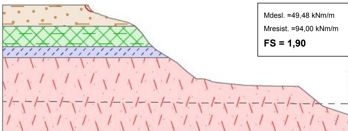
Figura 5.21 - Situação S5 da falésia da Ponta do Pirambu - após deslizamento de S4
