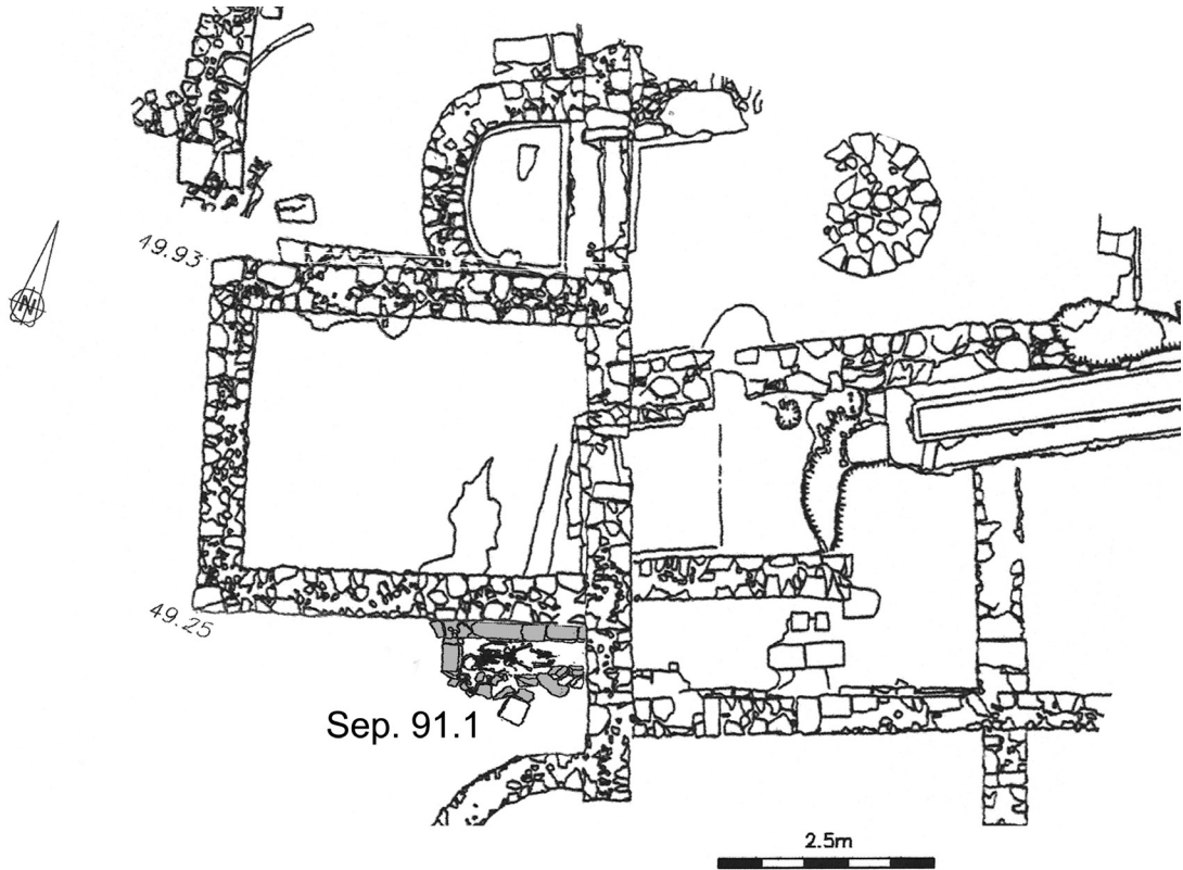
Fig. 12 – Planta das termas sul com a localização da sepultura 91.1.no seu interior.
