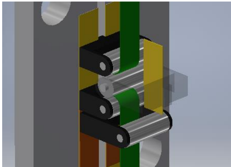
Figura 2.6 - Verificação do valor de penetração total, com auxílio de uma chapa plana. O elemento de suporte do rolo de conformação posicionado na placa superior for eliminado de modo a facilitar a visualização.
