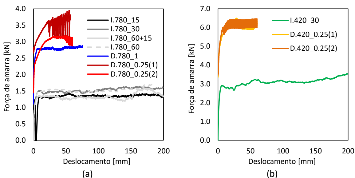
Figura 3.3 – Evolução da força da amarra com o deslocamento para os ensaios realizados no DEM e no IDMEC: (a) DP780; (b) HSLA420.
