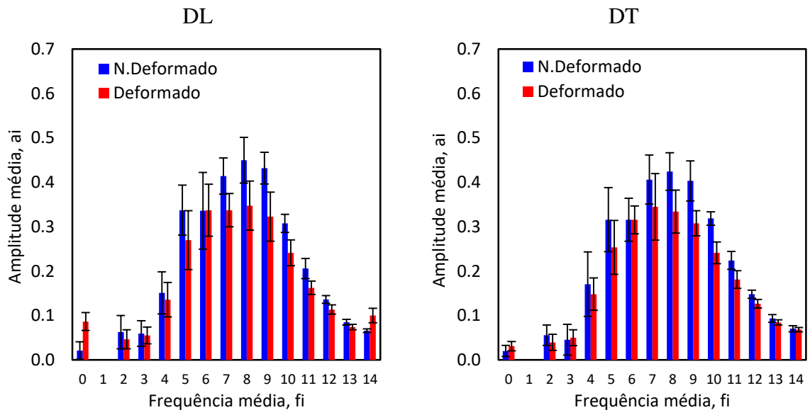
Figura A. 10 – Análise espectral em bandas de dois terços de oitava para o ensaio D.420_0.25(2).
