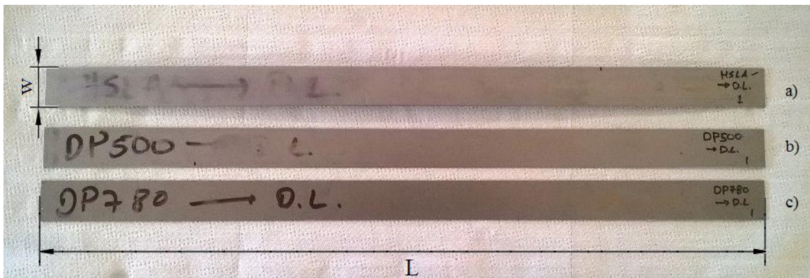
Figura 2.3 - Provetes de ensaio de atrito com freio: a) HSLA420 b) DP500 c) DP780.
