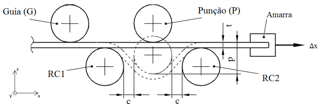
Figura 1.4 - Representação esquemática do ensaio de atrito com freio: posição inicial a traço contínuo e posição estacionária a traço interrompido.
