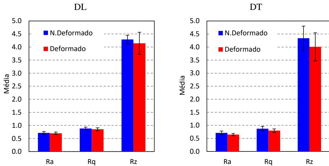
Figura A. 1 – Parâmetros de rugosidade determinados para o ensaio I.780_60+15.
