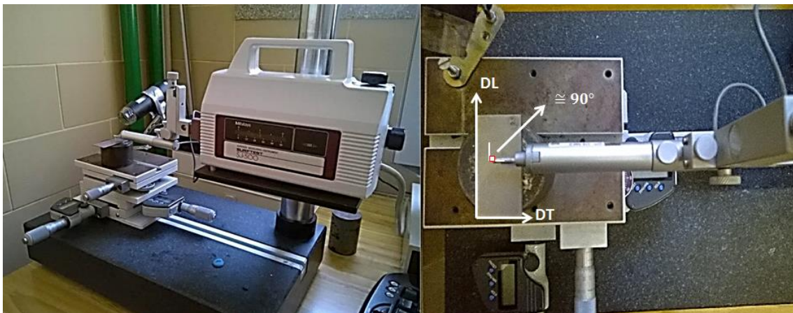
Figura 2.10 – À esquerda: Perfilómetro Mitutoyo SurfTest SJ-500 e à direita: posicionamento da amostra.
