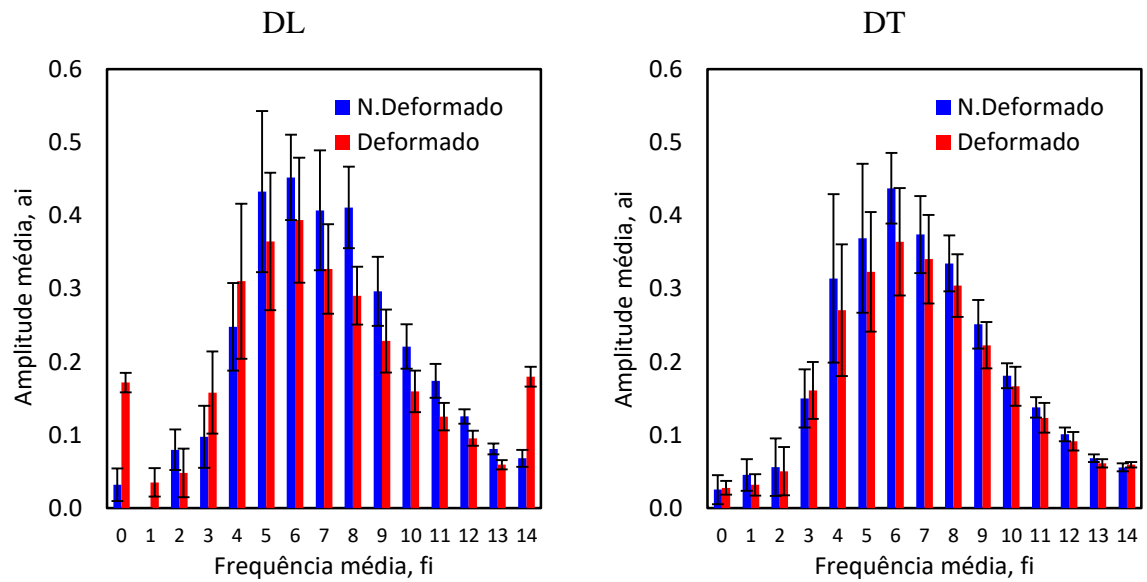
Figura A. 9 – Análise espectral em bandas de dois terços de oitava para o ensaio D.780_5.
