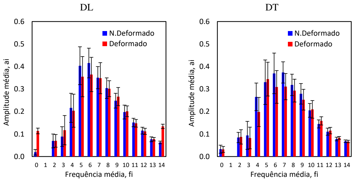
Figura A. 6 – Análise espectral em bandas de dois terços de oitava para o ensaio I.780_60+15.
