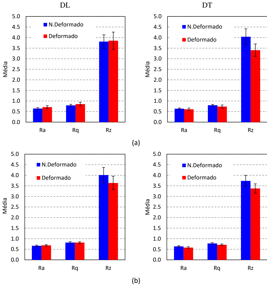
Figura 3.9 – Parâmetros de rugosidade determinados para os ensaios realizados no IDMEC: (a) ensaio I.780_15 e (b) ensaio I.780_30.
