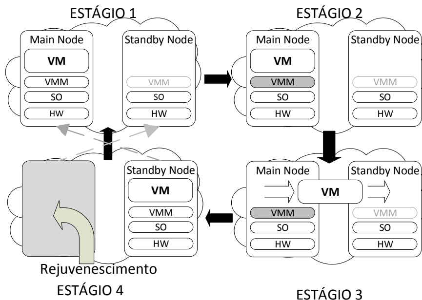
Figura 3.5: Estratégia adotada para o rejuvenescimento
