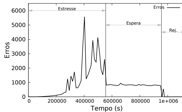
(f) Erros
