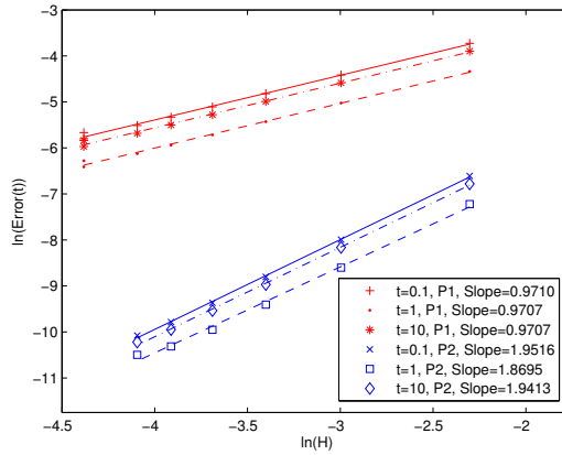
Figure 2: \ln(\|c(t) - c_H(t)\|_{H^1(\Omega)}) versus \ln(H) .
