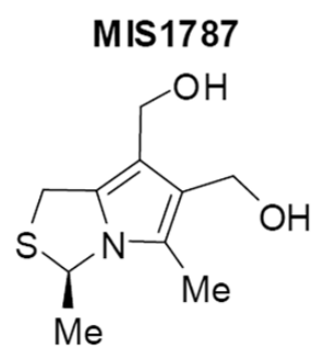
Figura 10 - Estrutura química dos compostos ASRO-13, ASRO-15, ASRO-17, MIS1707, MIS1786 e MIS1787. A Figura 10 também se encontra na página 57.
