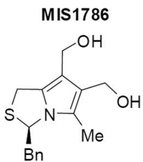
Figura 10 - Estrutura química dos compostos ASRO-13, ASRO-15, ASRO-17, MIS1707, MIS1786 e MIS1787. A Figura 10 também se encontra na página 57.
