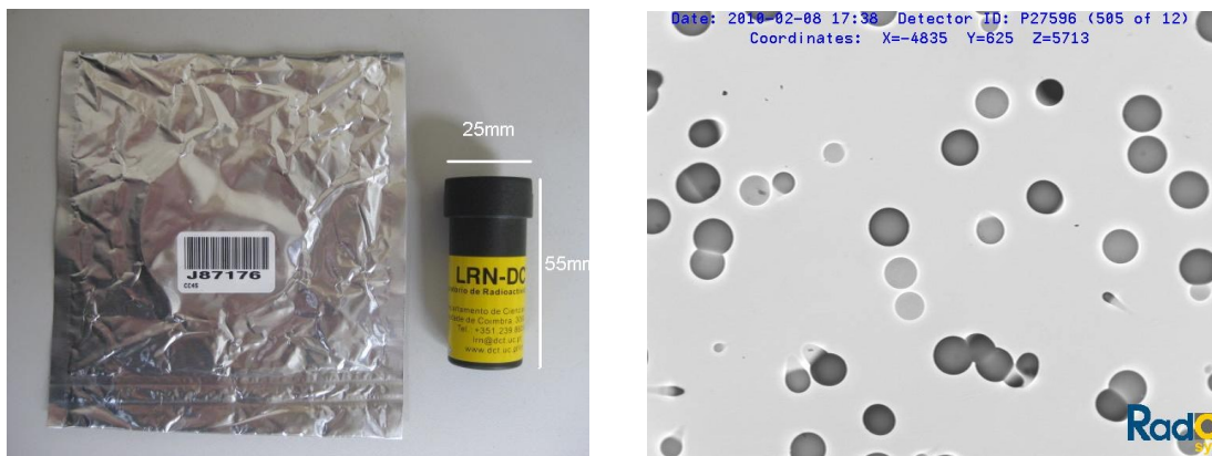
Figura 3.13 - Detector passivo do tipo CR39 em invólucro plástico anti-electrostático e respectiva embalagem de folha de alumínio (à esquerda), e aspecto dos impactos das partículas alfa no detector CR39 em observação ao microscópio após tratamento químico (à direita).
