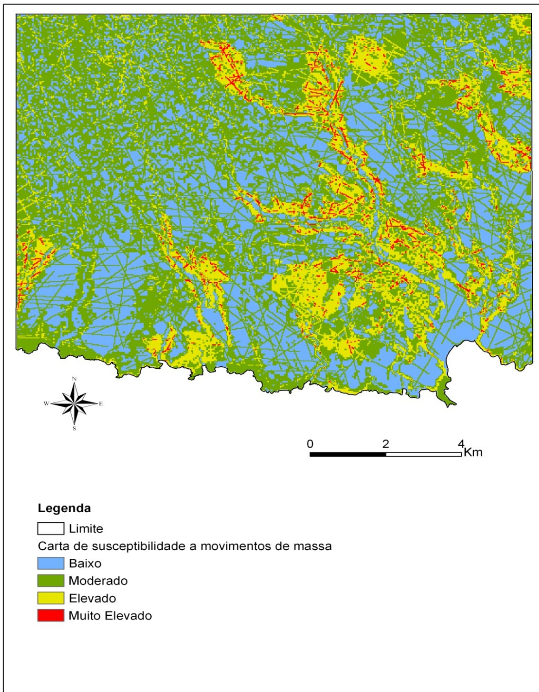
Figura 1.7 - Carta de susceptibilidade a movimentos de massa (Victória, 2006).
