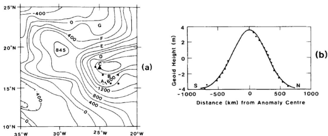
Figura 1.3 - a) Mapa de anomalias de profundidade em relação ao fundo oceânico não perturbado (em metros), com as estações de fluxo sobrepostas. b) Altura do geóide ao longo de uma linha centrada em 25° W. O triângulo marca o centro da anomalia. Retirado de Courtney & White (1986).
