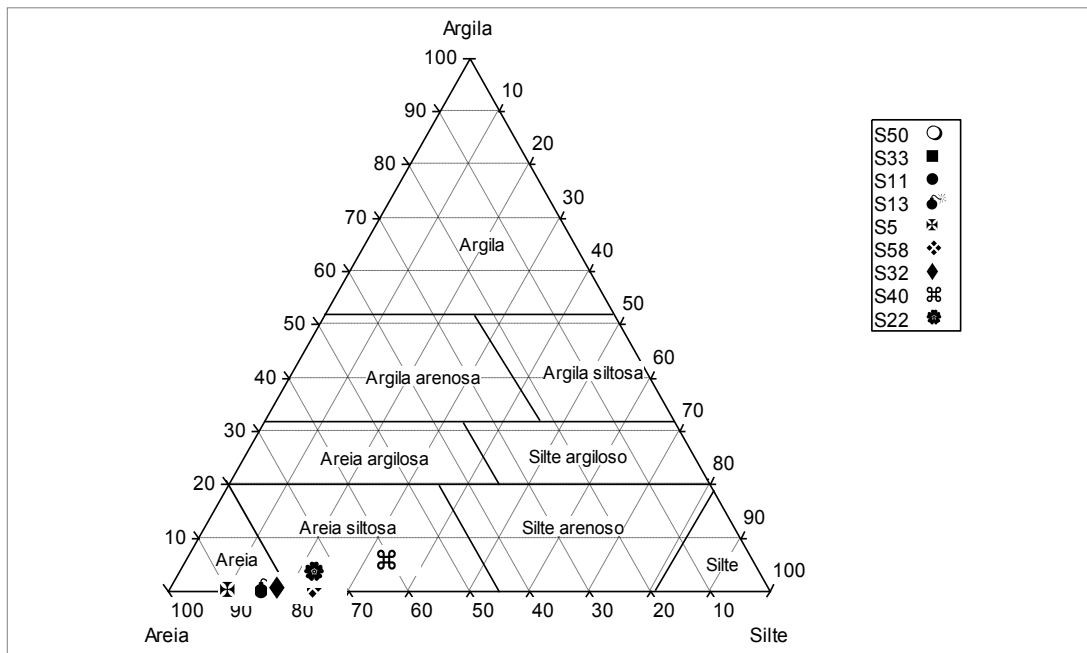
Figura 5.11 - Classificação textural – Brechas hialoclastíficas.
