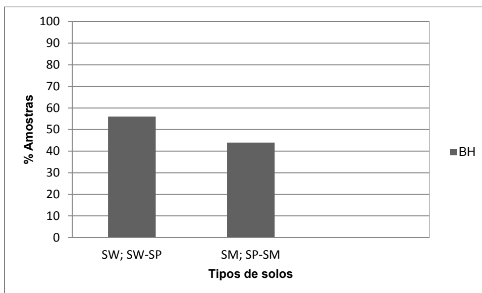
Figura 5.12 - % Amostras vs tipos de solos –Brechas hialoclastíficas.
