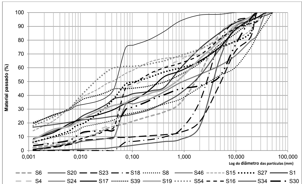
Figura 5.20 - Curvas granulométricas – Solos de cobertura
