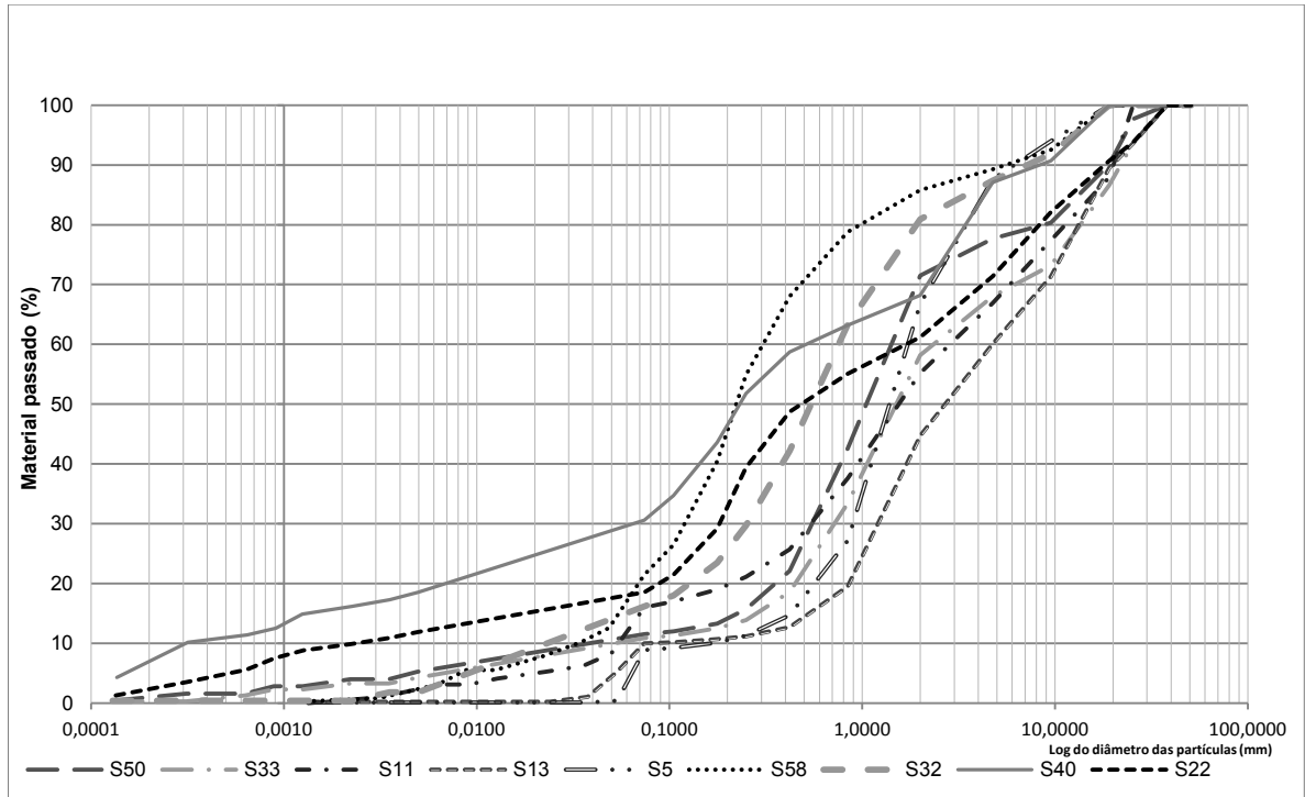
Figura 5.10 - Curvas granulométricas – Brechas hialoclastíficas.
