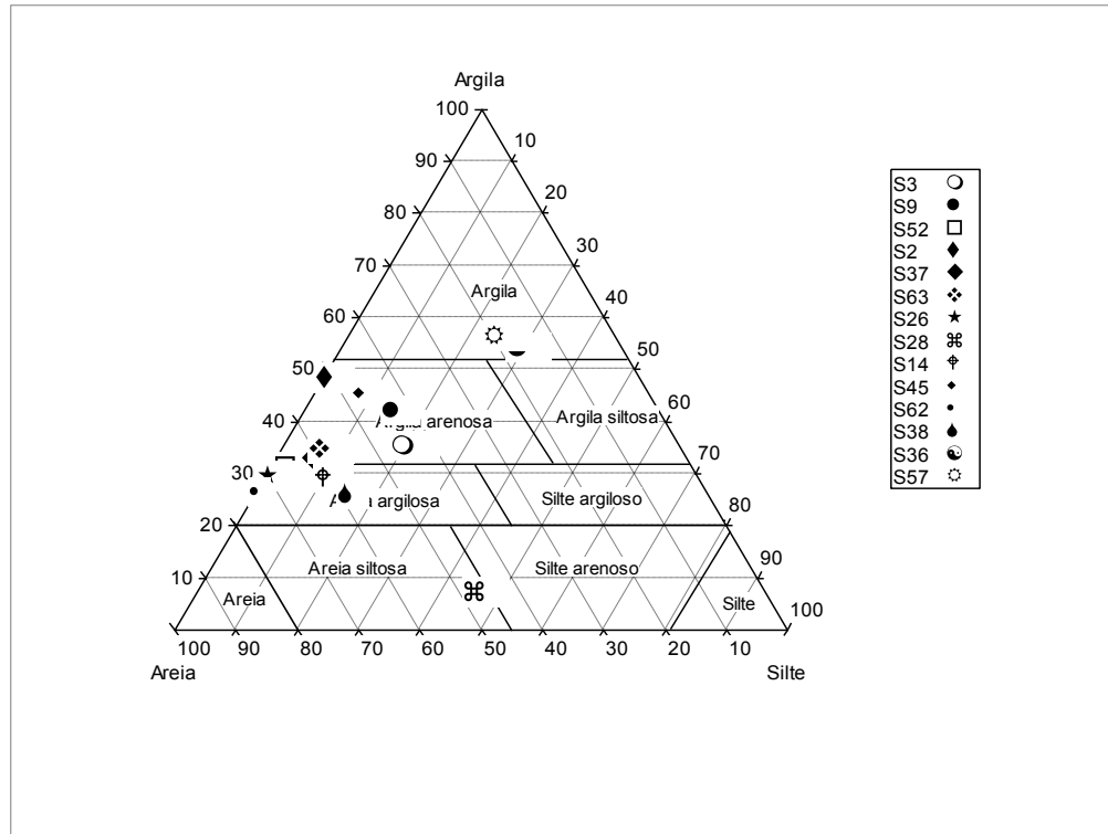
Figura 5.5 - Classificação textural – Mantos e filões básicos e ultra-básicos.
