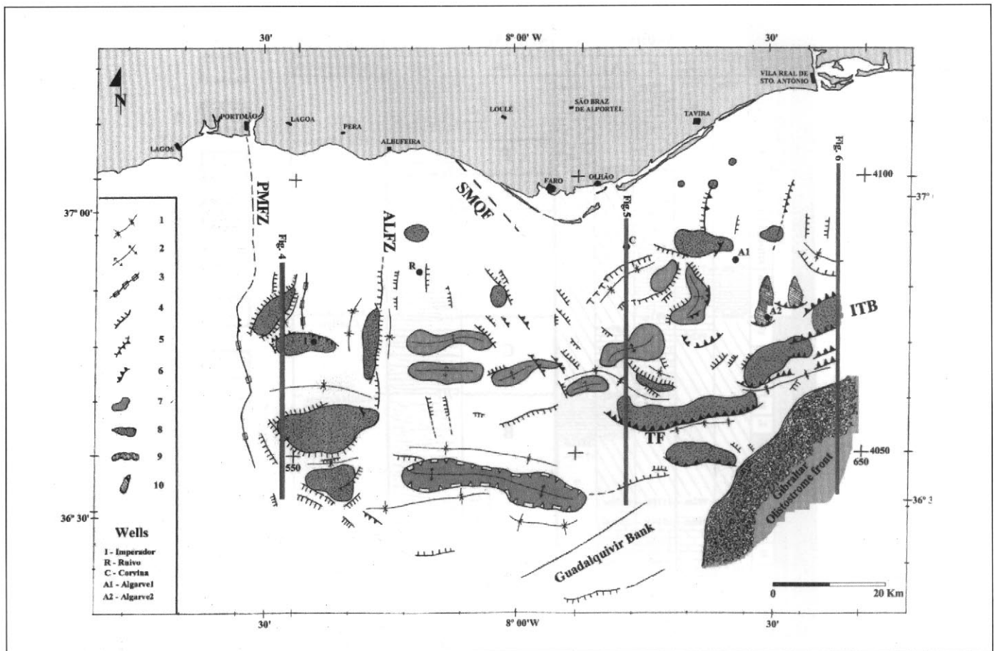
Fig. 3. Map of the main cenozoic structures. PMFZ: Portimão-Monchique Fault Zone; ALFZ: Albufeira Fault Zone; SMQF: São Marcos-Quarteira Fault Zone; TF: thrust front; ITB: imbricated thrust belt. 1: syncline axis; 2: anticline axis; 3: strike-slip fault; 4: normal fault; 5: reversal normal fault; 6: thrust fault; 7: structural high; 8: evaporitic structure; 9: reversal half-graben; 10: ramp anticline Fig. 3. Mapa de las principales estructuras cenozoicas. PMFZ: Zona de Falla de Portimão-Monchique; ALFZ: Zona de Falla de Albufeira; SMQF: Zona de Falla de São Marcos-Quarteira; TF: frente de cabalgamiento; 7: alto estructural; 8: estructura evaporítica; 9: semi-fosa inversa; 10: rampa anticlinal
