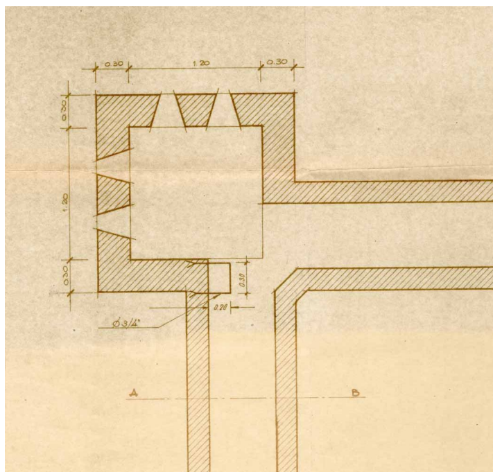
Pormenor da planta de fortificação do campo de trabalho de Chão Bom, da autoria do Comando Territorial Independente de Cabo Verde, 1967.
