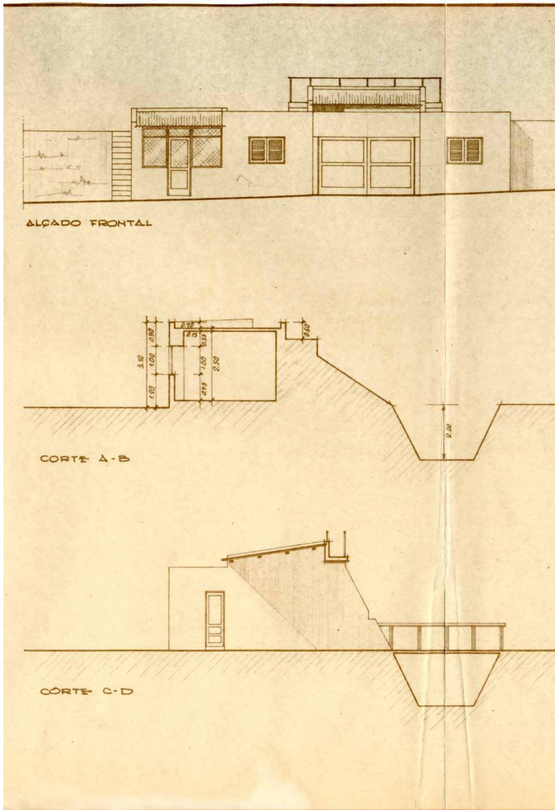
Alçado frontal e cortes do projecto de fortificação do campo de trabalho
