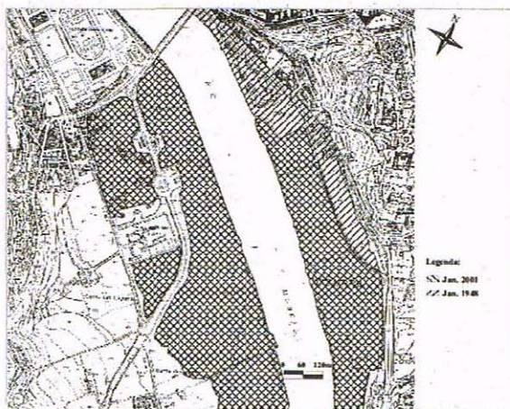
Figura 8 - Representação das áreas de “restrição” (Janeiro de 2001) e de “precaução” (Janeiro de 1948) com base nas maiores inundações em Coimbra (Secção de referência: Ponte de Sta Clara – Coimbra), com caudal natural (1948) e com caudal regularizado (2001).
