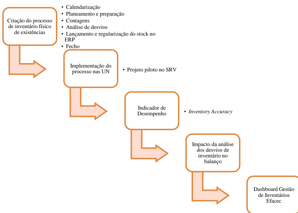
Figura 5. Metodologia aplicada
